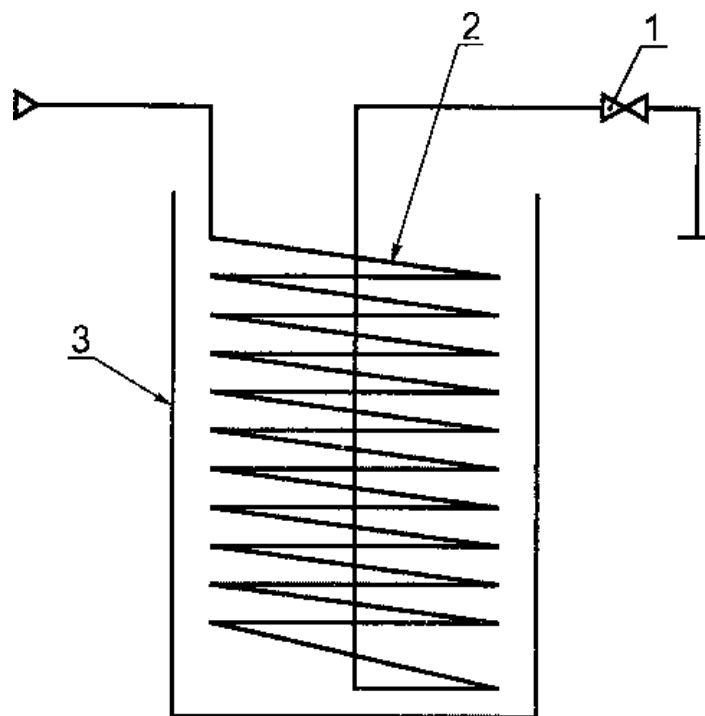
1 - игольчатый вентиль; 2 - змеевик; 3 - сосуд для охлаждающей смеси Рисунок 1. Устройство для охлаждения сжиженного газа
