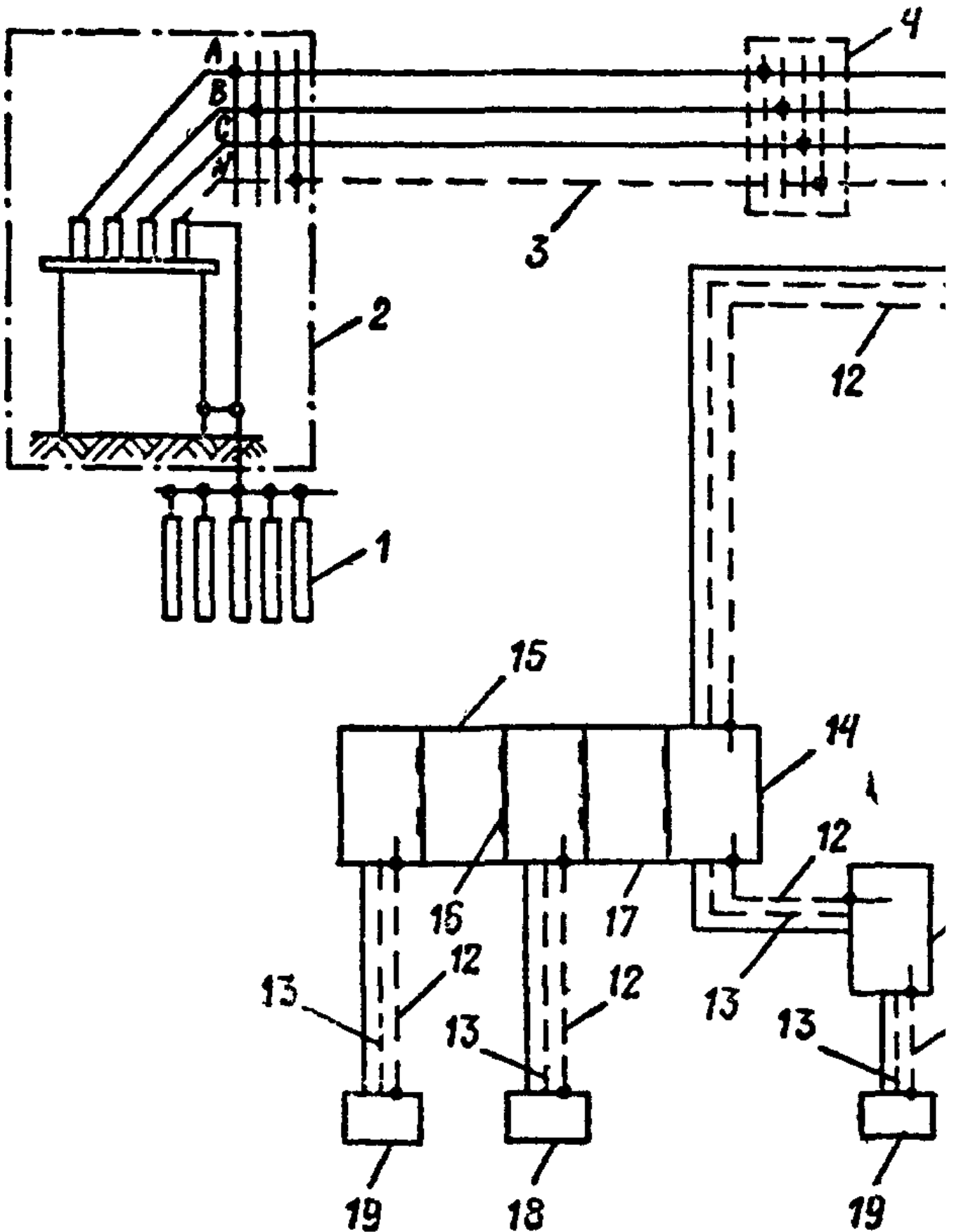
Рис. 3. Пример выполнения зануления в электроустановке системы автоматизации: 1 - заземлитель; 2 - понижающая трансформаторная подстанция автоматизируемого объекта; 3 - нулевой рабочий проводник, используемый в качестве магистрали зануления; 4 - промежуточный щит электроснабжения; 5 - распределительный щит электроснабжения, питающий систему автоматизации; 6 - нулевой рабочий проводник, который используется в качестве нулевого защитного проводника, зануляющего сборку питания задвижек, пускатель, электропривод; 7 - сборка питания задвижек; 8 - повторное зануление; 9 - электропривод задвижки; 10 - магнитный пускатель; 11 - местный щит контроля и управления; 12 - нулевой защитный проводник; 13 - нулевой рабочий проводник; 14 - панель питания системы автоматизации; 15 - щит контроля и управления в
