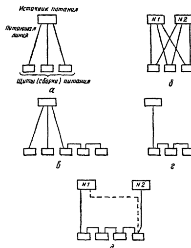
Рис. 2. Схема питающей сети системы электропитания: а - радиальная с односторонним питанием; б - радиальная с двухсторонним питанием; в - радиально-магистральная (смешанная); г - магистральная с односторонним питанием; д - магистральная с двухсторонним питанием от одного источника (линия от источника питания N 2 отсутствует) и от двух источников (пунктирная линия исключается)
