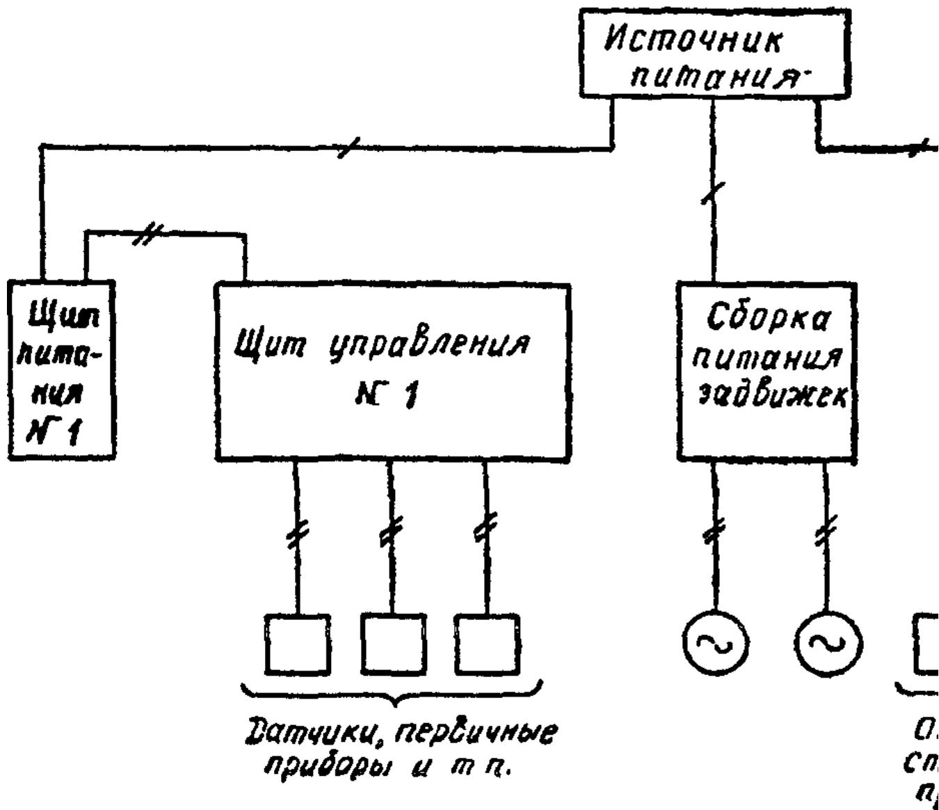
Рис. 1. Основные звенья схемы электропитания систем автоматизации (линия с одним штрихом - питающая сеть, с двумя штрихами - распределительная сеть)
