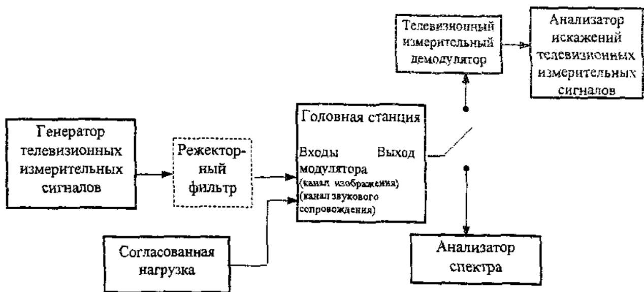
Рисунок 7.18. Структурная схема для определения отношения радиосигнала к одночастотной помехе комбинационных частот третьего порядка
