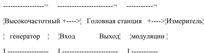
Рисунок 7.14. Структурная схема для определения отношения сигнала к фоновой помехе
