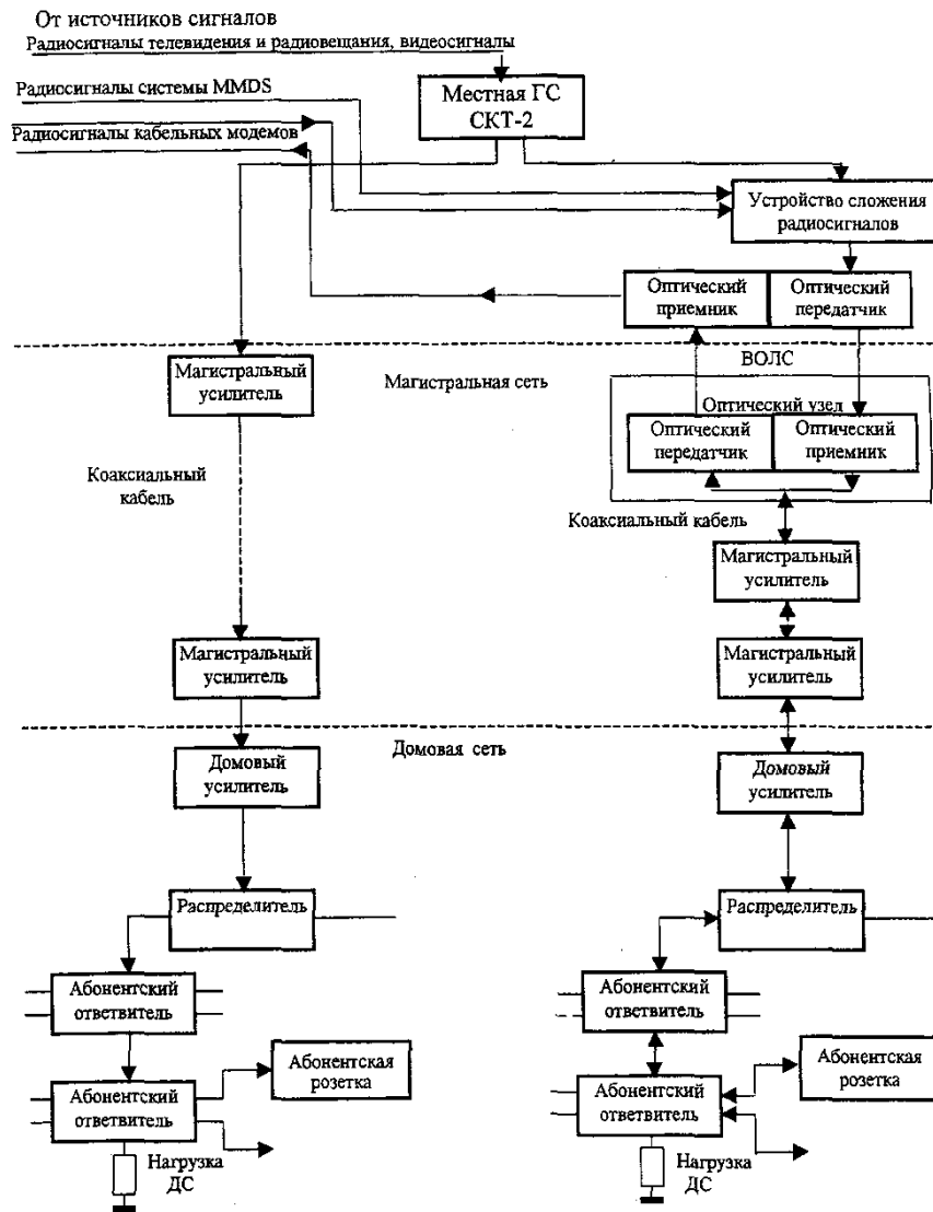
Рисунок 4.2. Структурные схемы районной кабельной распределительной сети SKT-2
