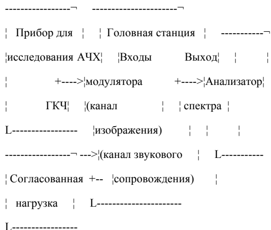
Рисунок 7.20. Структурная схема для определения характеристики боковых полос
