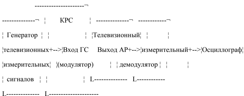
Рисунок 7.2. Структурная схема измерения импульсной характеристики канала распределения (К-фактора)
