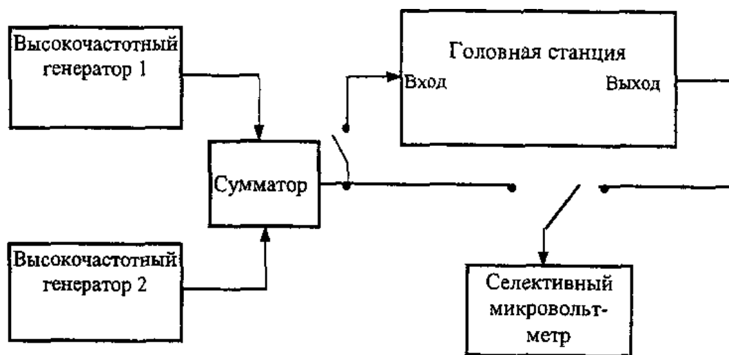
Рисунок 7.13. Структурная схема для определения отношения радиосигнала изображения к побочным помехам, неравномерности АЧХ в канале распределения и избирательности канального усилителя (конвертора) ГС
