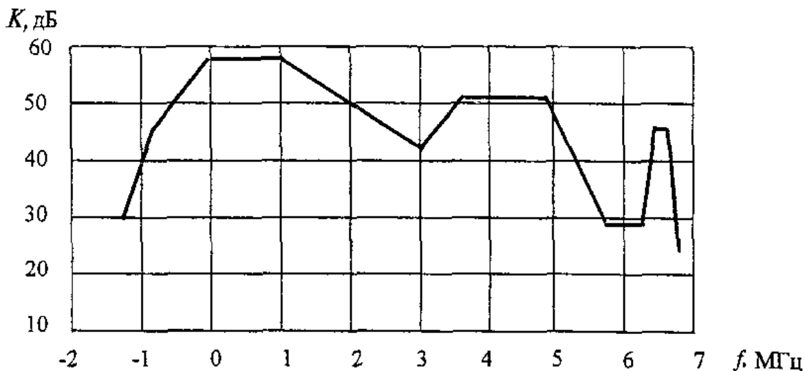
Рисунок 5.1. Кривая защитных отношений для системы вещательного телевидения
