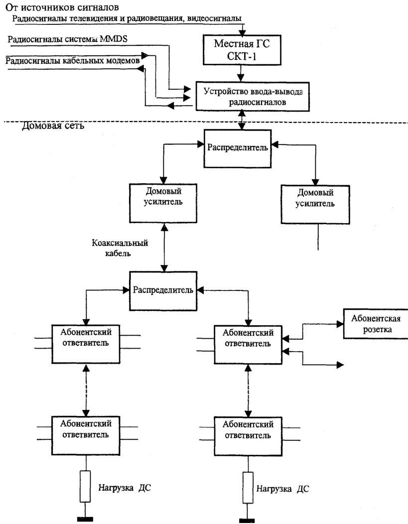
Рисунок 4.1. Структурная схема местной кабельной распределительной сети СКТ-1
