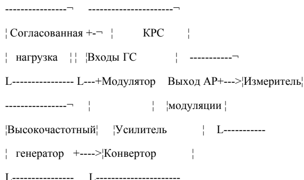
Рисунок 7.6. Структурная схема для определения отношения сигнала изображения к фоновой помехе
