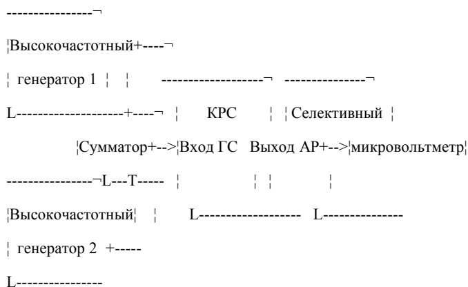
Рисунок 7.1. Структурная схема для определения неравномерности АЧХ в канале распределения радиосигнала вещательного телевидения
