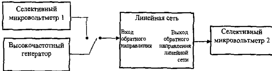
Рисунок 7.9. Структурная схема для определения уровня радиосигнала на входе обратного направления, наклона АЧХ в полосе частот обратного направления и отношения радиосигнала с цифровой модуляцией к одночастотной помехе в канале обратного направления
