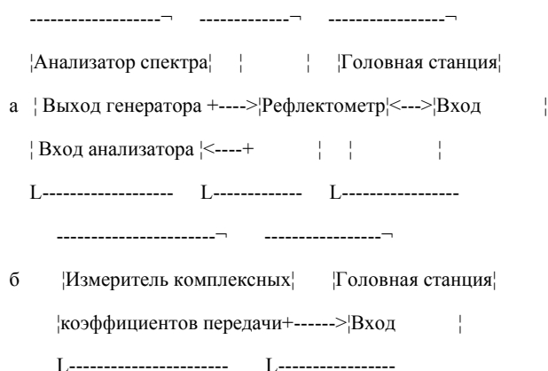
Рисунок 7.15. Структурная схема для измерения затухания несогласованности
