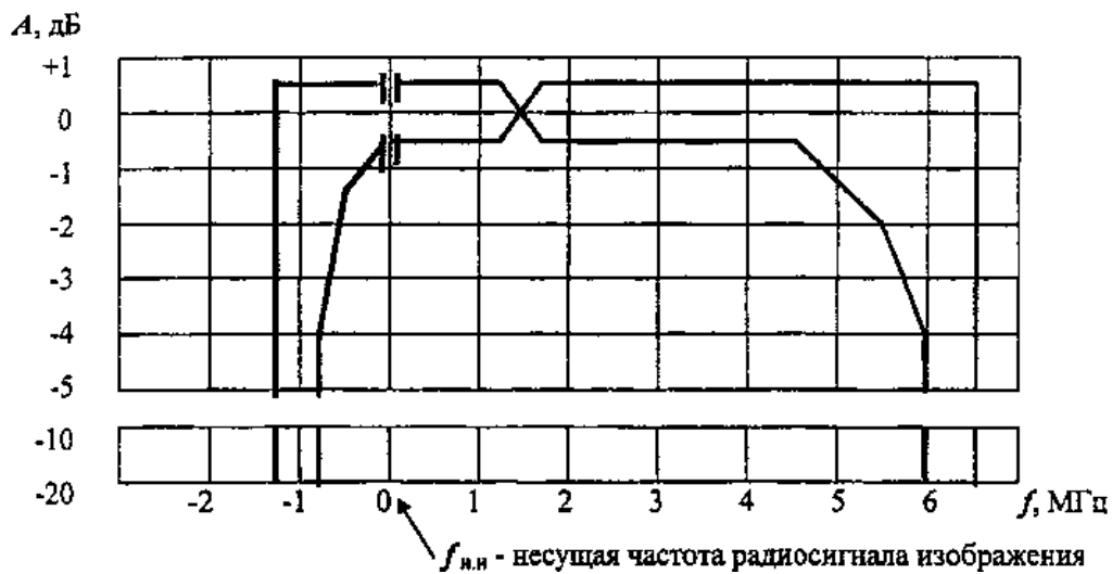
Рисунок Б.1. Поле допуска характеристики боковых полос в полосе частот от - 1,25 МГц до + 6,5 МГц
