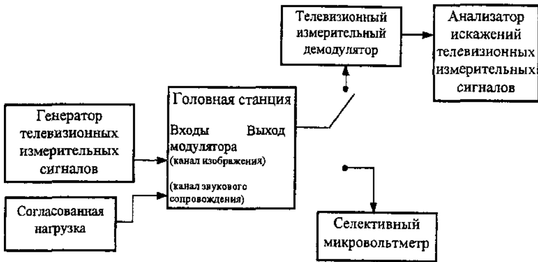
Рисунок 7.21. Структурная схема для определения отношения радиосигнала изображения к внеполосной помехе и измерения параметров канала изображения
