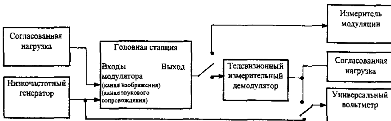
Рисунок 7.27. Структурная схема для определения отклонения АЧХ канала звукового сопровождения от характеристики идеальной цепи предискажений
