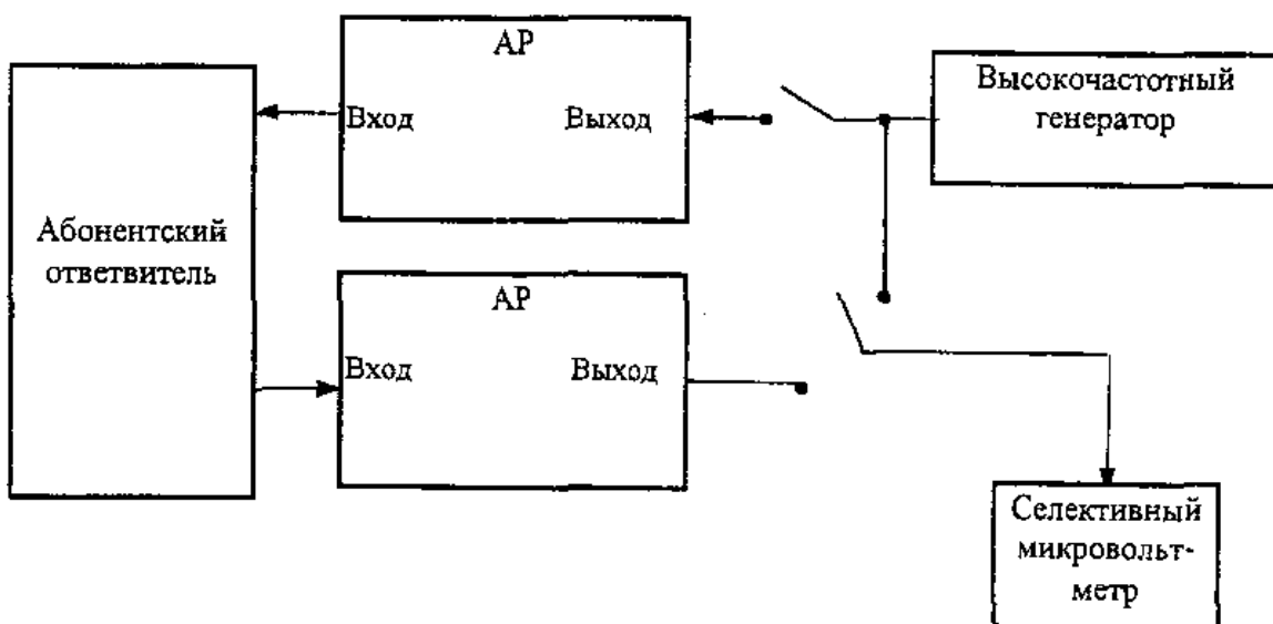
Рисунок 7.8. Структурная схема для определения переходного затухания между выходами абонентских розеток
