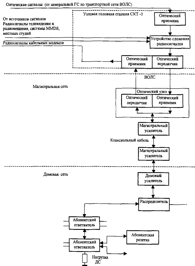
Рисунок 4.3. Структурная схема городской кабельной распределительной сети СКТ-3
