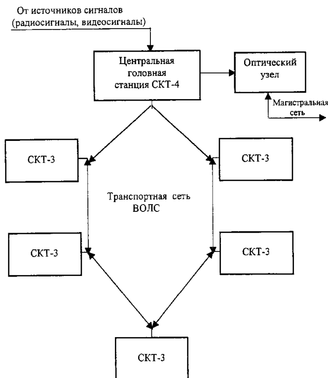
Рисунок 4.4. Структурная схема региональной кабельной распределительной сети СКТ-4
