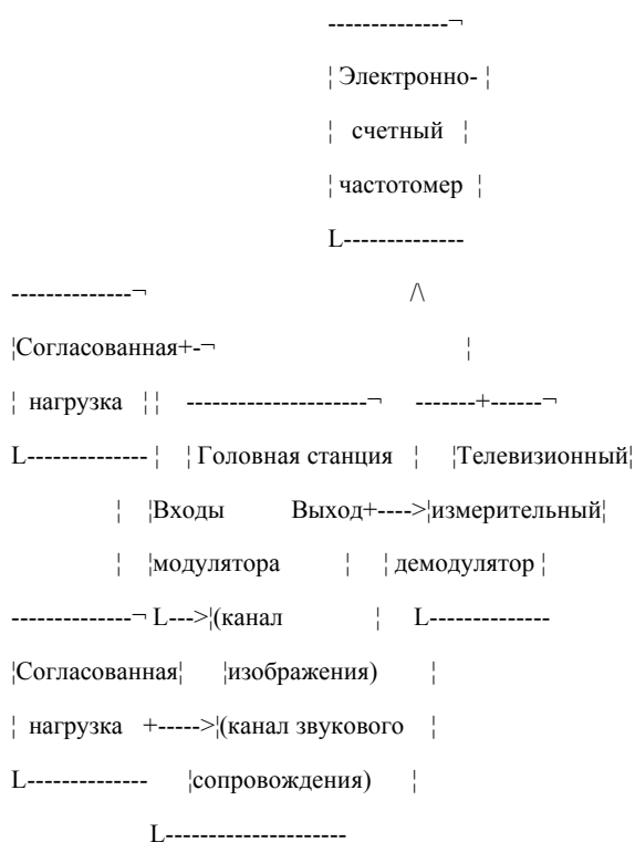
Рисунок 7.23. Структурная схема для определения отклонения разности несущих частот радиосигналов изображения и звукового сопровождения от номинального значения
