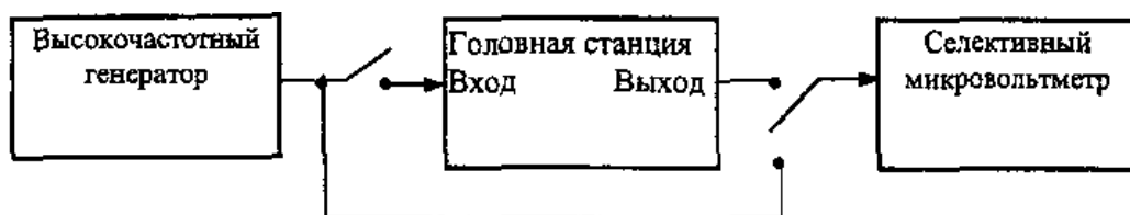
Рисунок 7.11. Структурная схема для определения диапазона входных уровней напряжения радиосигнала изображения, эффективности автоматической регулировки усиления, диапазона регулировки выходного уровня напряжения
