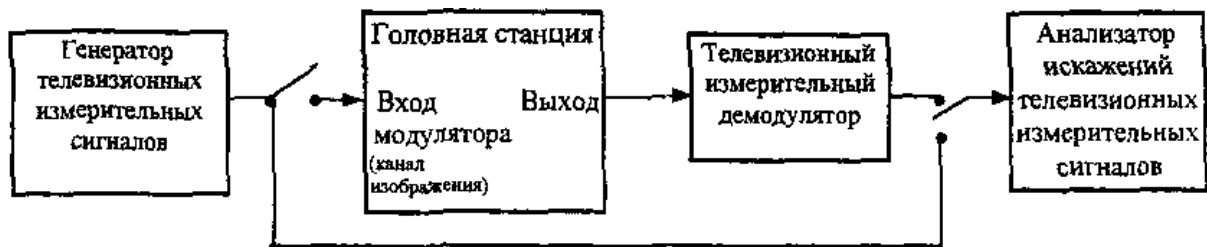
Рисунок 7.17. Структурная схема для измерения размаха полного цветного видеосигнала на входе телевизионного модулятора
