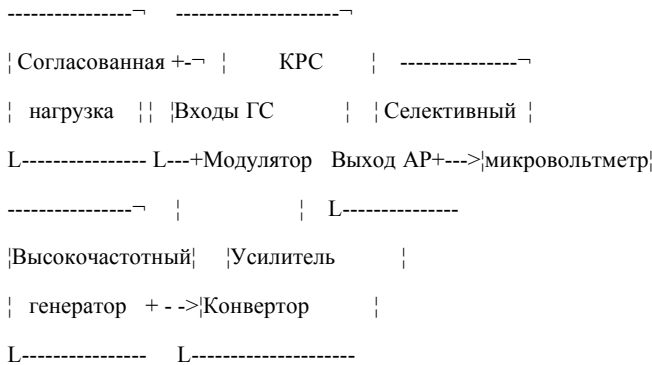
Рисунок 7.4. Структурная схема для определения отношения радиосигнала изображения к шуму
