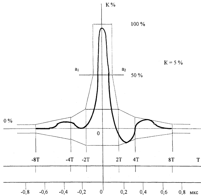
Рисунок 7.3. Оциллограмма 2Т-импульса измерительного сигнала N 2 (ГОСТ 18471)
