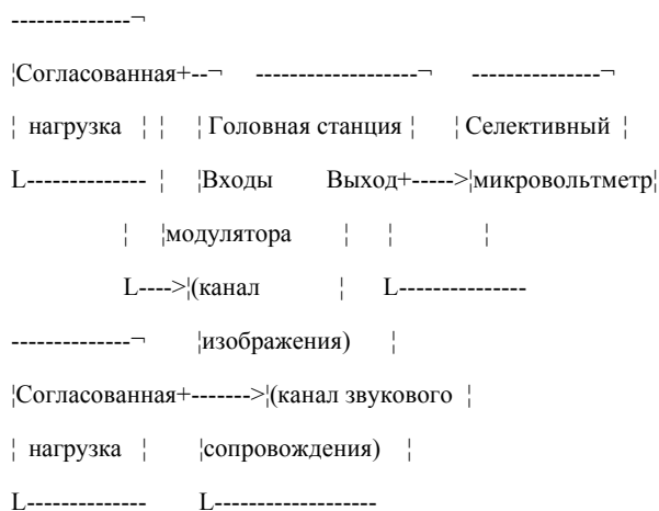
Рисунок 7.19. Структурная схема для определения отношения радиосигнала изображения к побочным помехам, разности уровней напряжения радиосигналов изображения и звукового сопровождения, отношения радиосигнала изображения к шуму в полосе частот канала изображения
