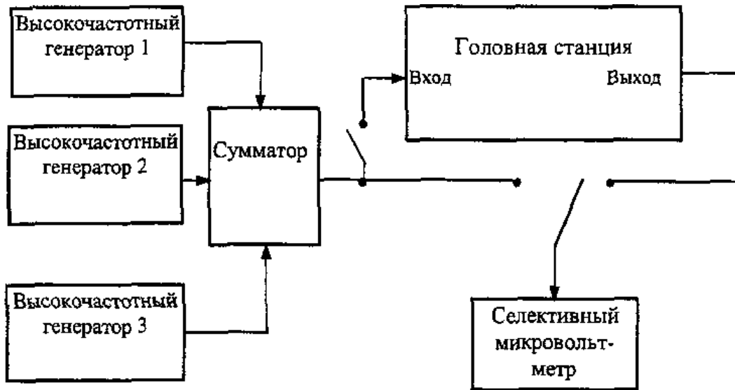
Рисунок 7.12. Структурная схема для определения отношения радиосигнала изображения к одночастотной помехе комбинационных частот третьего порядка
