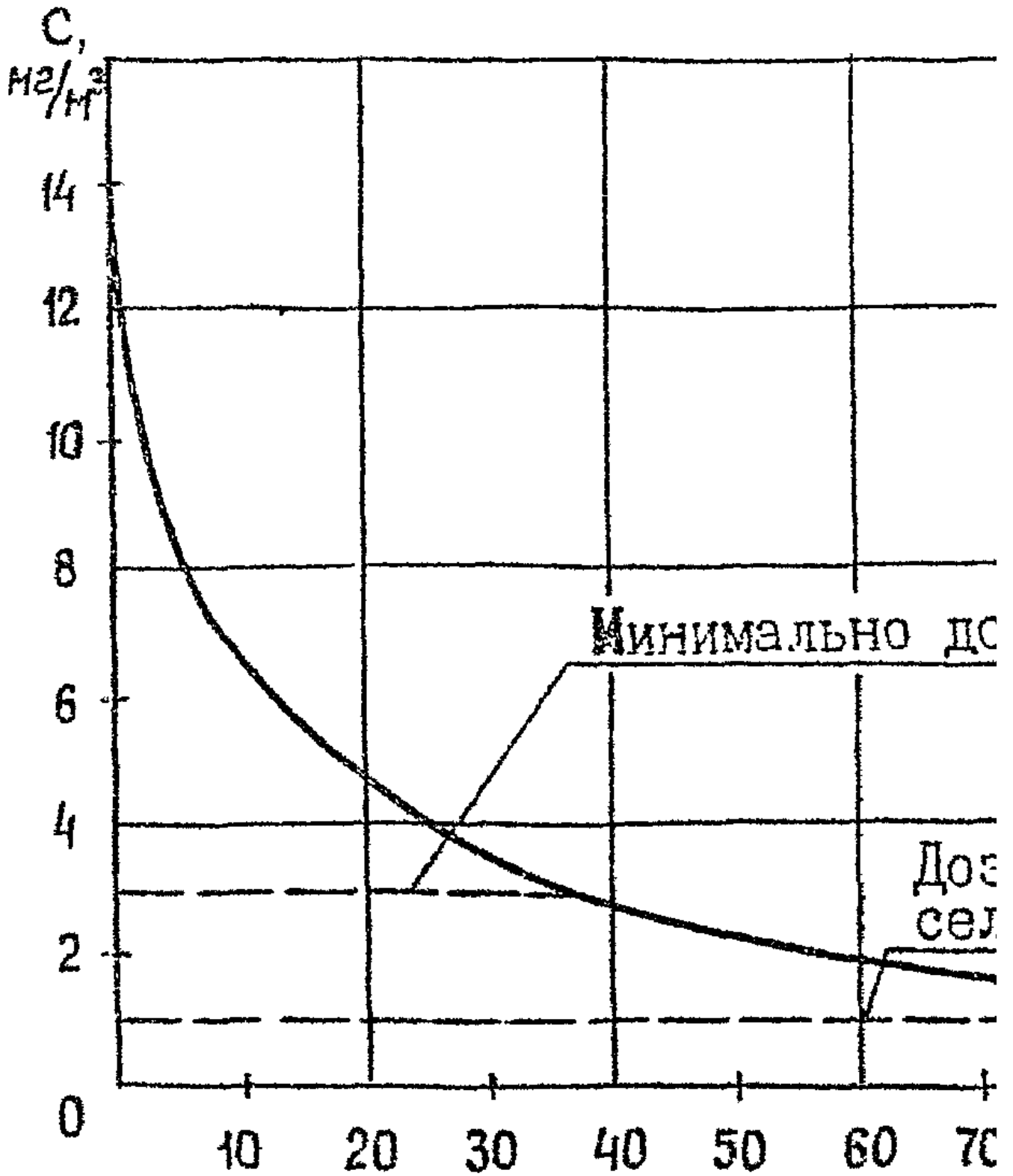
Рис. 1. Загазованность придорожной территории на автомобильной дороге I категории (N = 10000 авт./сут.) выбросами автотранспорта (окись углерода)
