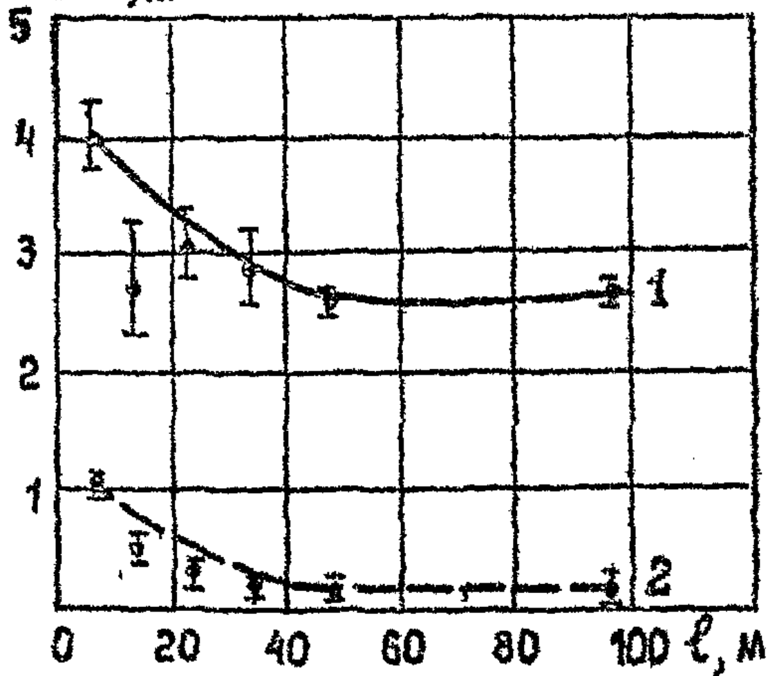
Рис. 6. Содержание меди (1) и кадмия (2) в напочвенном слое придорожной полосы в зависимости от расстояния от полотна дороги
