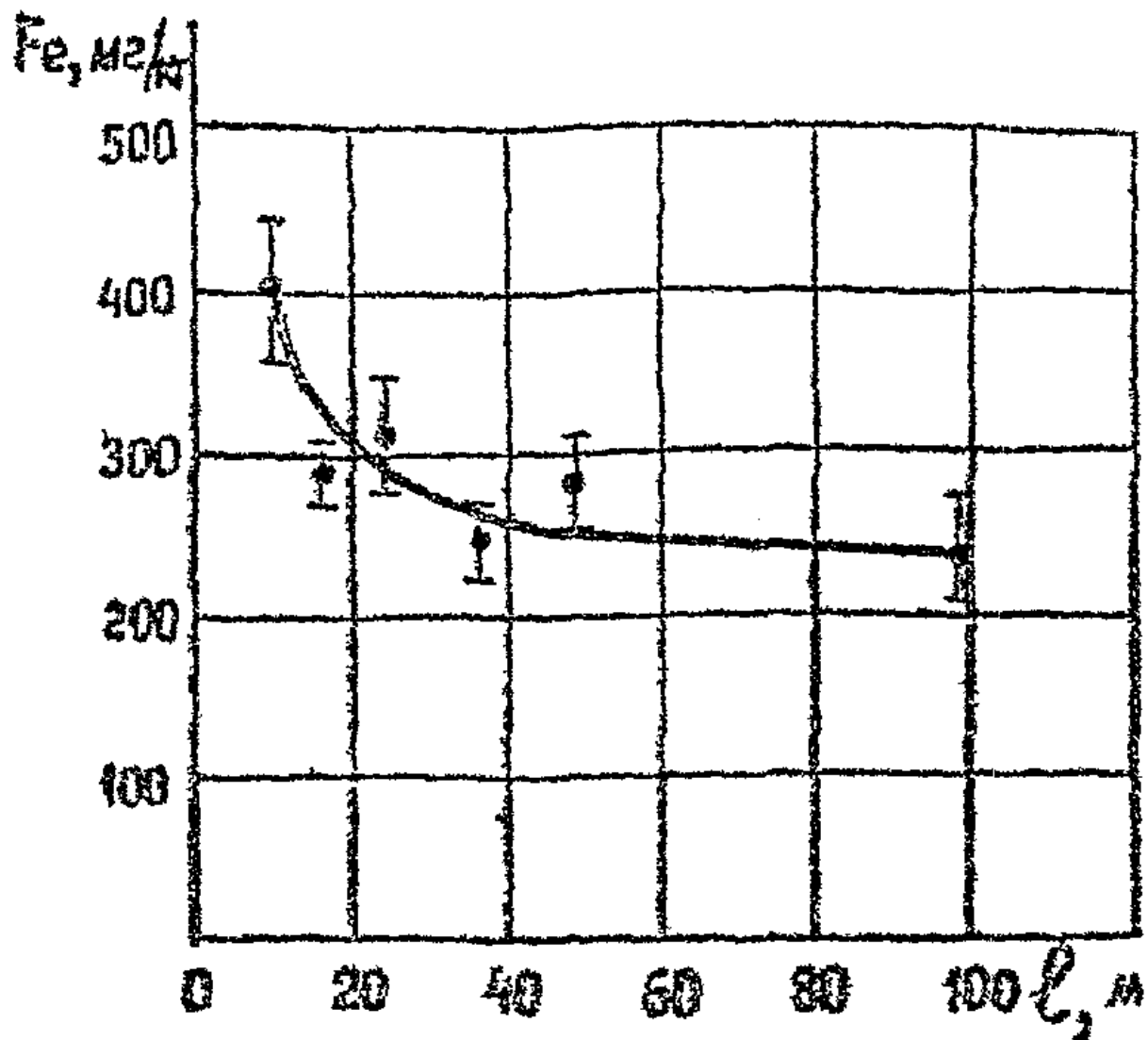
Рис. 5. Содержание железа в напочвенном слое придорожной полосы в зависимости от расстояния от полотна дороги
