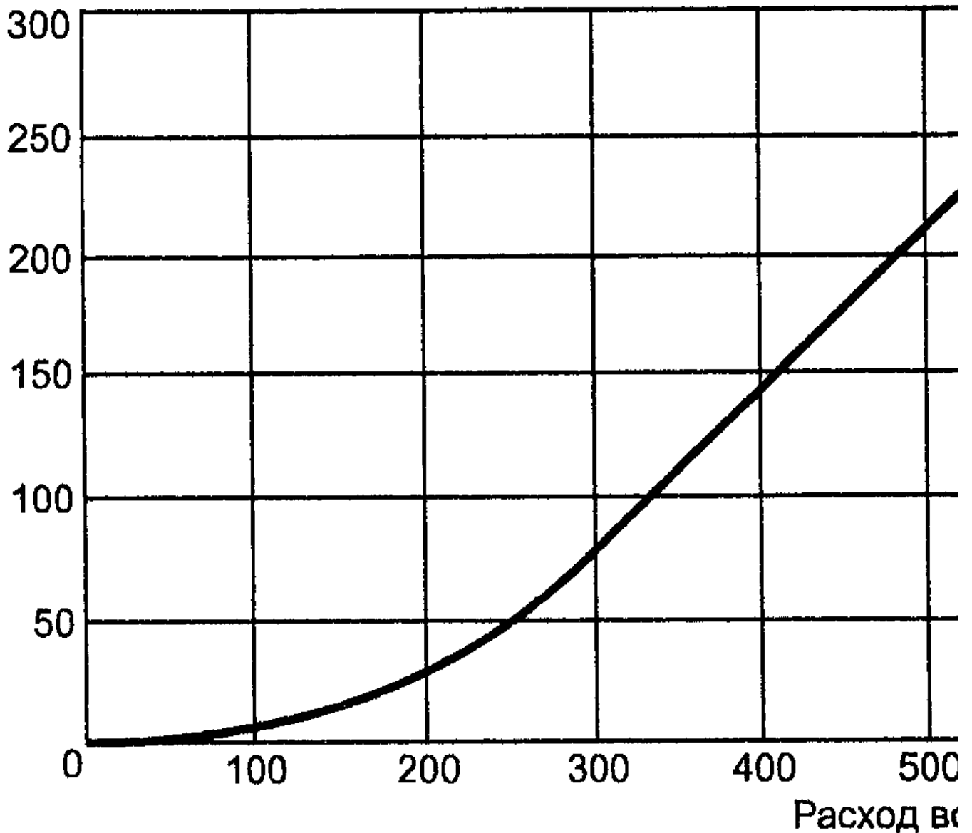
Рисунок 4. Калибровочная диаграмма капиллярной трубки (диаметр d = 2 мм; длина l = 70 мм) расходомера для измерения скорости потока воздуха в термостате по методу 2
