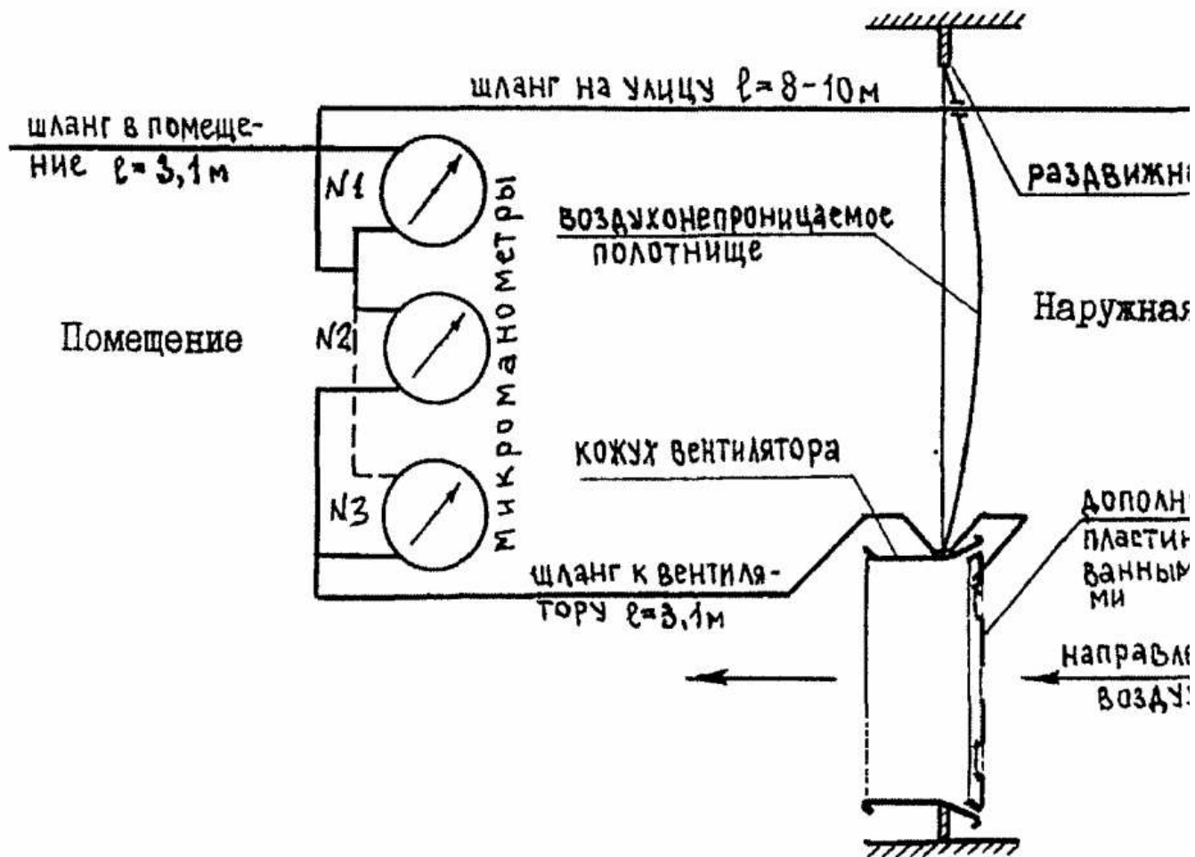
Рисунок 5. Схема монтажа установки при проведении испытаний на воздухопроницаемость
