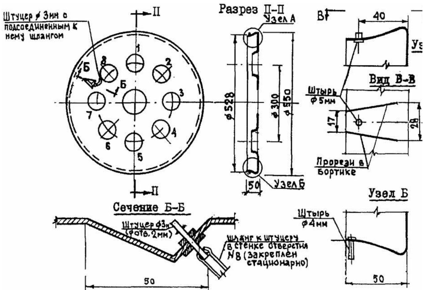
Рисунок 4. Пластина с отверстиями к кожуху вентилятора
