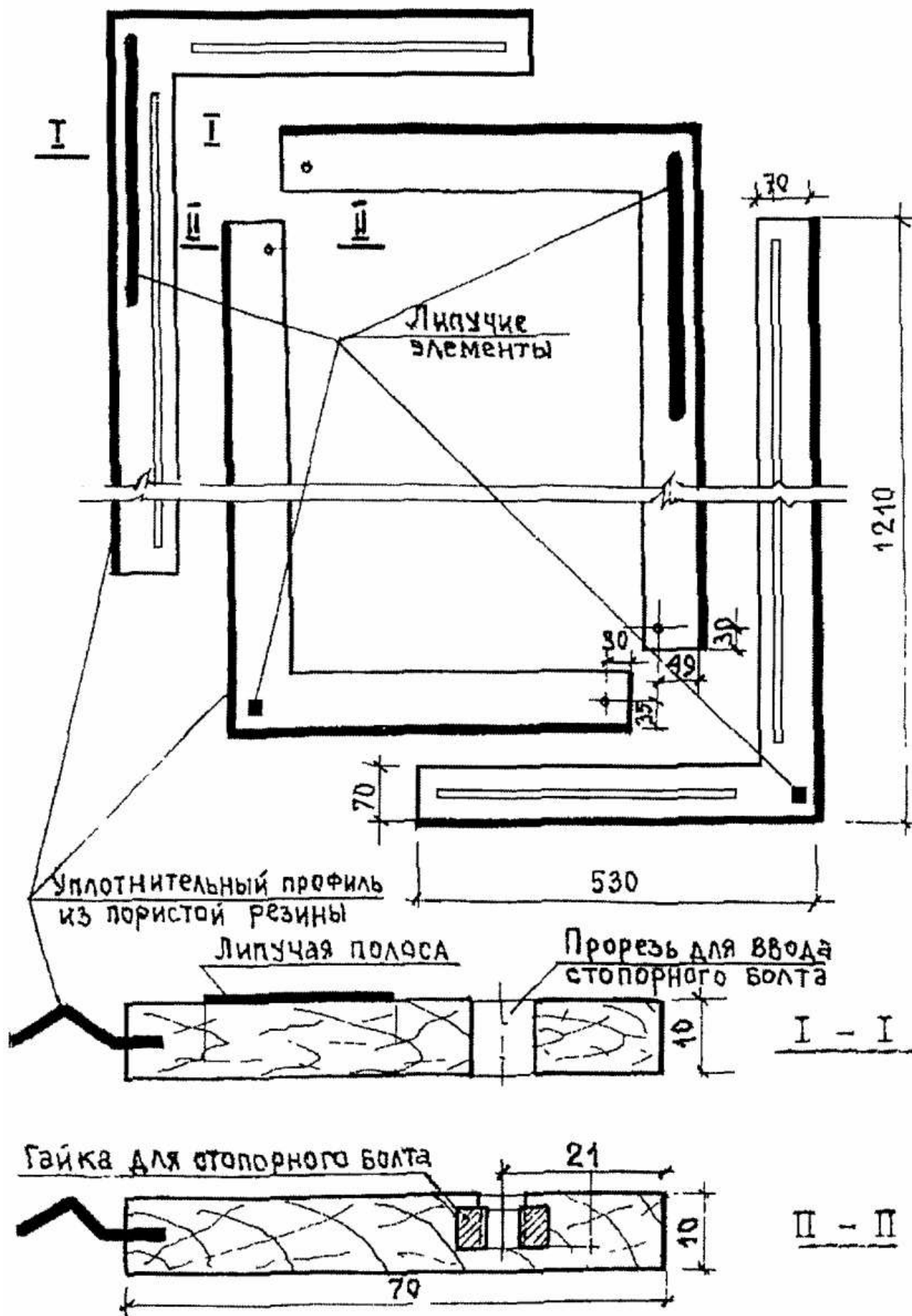
Рисунок 1. Элементы раздвижной деревянной рамы
