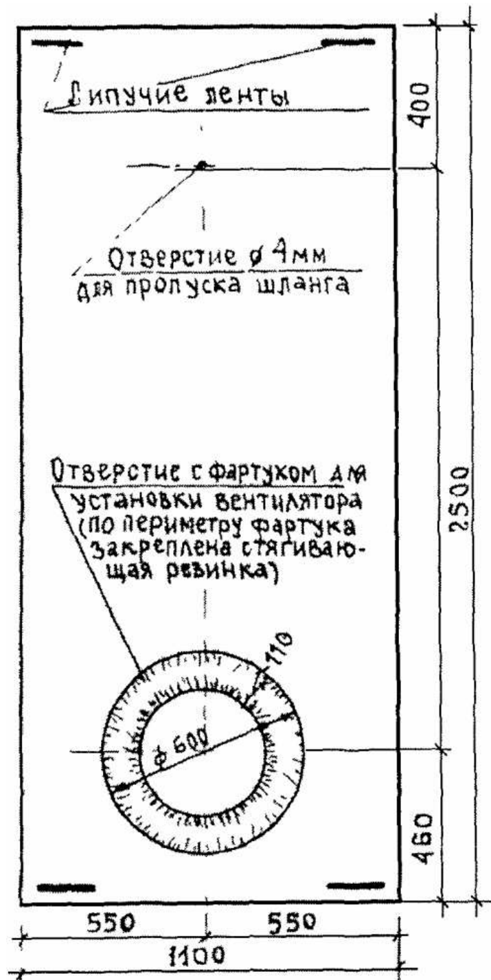
Рисунок 2. Воздухонепроницаемое полотнище
