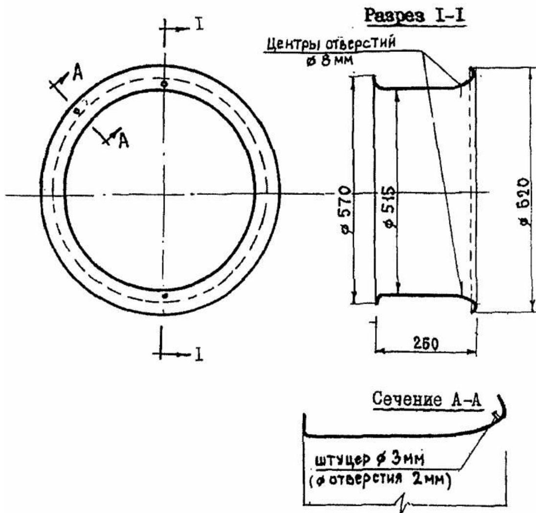
Рисунок 3. Кожух вентилятора
