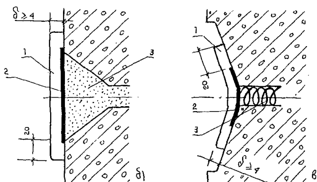
Рис. 1. Герметизация стыков тиоколовым герметиком: а) 1 - 3 - последовательность заполнения герметиком стыка; б) герметизация по жесткому основанию; в) герметизация по упругому основанию 1 - герметик; 2 - самоклеящаяся полимерная лента; 3 - стык
