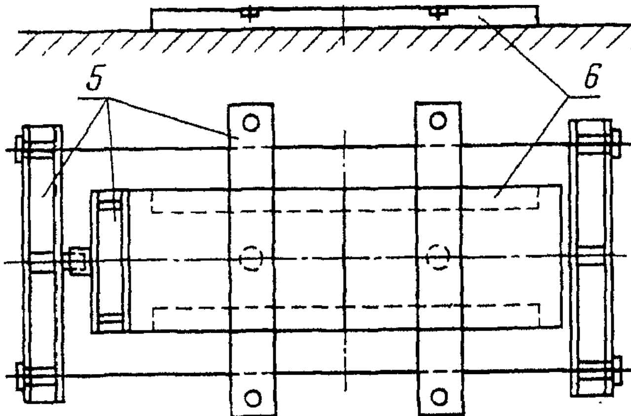
1 - звено трубы; 2 - металлические тяжи; 3 - гидродомкраты; 4 - слой цементно-песчаного раствора; 5 - металлические траверсы; 6 - опоры; - вертикальная нагрузка; - горизонтальная нагрузка
