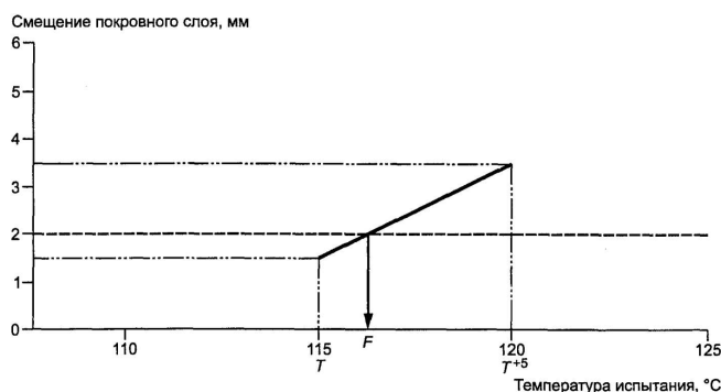
Рисунок 2. Пример определения предельного значения теплостойкости интерполяцией
