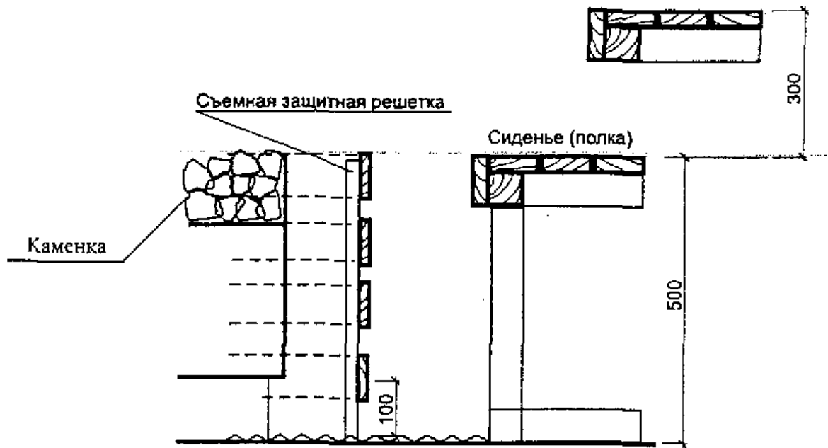
Рис. 6.2 Варианты решений и оборудование саун
