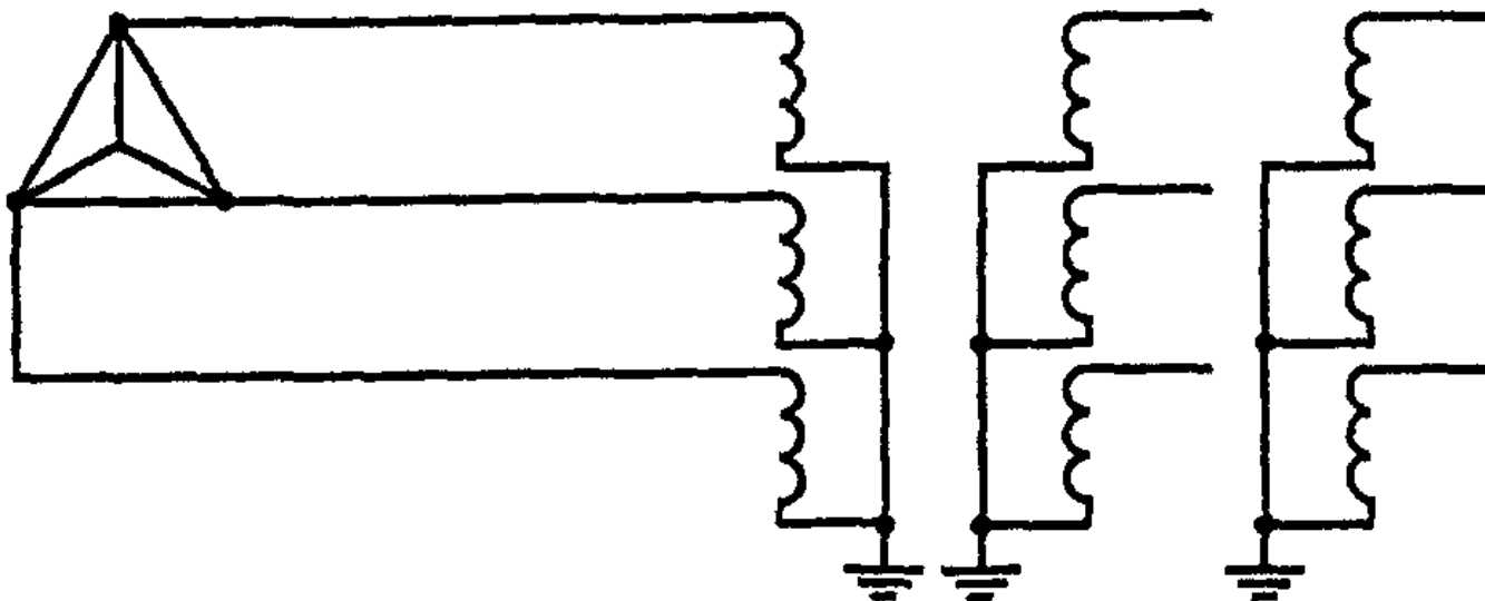
Рисунок Б.6. Схема включения однофазных заземляемых и трехфазных заземляемых трехобмоточных трансформаторов с двумя основными вторичными обмотками в трехфазных электрических сетях с изолированной нейтралью и напряжением 3 - 35 кВ
