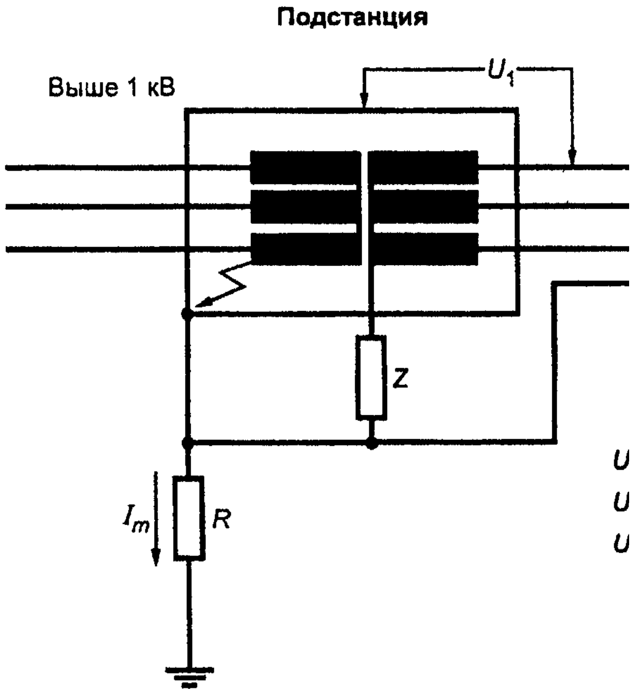
2) Первое замыкание в установке до 1 кВ
