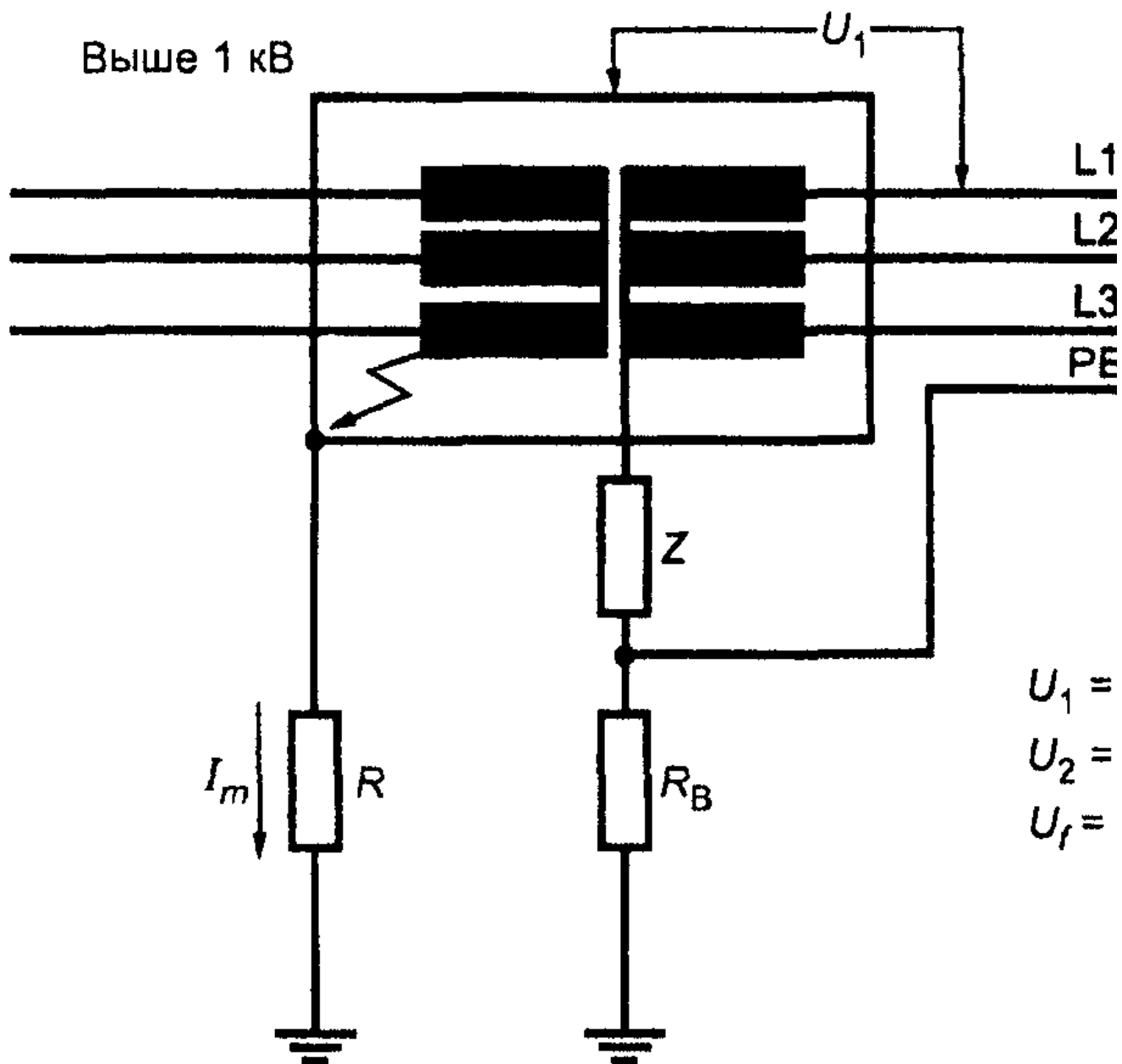
1) В установке до 1 кВ замыкания нет
