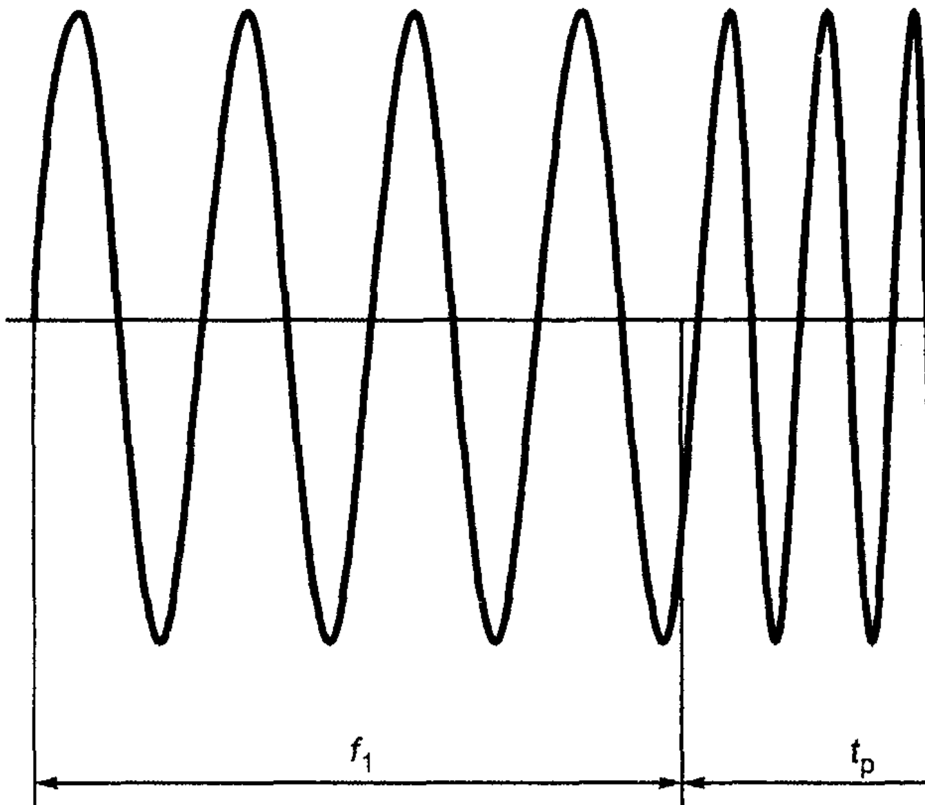
Рисунок 2. Пример изменения частоты в течении переходного интервала времени
