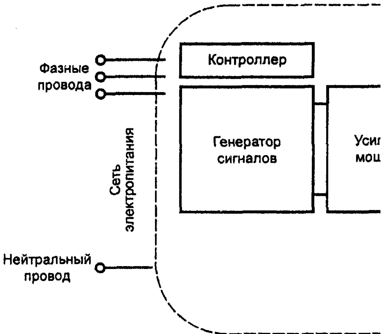
Рисунок 3. Схема испытательного оборудования с усилителем мощности
