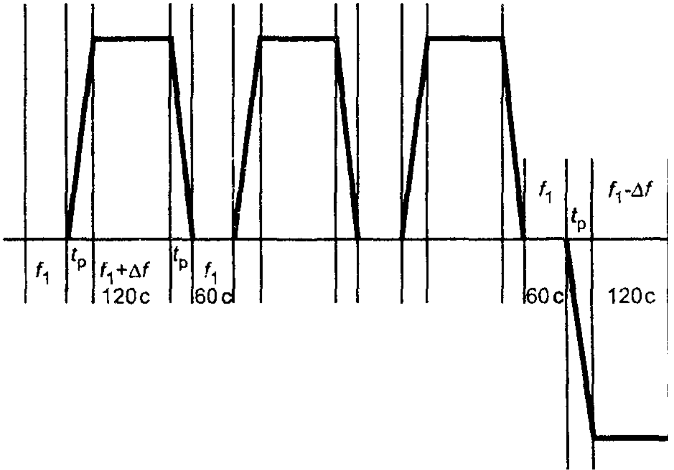
Рисунок 1. Последовательность изменений частоты
