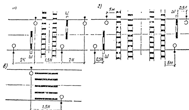
Рис. 3. Схемы размещения светильников а, б - на железнодорожных переездах; в - на пешеходном переходе; г - автоматический шлагбаум
