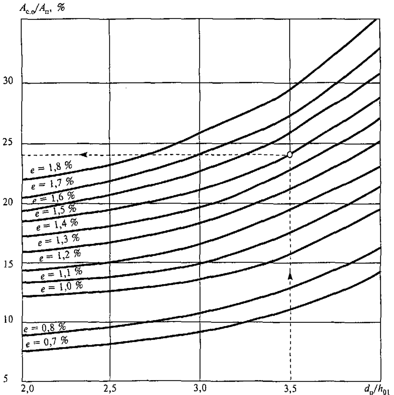
Рисунок 3. График для определения относительной площади световых проемов при боковом освещении школьных классов
