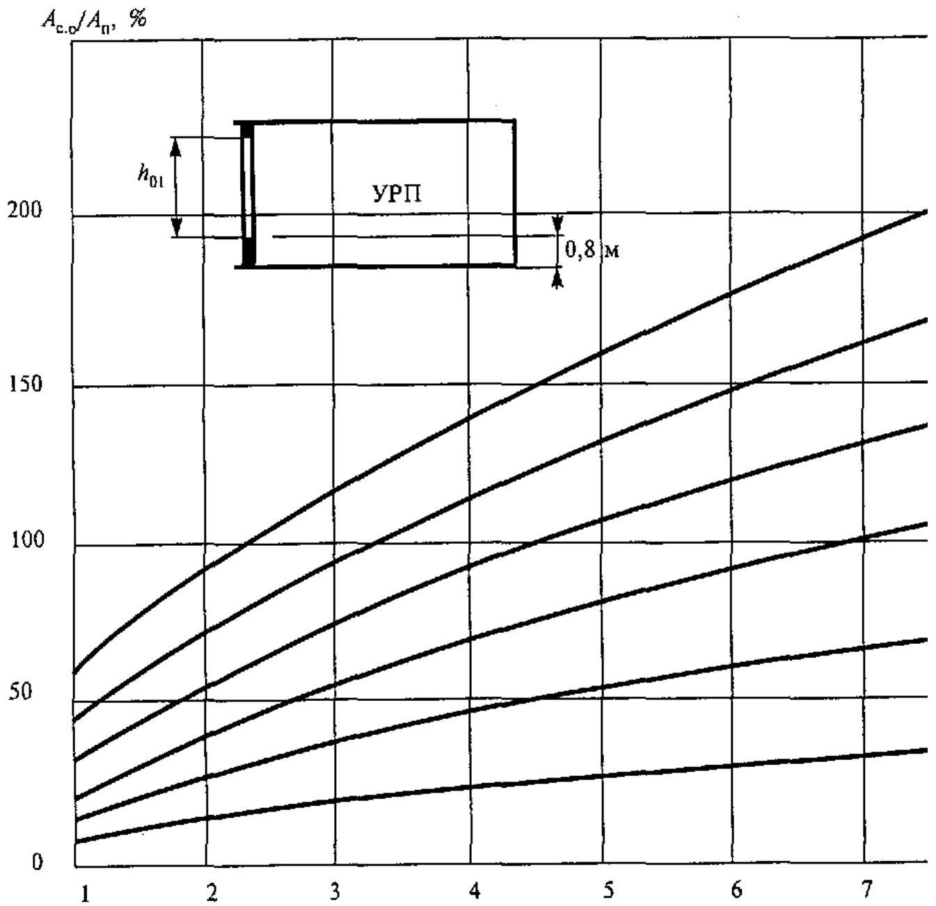
Рисунок 2. График для определения относительной площади световых проемов при боковом освещении помещений общественных зданий
