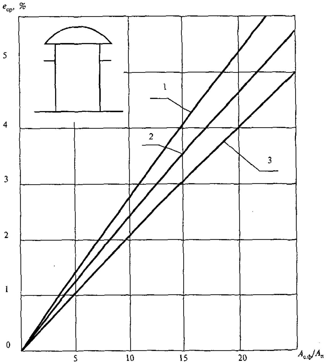
Рисунок 5. График для определения среднего значения КЕО в общественных помещениях с шахтными фонарями с глубиной светопроводной шахты 3,50 м и размерами в плане, м: 1 - 2,9 x 5,9; 2 - 2,7 x 2,7; 2,9 x 2,9; 1,5 x 5,9; 3 - 1,5 x 1,7
