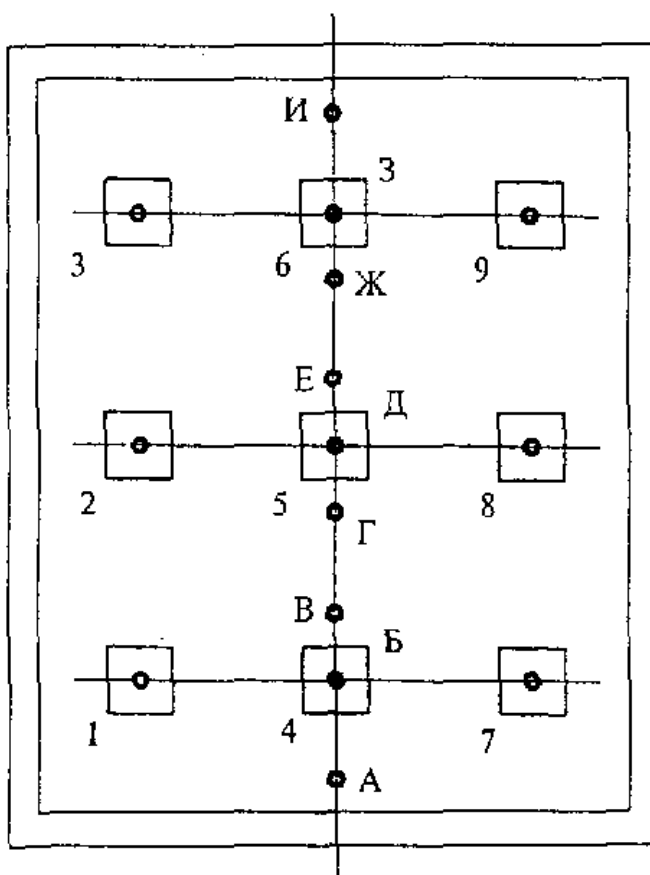
Рисунок 24. Схема размещения шахтных фонарей
