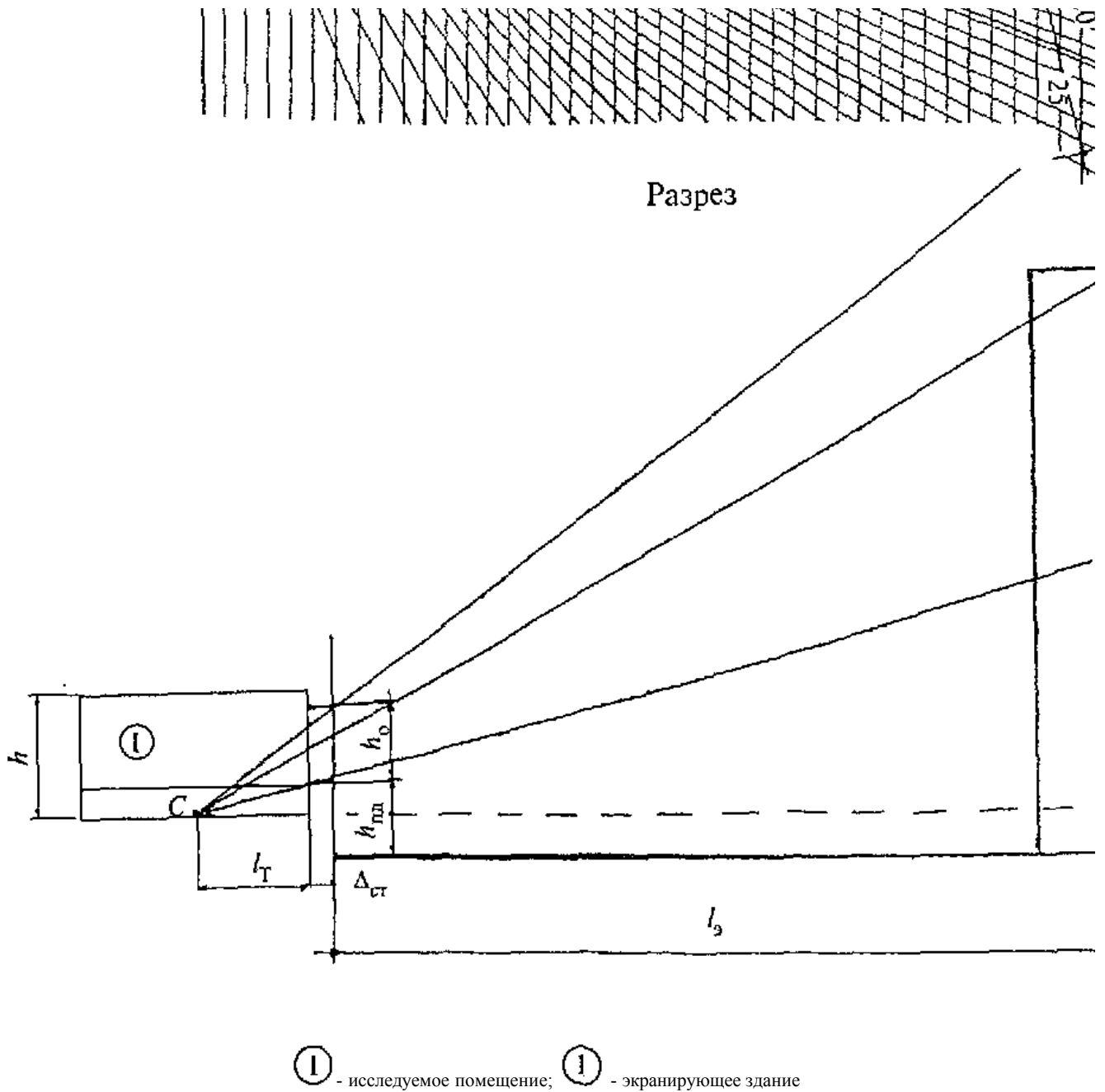
Рисунок Б.3. Схема N 2 к определению параметров застройки при расположении экранирующего здания под углом к исследуемому
