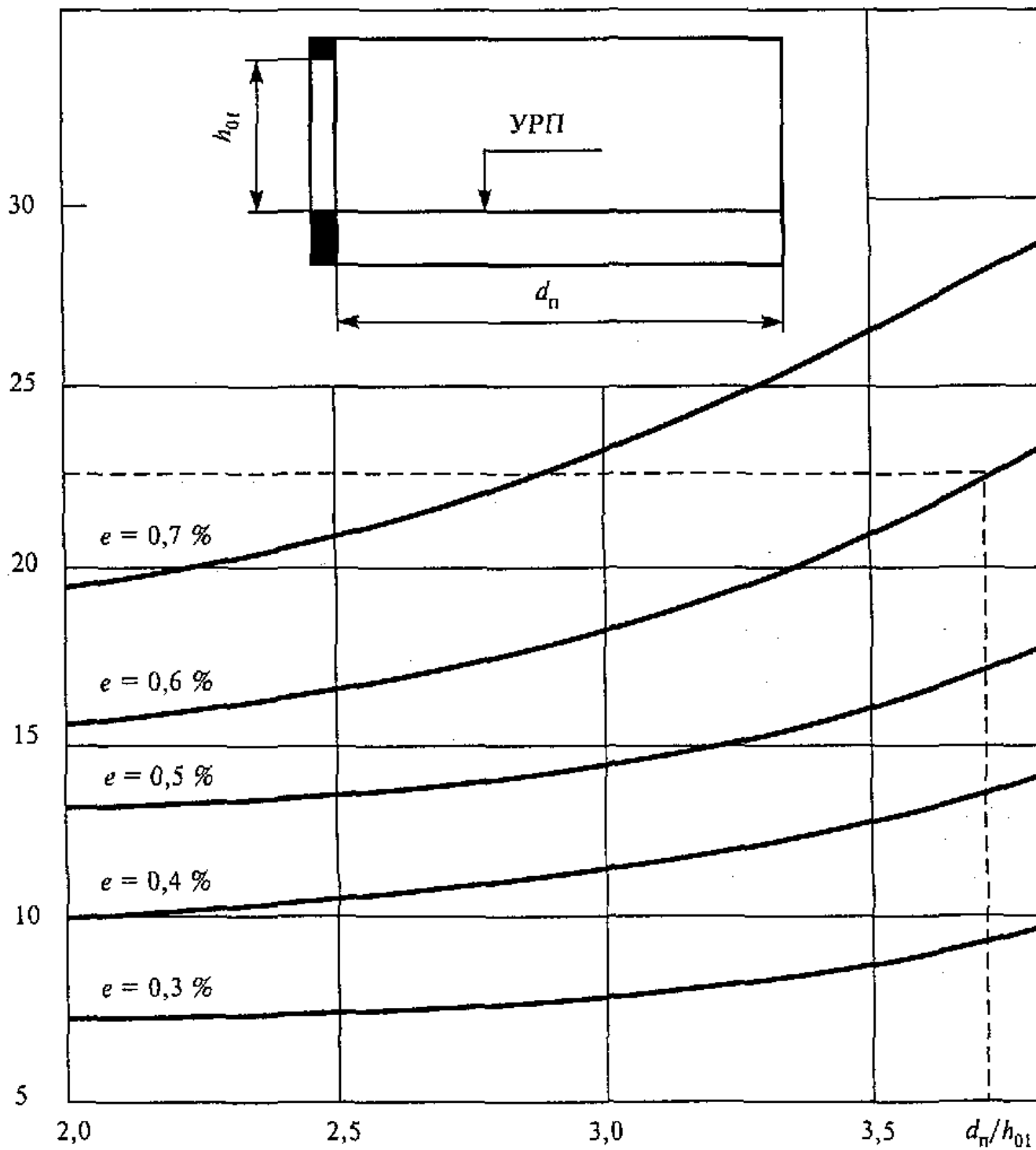
Рисунок 1. График для определения относительной площади световых проемов при боковом освещении жилых помещений
