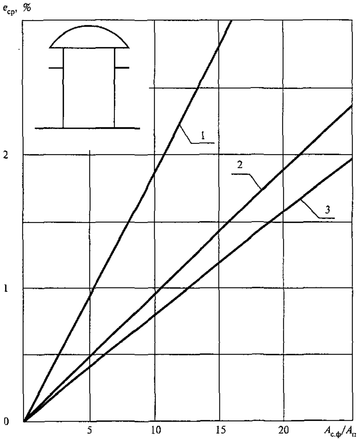
Рисунок 6. График для определения среднего значения КЕО в общественных помещениях с шахтными фонарями диффузного света с глубиной светопроводной шахты 3,50 м и размерами в плане, м: 1 - 2,9 x 5,9; 2 - 2,7 x 2,7; 2,9 x 2,9; 1,5 x 5,9; 3 - 1,5 x 1,7
