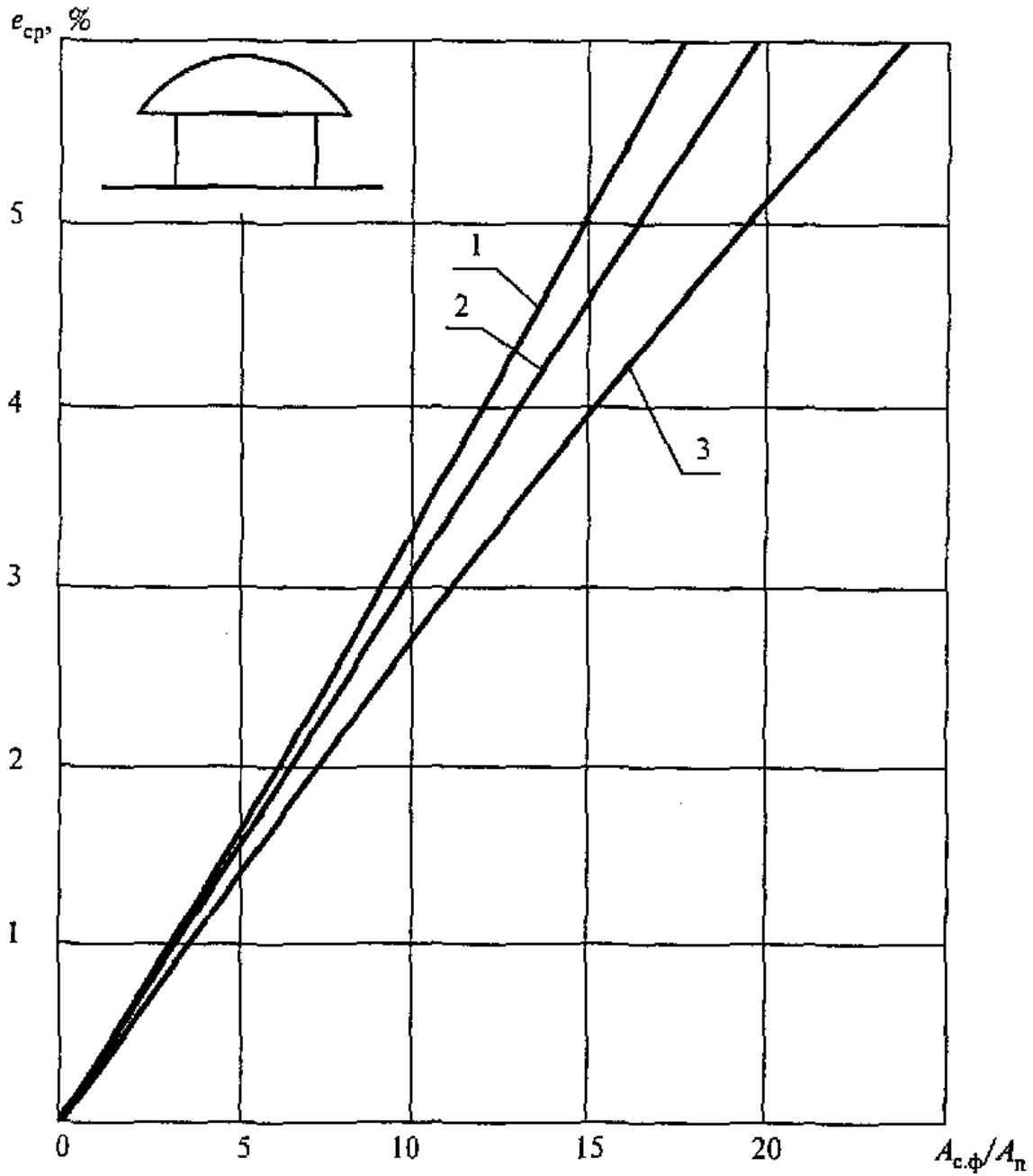
Рисунок 4. График для определения среднего значения КЕО в помещениях с зенитными фонарями с глубиной проема до 0,7 м и размерами в плане, м: 1 - 2,9 x 5,9; 2 - 2,7 x 2,7; 2,9 x 2,9; 1,5 x 5,9; 3 - 1,5 x 1,7
