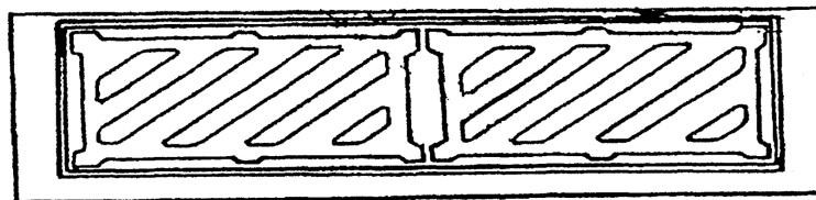
Рисунок Б.2. Дождеприемник с минимальной шириной продольной опорной части корпуса, прилегающего к бордюру дороги
