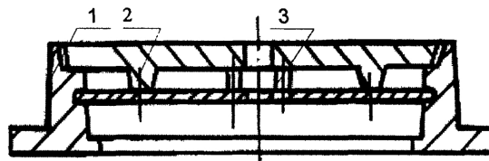
Рисунок А.1. Люк общего назначения 1 - крышка; 2 - корпус; 3 - опорная поверхность корпуса
