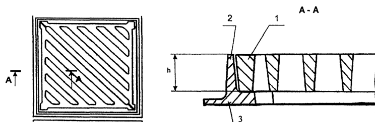
Рисунок Б.1. Дождеприемник ливнесточного колодца 1 - крышка; 2 - корпус; 3 - опорная поверхность корпуса
