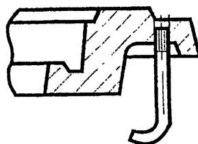
Рисунок А.3. Люк с крышкой, имеющей углубление под заполнение бетоном 1 - крышка; 2 - бетон; 3 - корпус
