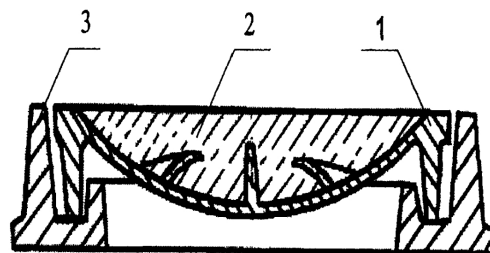
Рисунок А.2. Люк, оснащенный запорным замковым устройством 1 - корпус; 2 - крышка; 3 - замковый механизм
