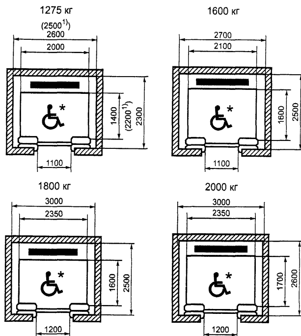
Рисунок 5. Лифты скоростью 2,50 м/с и более для зданий большой этажности и заселенности с интенсивными пассажиропотоками
