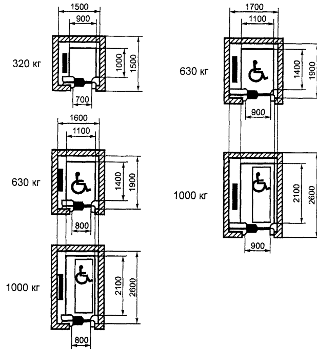
Рисунок 3. Пассажирские лифты для жилых зданий
