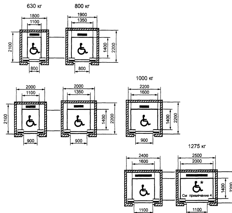
Рисунок 4. Пассажирские лифты для общественных и промышленных зданий (сооружений)
