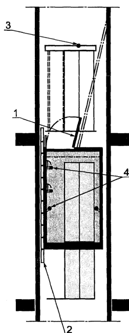
1 - люк; 2 - переносная лестница, закрепленная снаружи кабины лифта; 3 - замок шахтной двери; 4 - точки в купе кабины,
