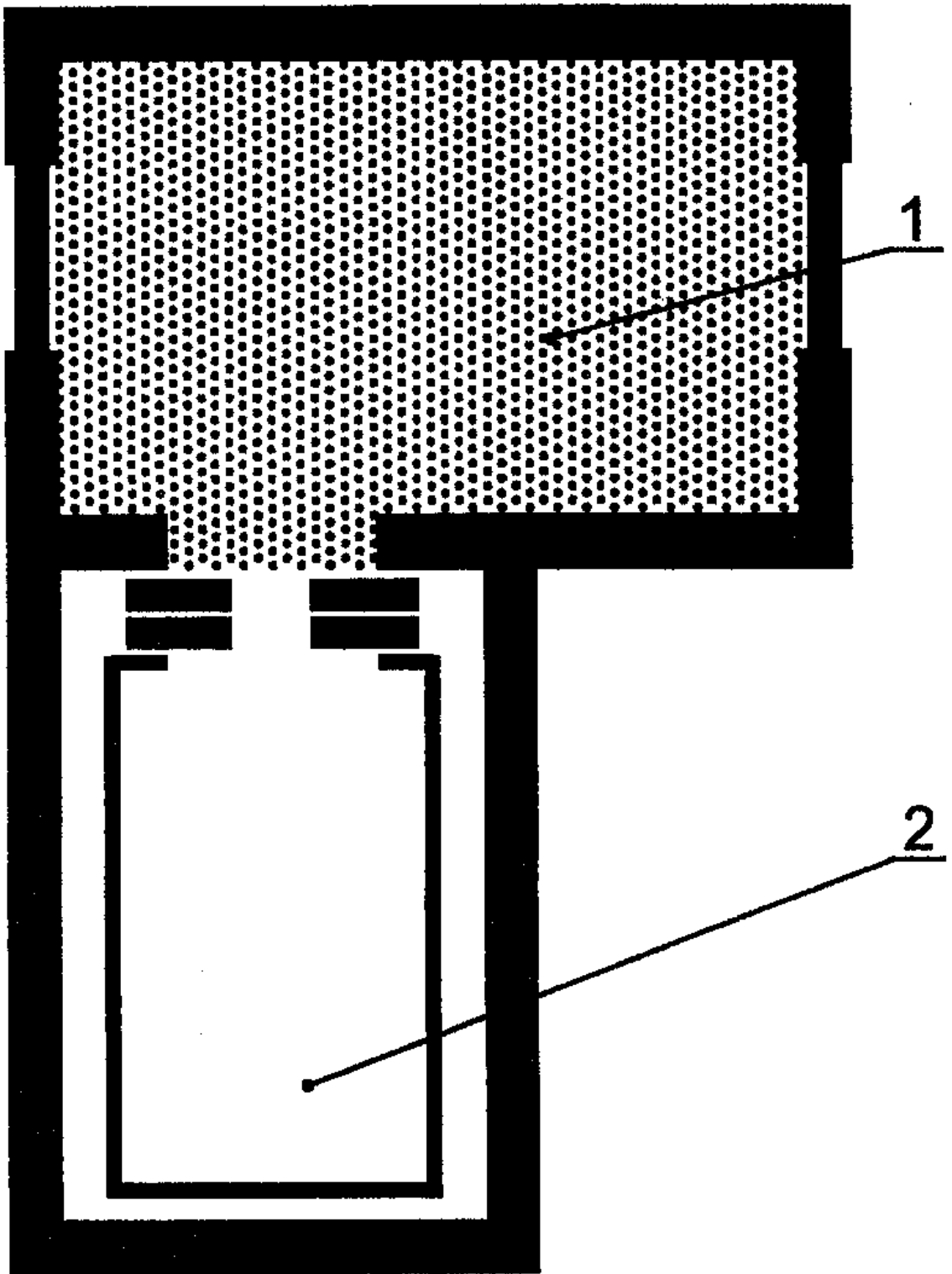
1 - пожарозащищенный лифтовой холл; 2 - лифт для пожарных
