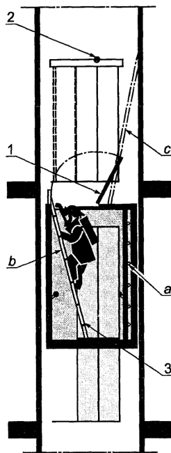
1 - люк; 2 - замок шахтной двери; 3 - переносная лестница
