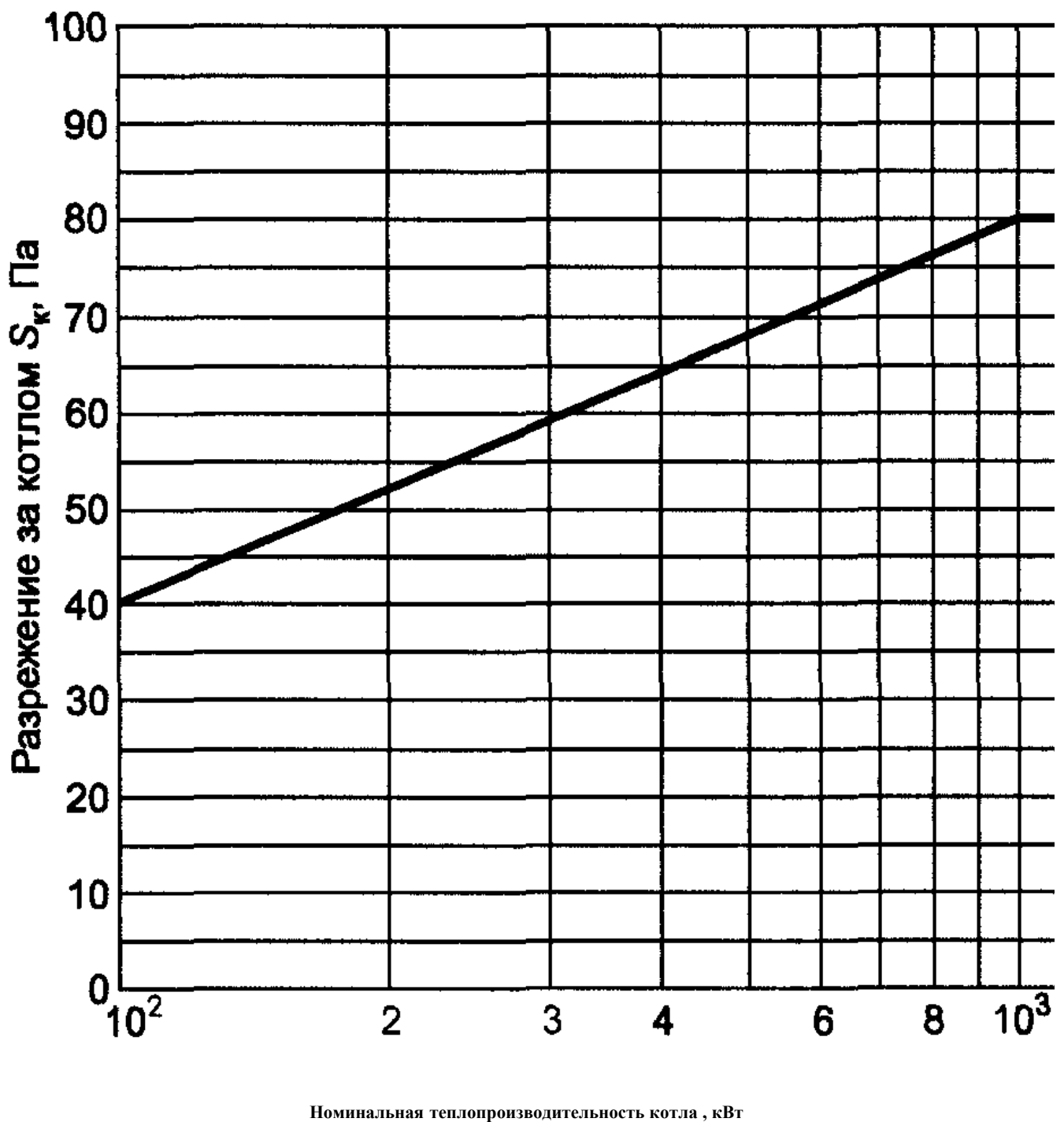
Рисунок 2. Максимальное разрежение за котлом на естественной тяге
