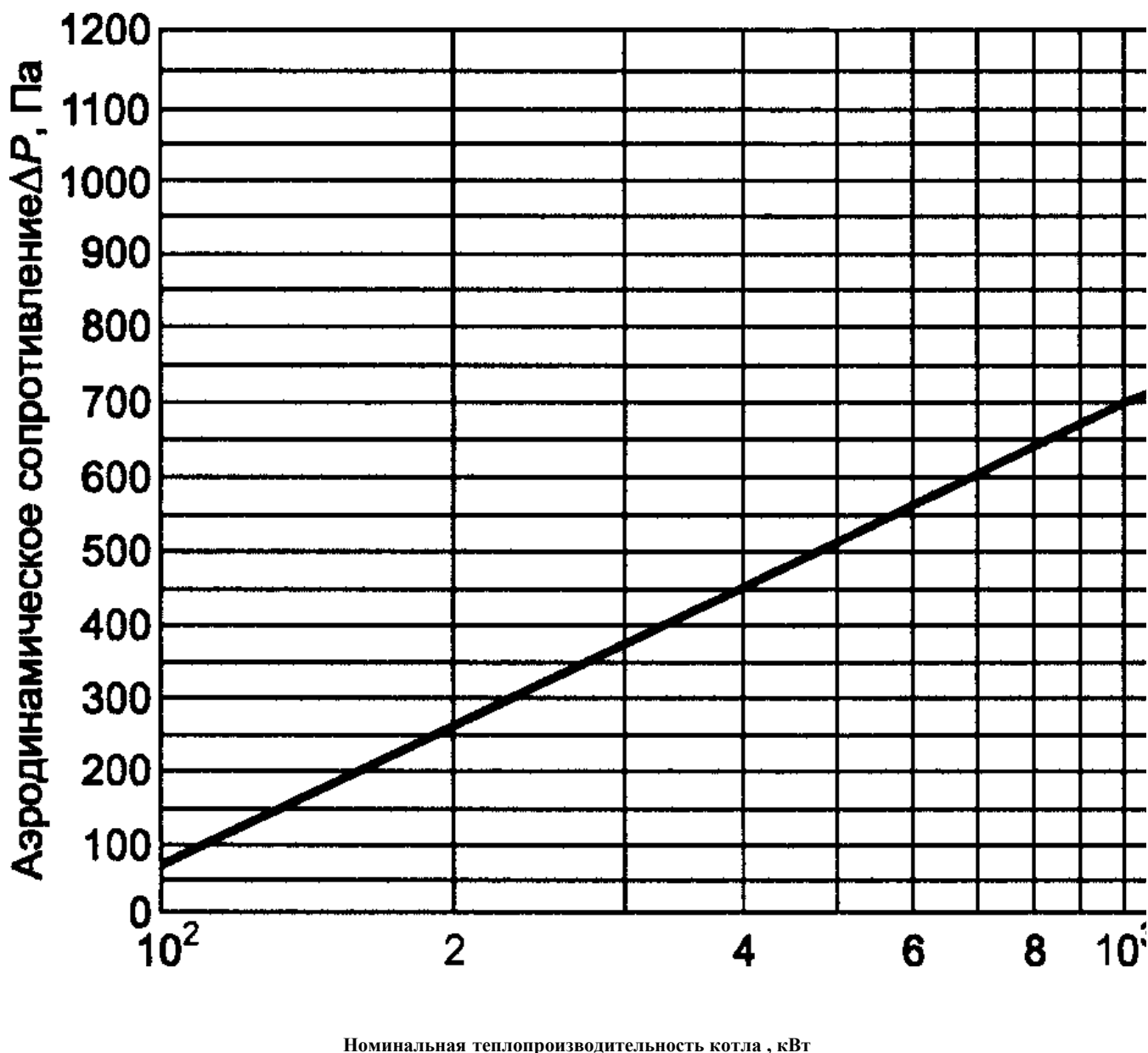
Рисунок 3. Максимальное аэродинамическое сопротивление котла на принудительной тяге или под наддувом
