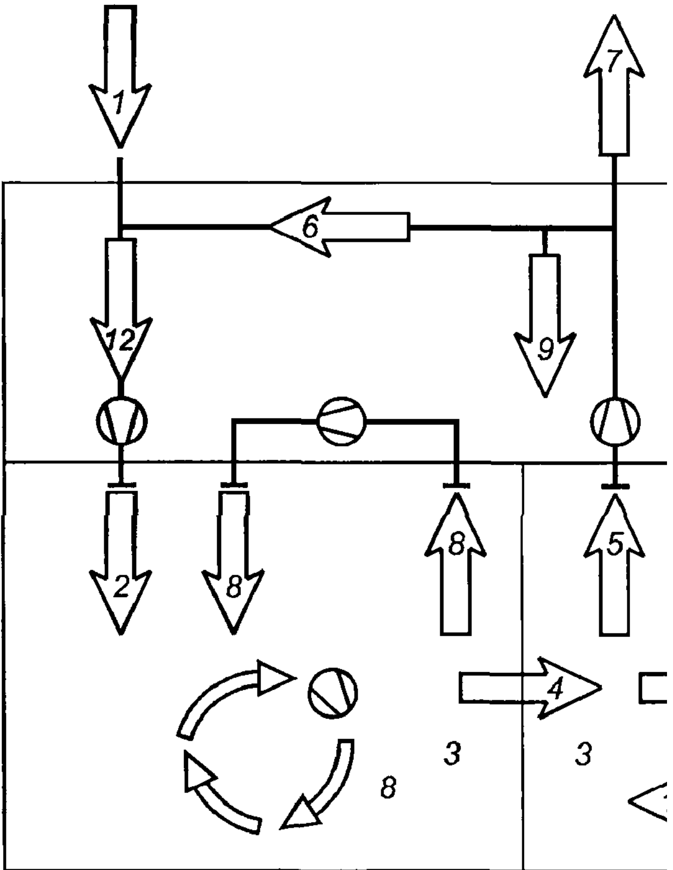
Рисунок 1. Типы потоков воздуха. Номера позиций соответствуют таблице 2
