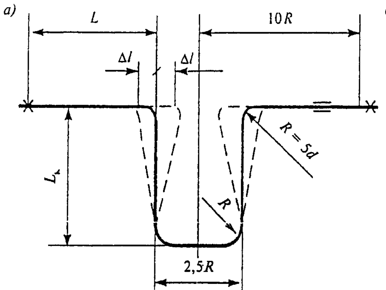
Рисунок 1. Устройство П-образного (а) и Г-образного (б) компенсаторов
