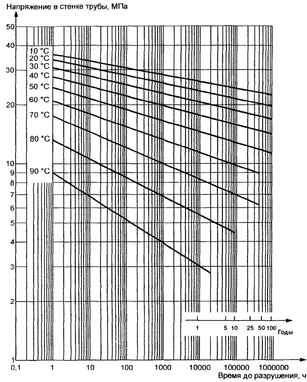
Рисунок В.6. Эталонные кривые длительной прочности материала труб PVC-C Тип I
