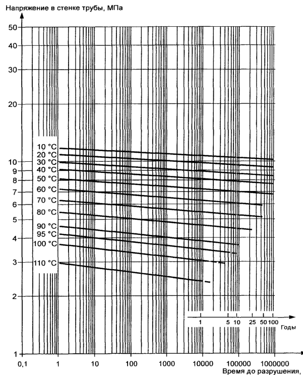
Рисунок В.14. Эталонные кривые длительной прочности PE-RT Тип I
