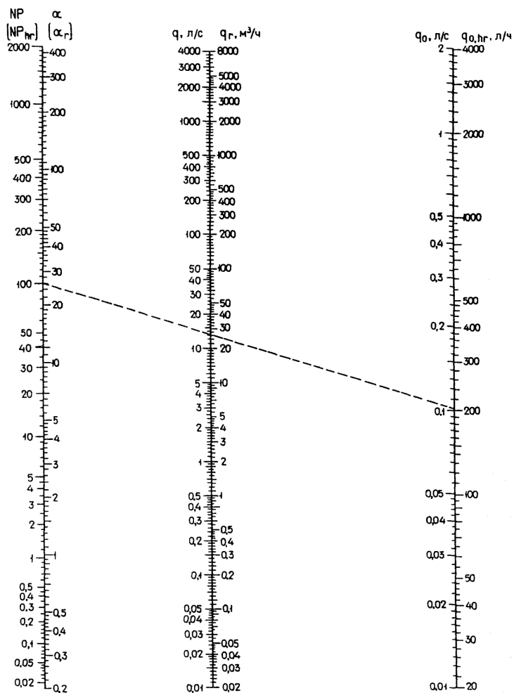
Черт. 4. Номограмма для определения секундных и часовых расходов воды в зависимости от NP ( ) при различных значениях , л/с, и , л/ч
