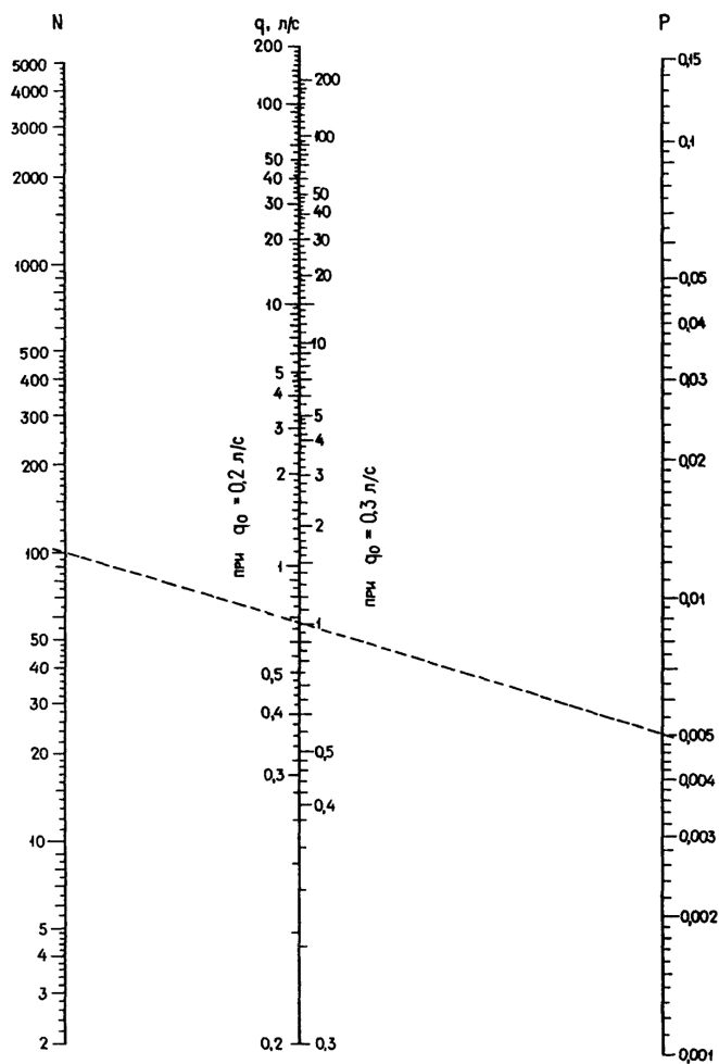
Черт. 2. Номограмма для определения секундных расходов воды q при = 0,2 и 0,3 л/с и P 0,15
