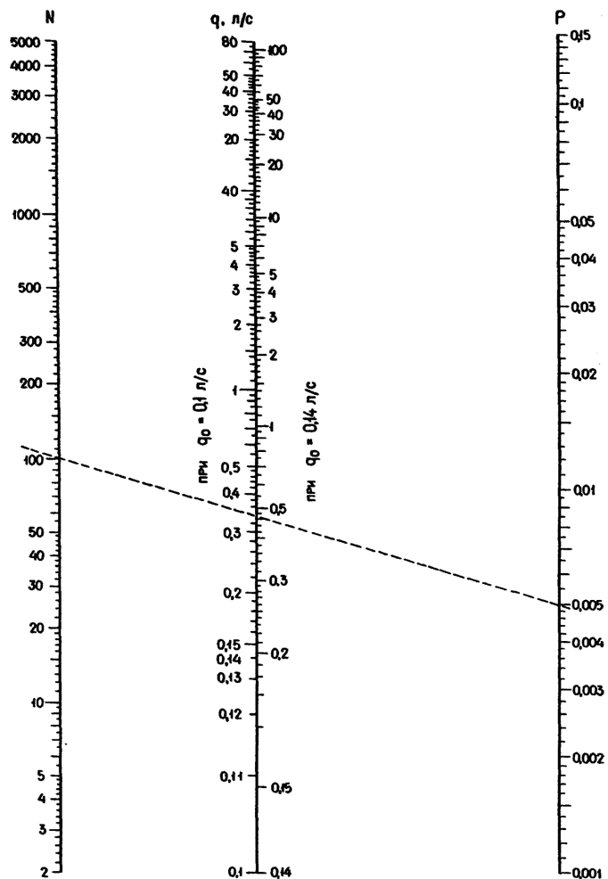
Черт. 1. Номограмма для определения секундных расходов воды q при q_0 = 0,1 и 0,14 \text{ л/с} и P = 0,15
