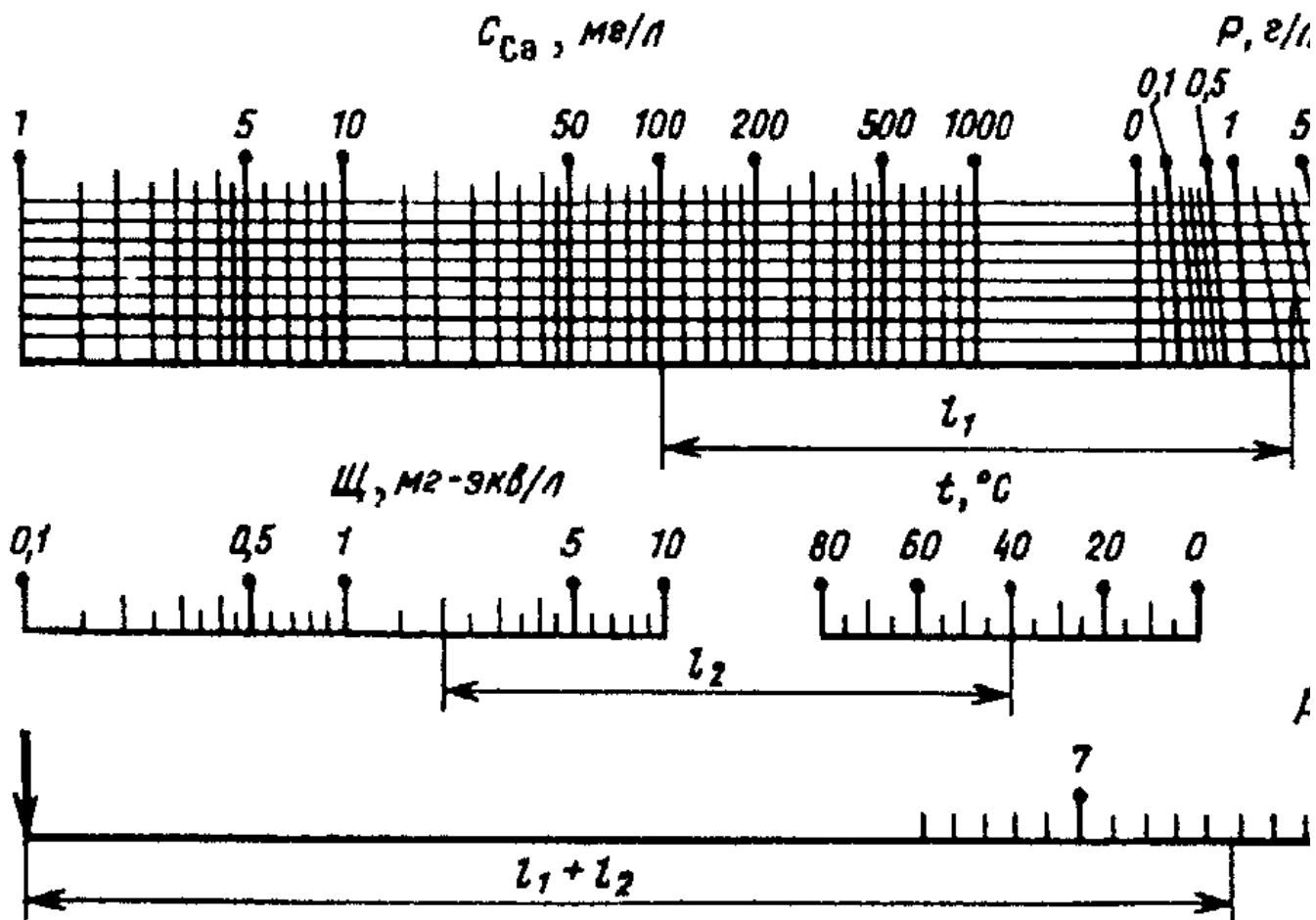
Рис. 1. Номограмма для определения pH насыщения воды карбонатом кальция ()
