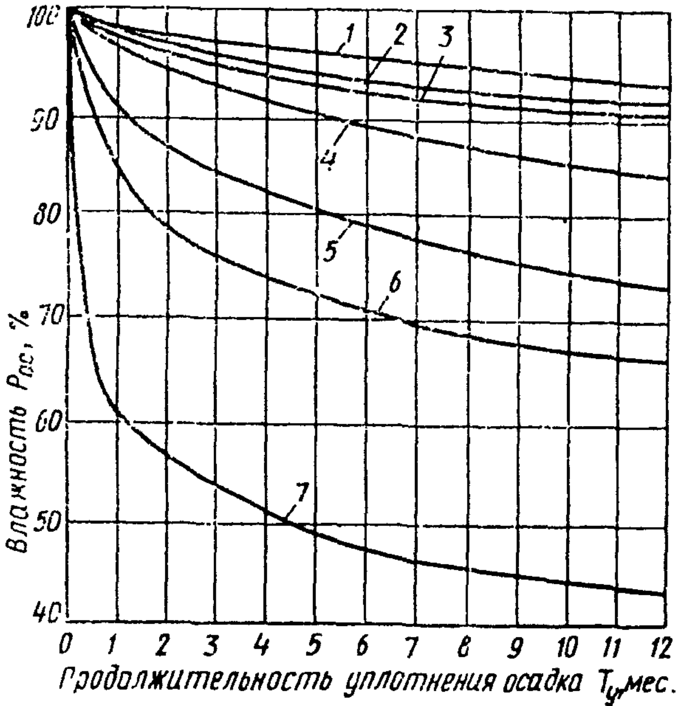
Рис. 3. Средние значения влажности осадка станций осветления и обезвреживания воды при уплотнении до одного года
