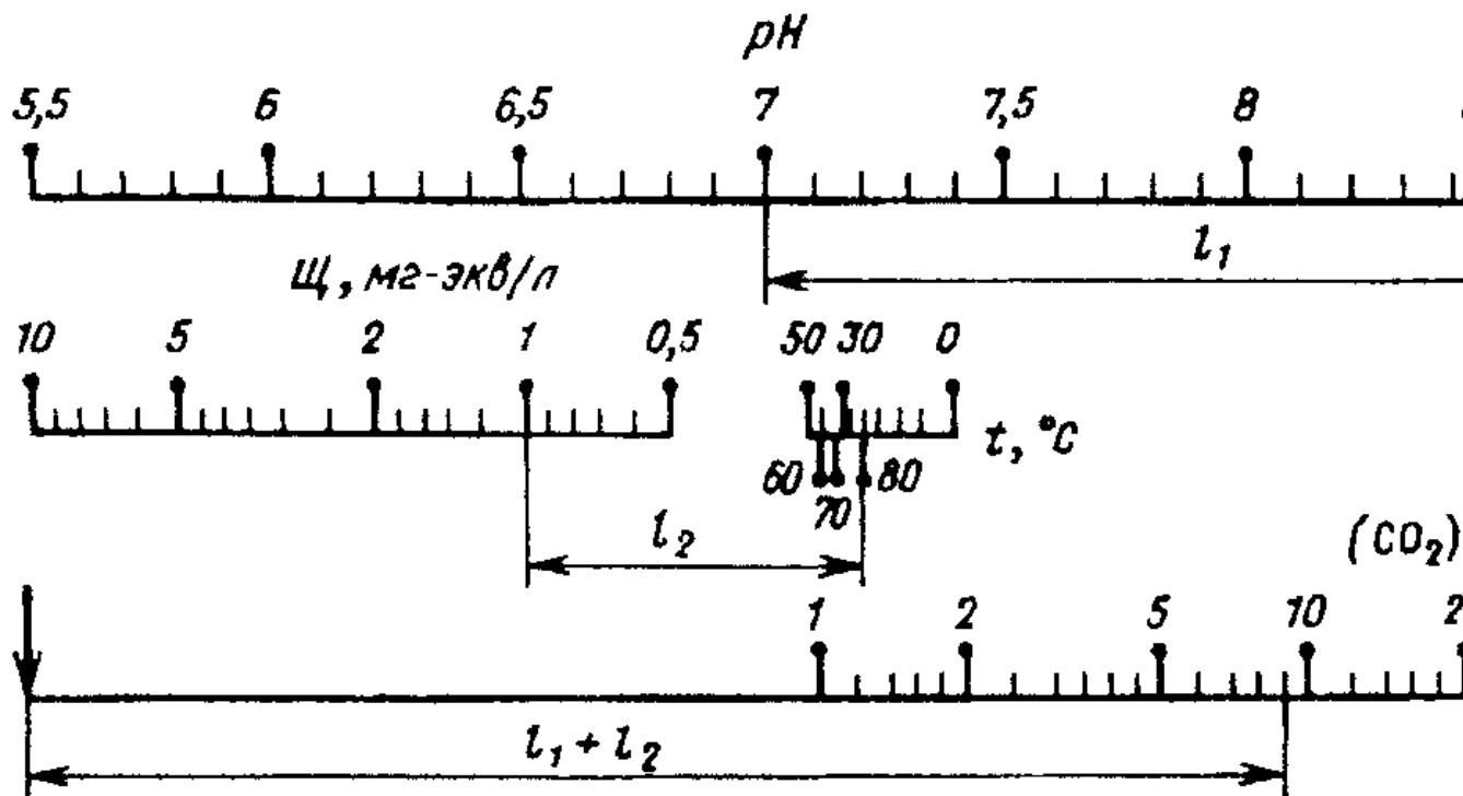
Рис. 2. Номограмма для определения концентрации свободной двуокиси углерода в природной воде (или pH)
