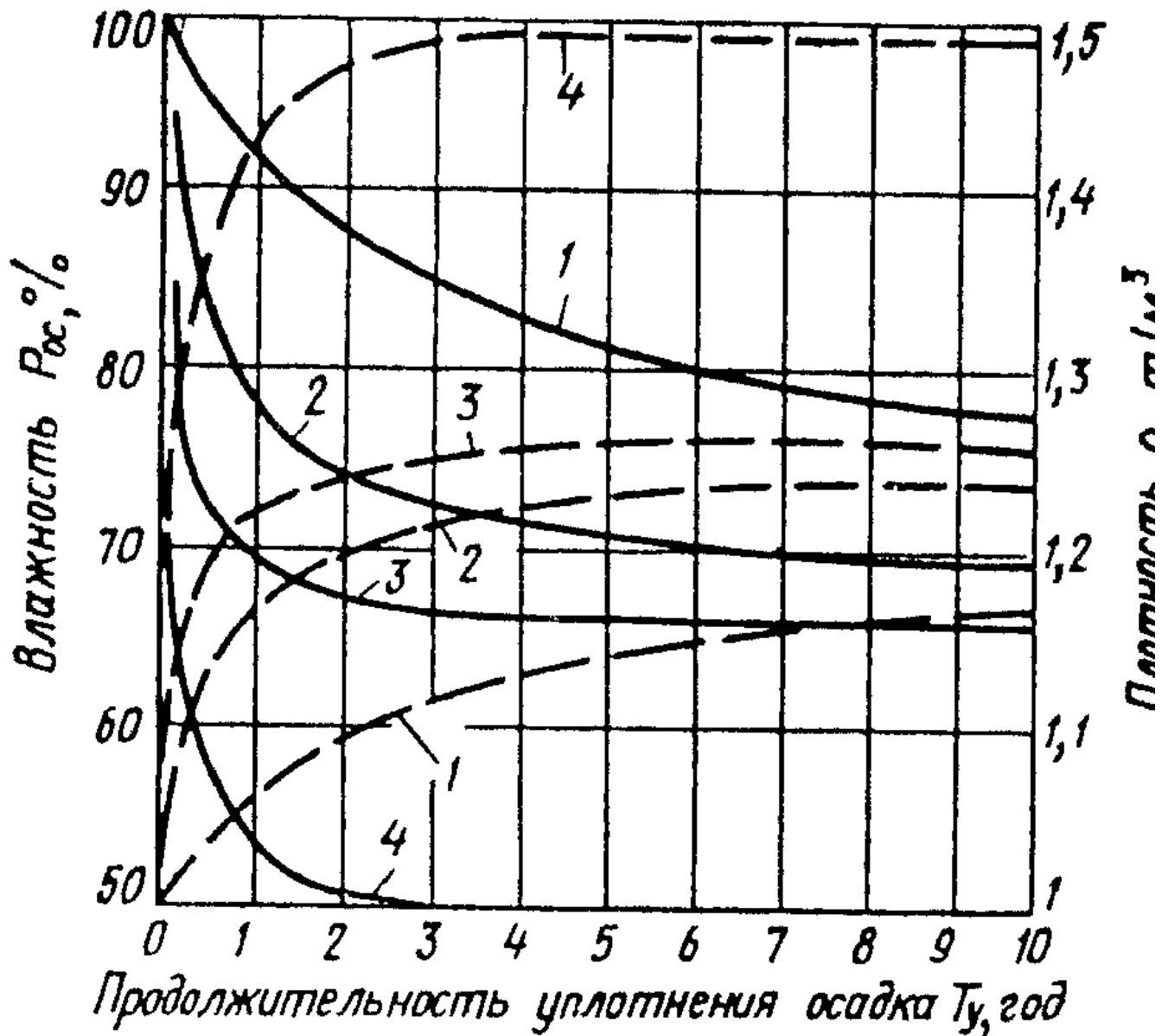
Рис. 2. Средние значения влажности и плотности осадка станций обезжелезивания или реагентного умягчения воды при многолетнем уплотнении
