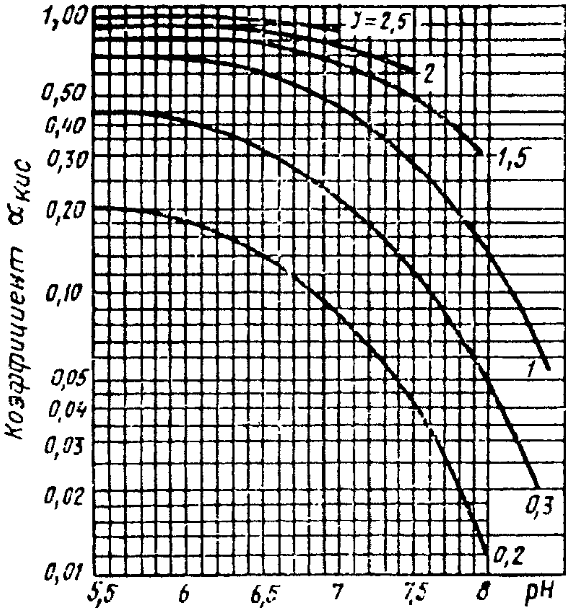
Рис. 3. Номограмма для определения коэффициента при расчете дозы кислоты
