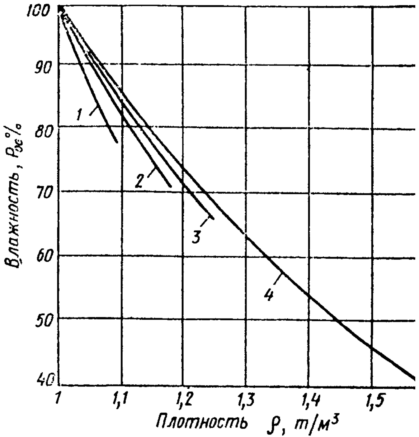
Рис. 5. Значения плотности в зависимости от влажности осадка станций осветления и обесцвечивания воды
