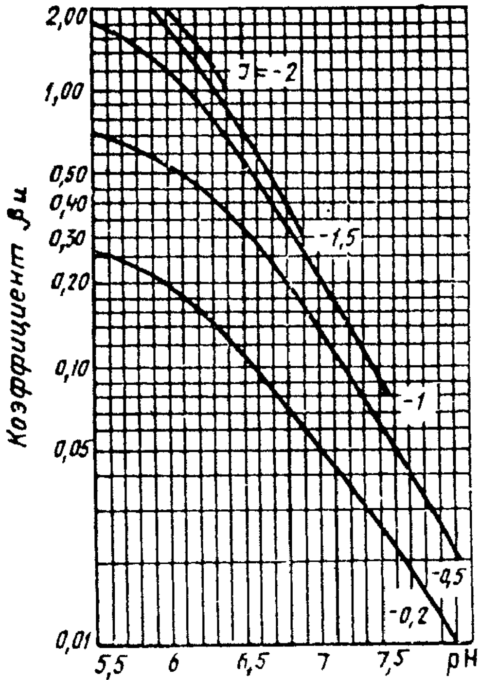
Рис. 4. Номограмма для определения коэффициента при расчете дозы щелочи
