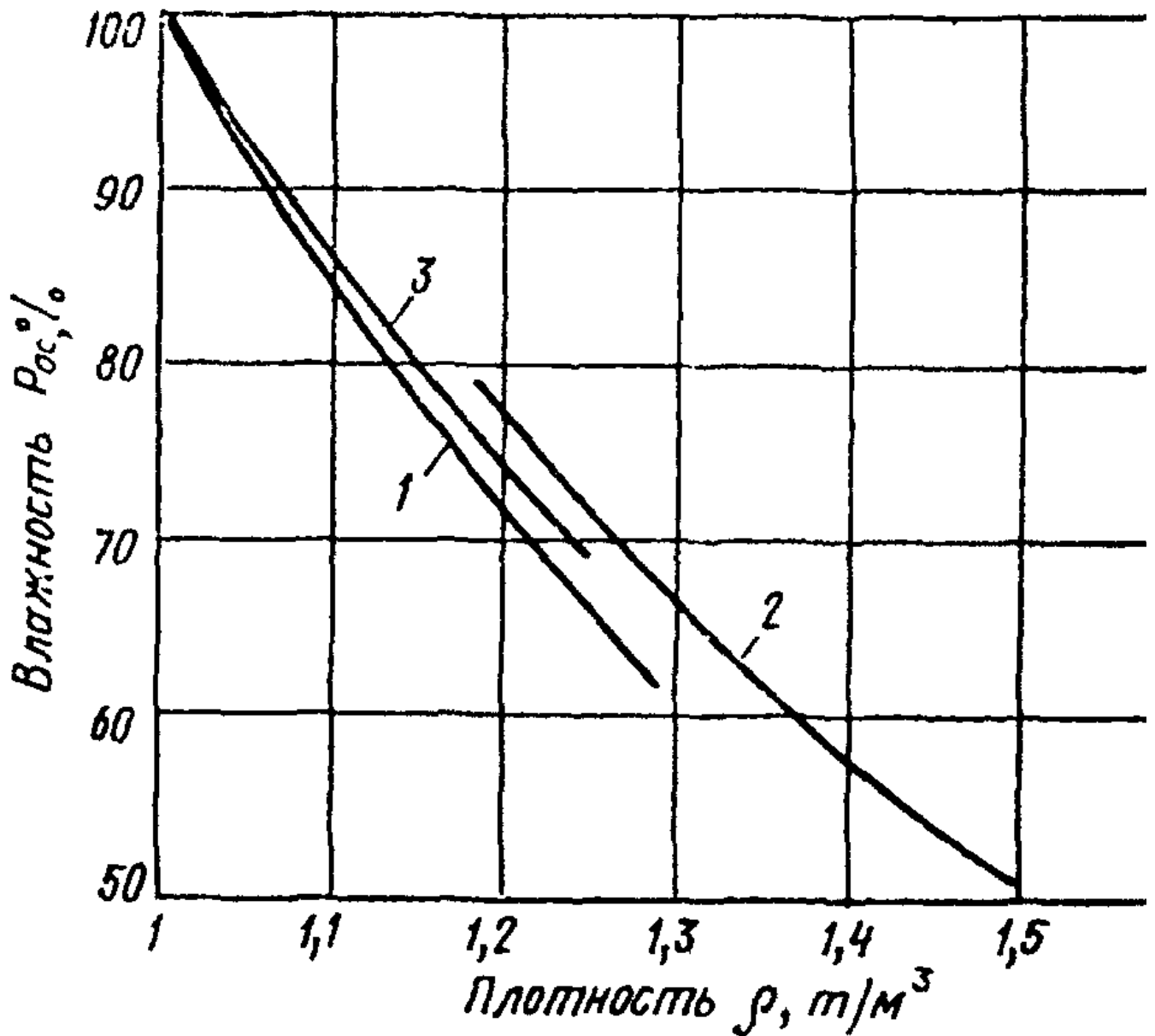
Рис. 6. Значения плотности в зависимости от влажности осадка станций обезжелезивания и реагентного умягчения воды
