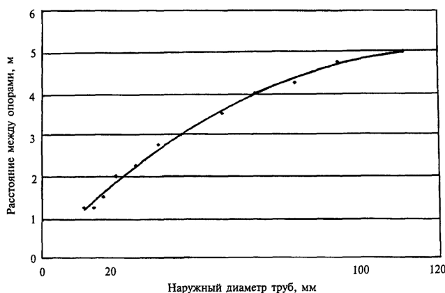
Рисунок 1. График для выбора расстояний между креплениями горизонтальных трубопроводов из твердых медных труб
