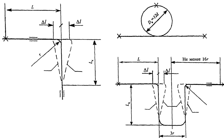
а - отводообразных; б - круговых; в - П-образных Рисунок Д.1. Расчетные схемы гнутых компенсаторов
