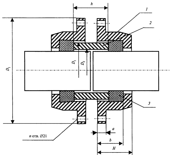
1 - муфта; 2 - втулка; 3 - резиновое кольцо
