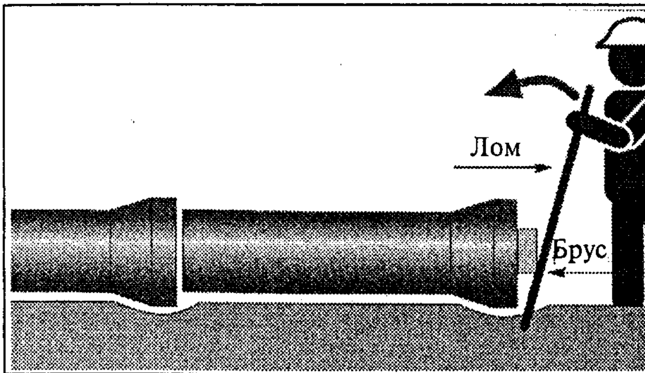
а - при помощи лома и деревянного бруса (для 100 мм)
