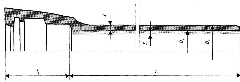
Рисунок А.1. Схема трубы раструбной под соединение "Тайтон"
