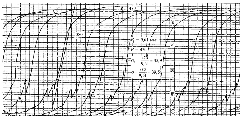
Рисунок 3.3. Диаграммы растяжения образца из ВЧШГ при заводских испытаниях ОАО Липецкий металлургический завод "Свободный Сокол"
