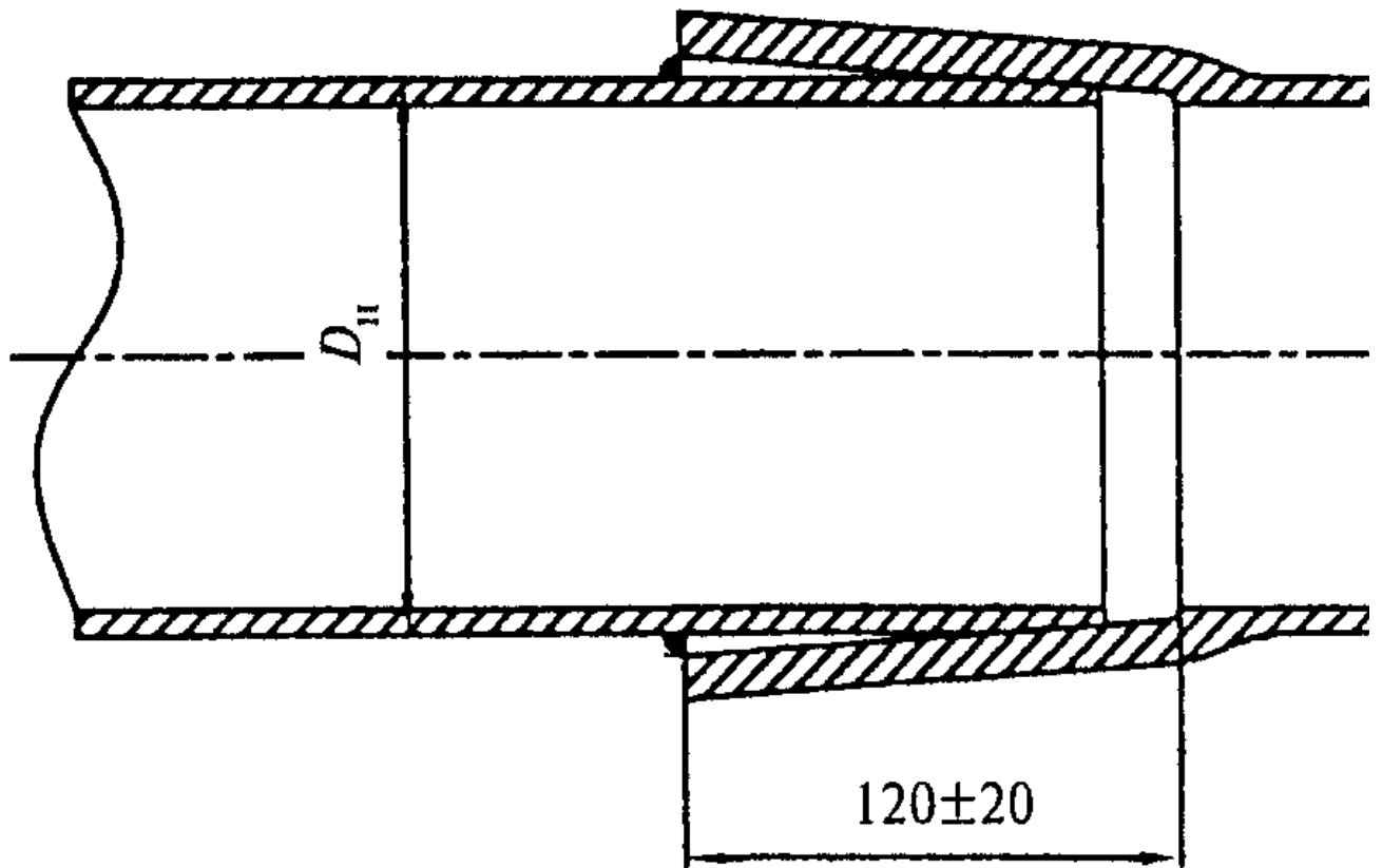
Рисунок А.5. Схема сварного нахлестного соединения
