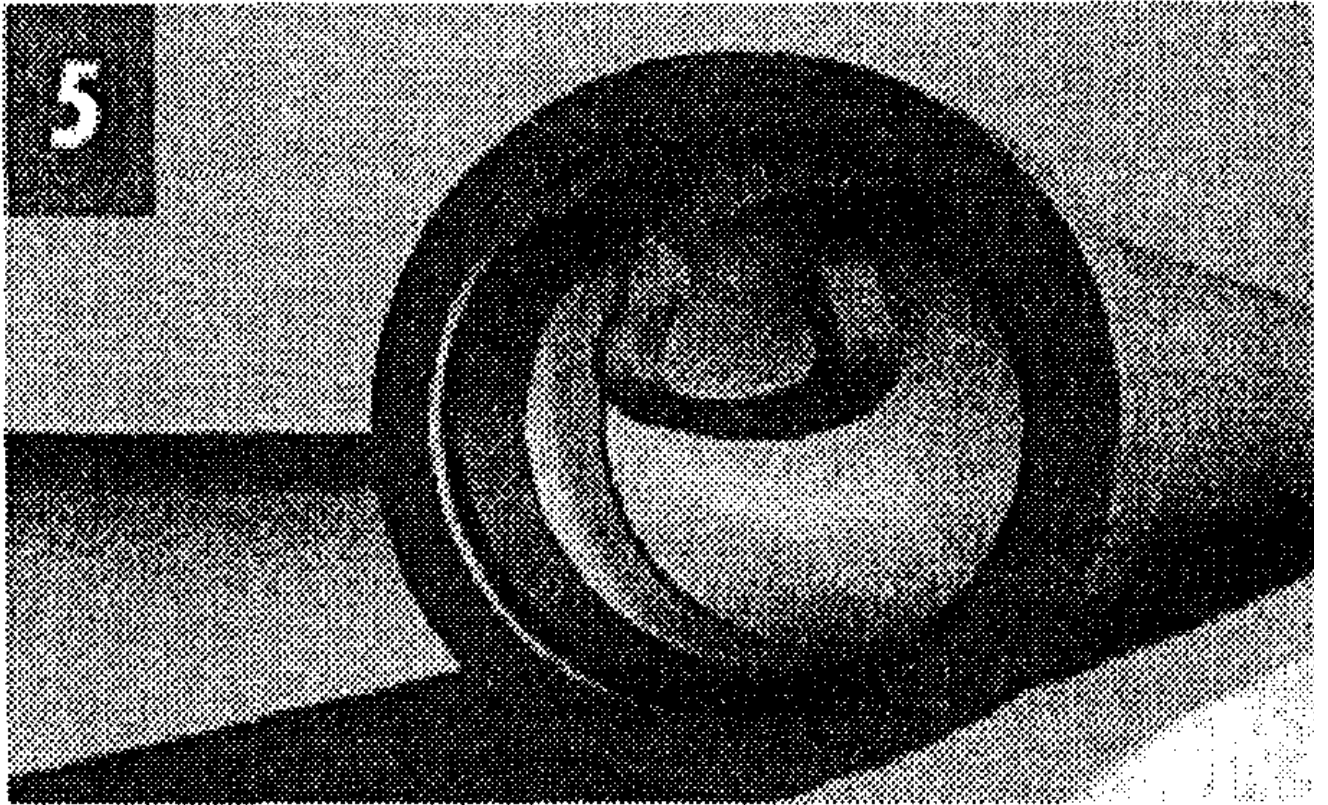
Установка уплотнительного резинового кольца в раструб
