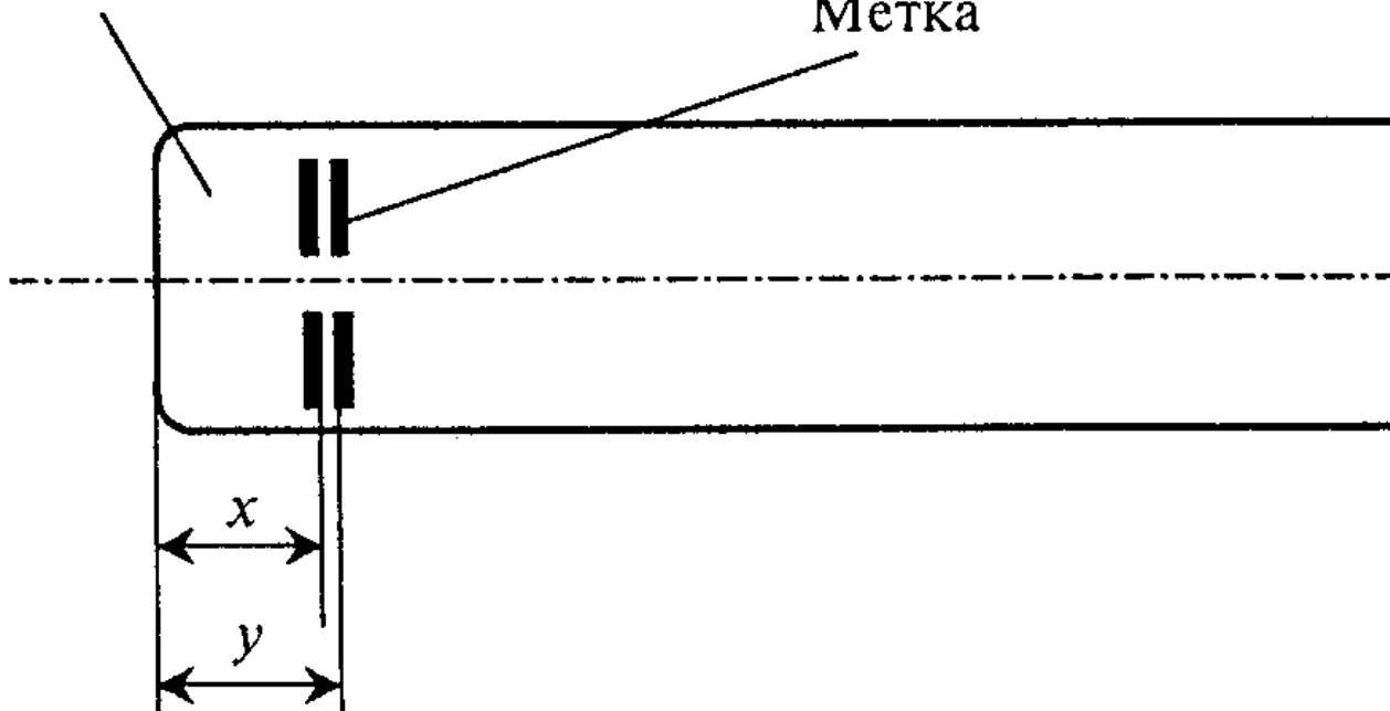
Рисунок 5.2. Метка на гладком конце трубы
