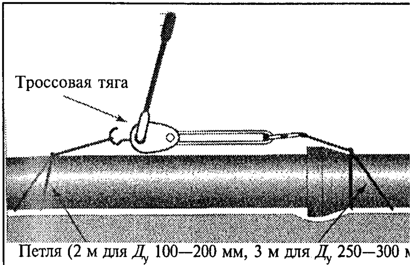
в - при помощи петли и тросовой тяги (для 100 - 300 мм)
