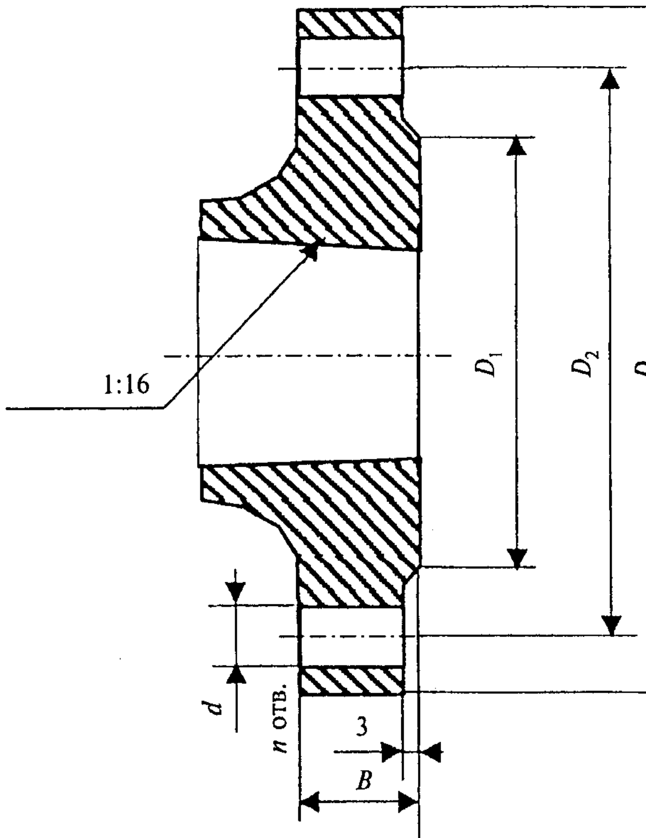
Рисунок А.10. Схема фланца из высокопрочного чугуна (тип Б)
