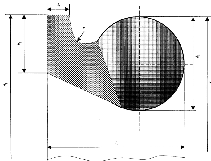
Рисунок А.13. Уплотнительное резиновое кольцо (под соединение "Тайтон")
