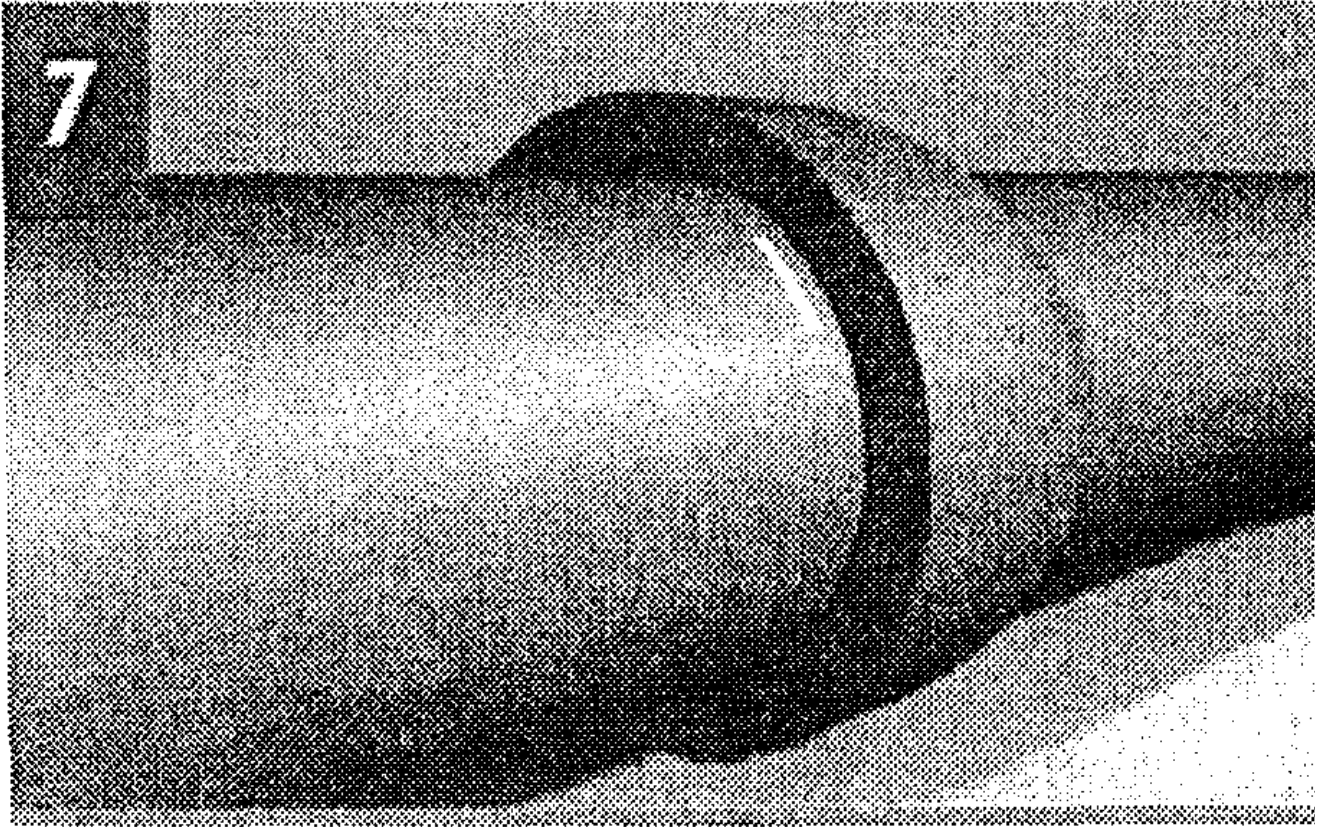
Смонтированное соединение Рисунок 5.5. Порядок монтажа труб под соединения "Универсал" и "Тайтон"
