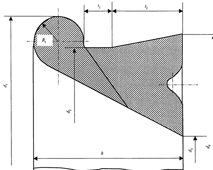
Рисунок А.14. Уплотнительное резиновое кольцо (под соединение "BPC")
