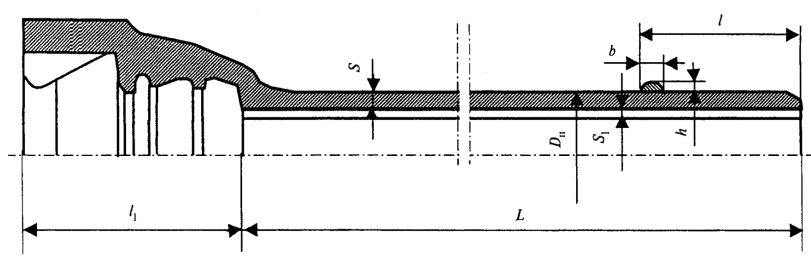
Рисунок А.2. Схема трубы раструбной под соединение "BPC"
