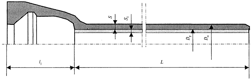
Рисунок А.3. Схема трубы раструбной под соединение "Универсал"
