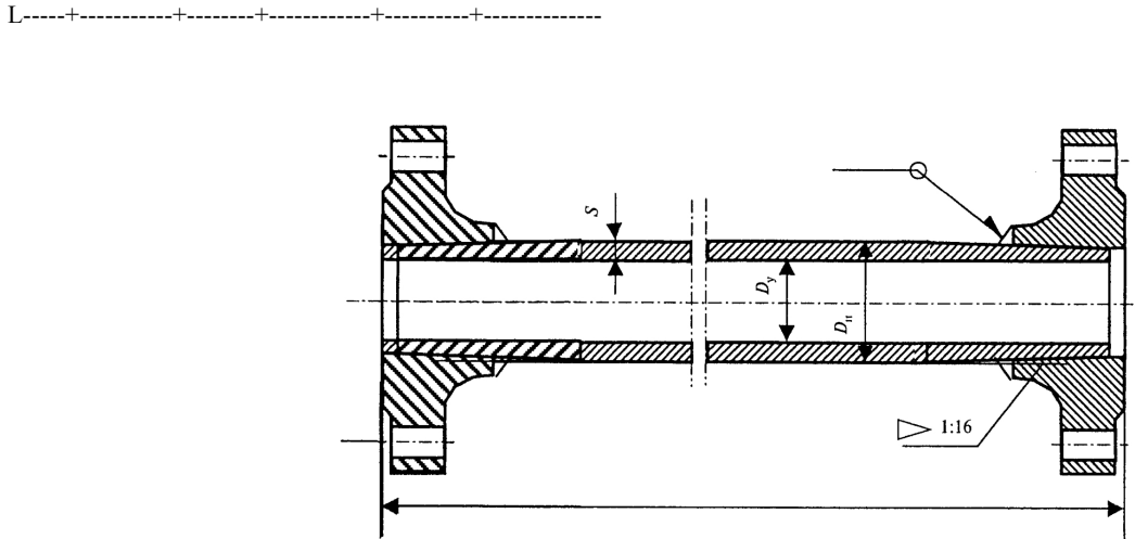
Рисунок А.8. Схема трубы с приваренными фланцами (тип Б)
