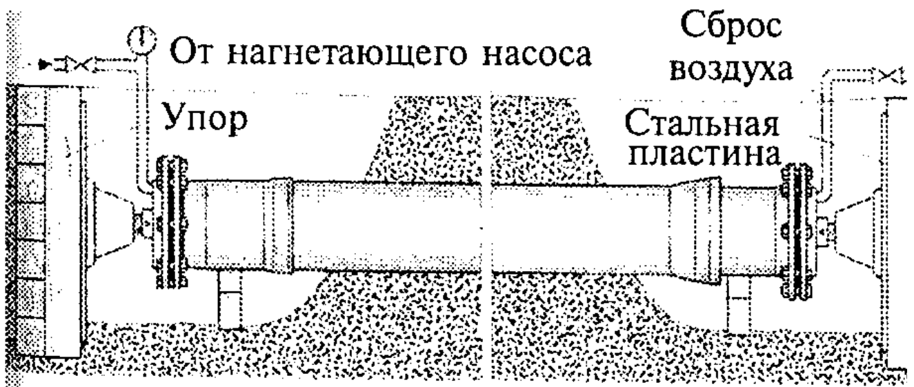
Рисунок 5.11. Подготовка трубопровода к гидрониспытанию
