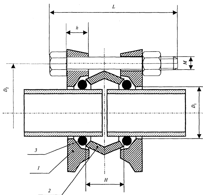
1 - фланец; 2 - втулка; 3 - резиновое кольцо
