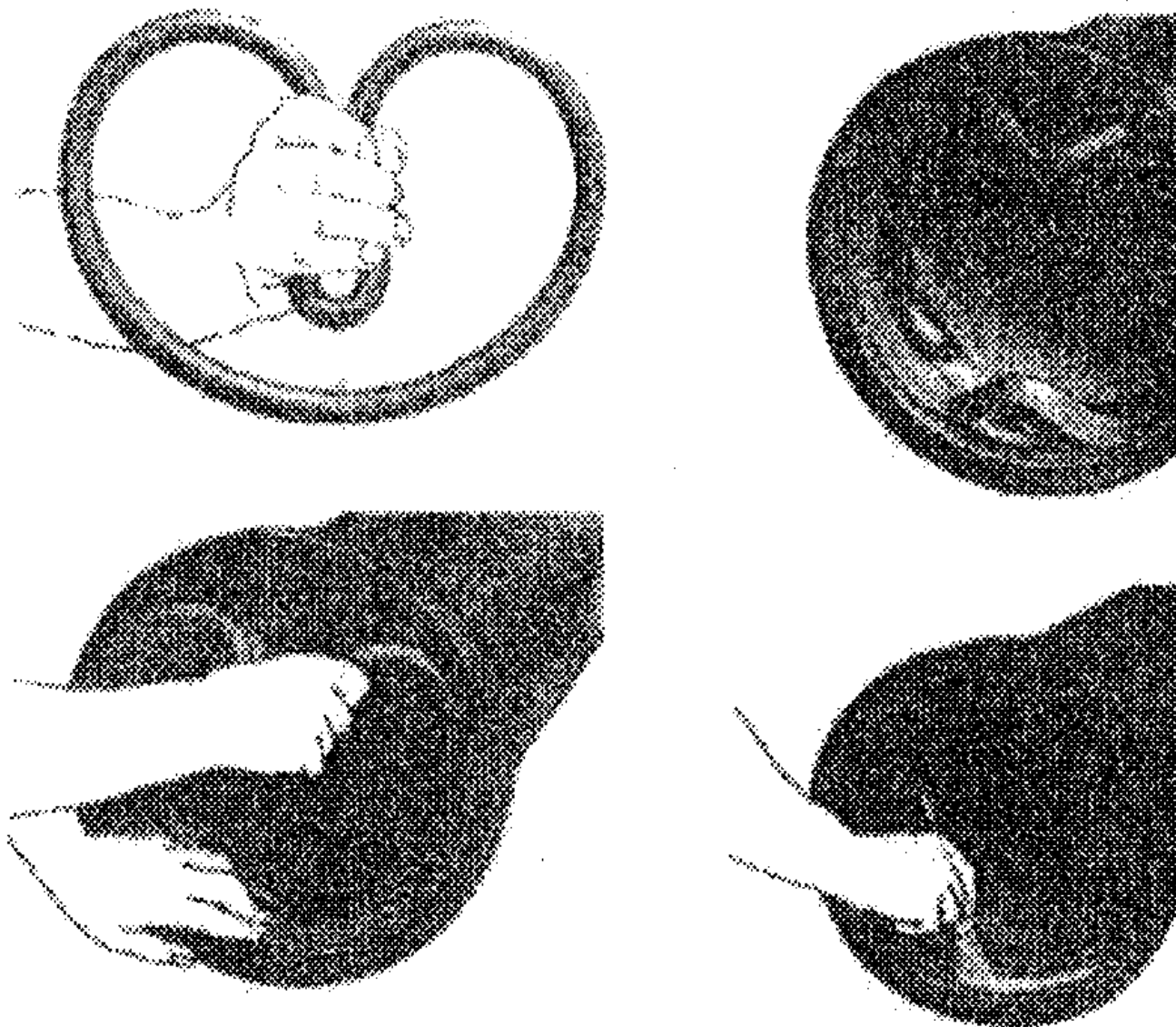
Рисунок 5.3. Схема укладки уплотнительного резинового кольца
