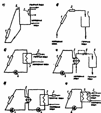
Принципиальные схемы установок солнечного горячего водоснабжения а) - с естественной циркуляцией; б) - одноконтурная; в) - двухконтурная; г) - двухконтурная с постоянной температурой воды; д) - трехконтурная; е) - с двумя змеевиками в баке-аккумуляторе 1 - солнечный коллектор; 2 - бак-аккумулятор; 3 - дублер нагрева воды; 4 - циркуляционный насос; 5 - теплообменник; 6 - регулятор температуры
