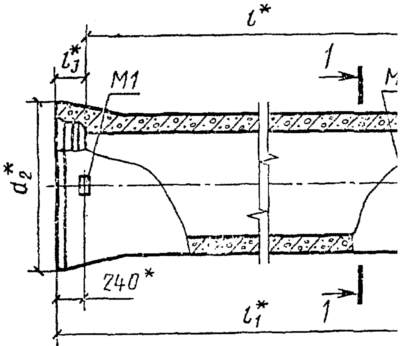
Продольный разрез стенки
