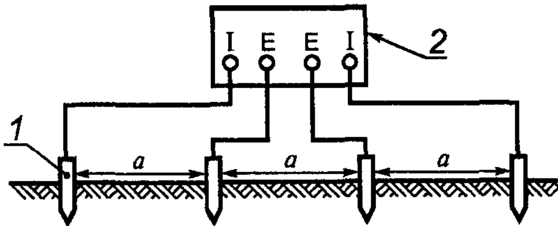
1 - электрод; 2 - прибор с клеммами: I - силы тока; E - напряжения; a - расстояние между электродами (см. формулу А.1) Рисунок А.1. Схема определения удельного сопротивления грунта
