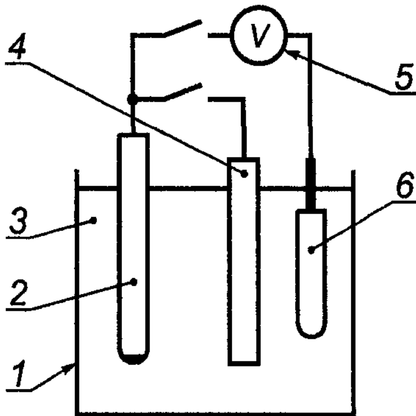
1 - емкость; 2 - испытуемый образец; 3 - электролит; 4 - магниевый анод; 5 - вольтметр; 6 - электрод сравнения Рисунок Л.1. Схема проведения испытания с применением магниевых анодов
