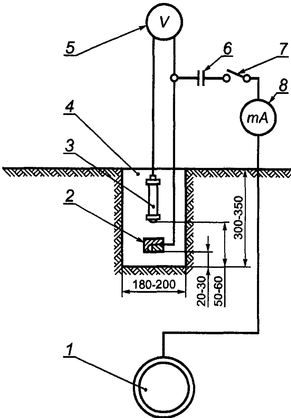
1 - трубопровод; 2 - датчик потенциала; 3 - переносной медно-сульфатный электрод сравнения; 4 - шурф; 5 - вольтметр; 6 - конденсатор; 7 - выключатель; 8 - миллиамперметр переменного тока Рисунок Ж.1. Схема измерений опасного влияния переменного тока на подземный стальной трубопровод
