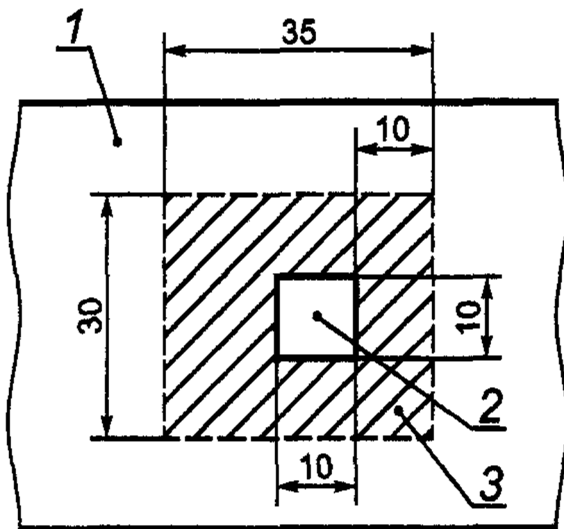
1 - испытуемое покрытие; 2 - образец покрытия для сдвига; 3 - площадь без покрытия Рисунок И.2. Схема проведения надреза для сдвига образца покрытия
