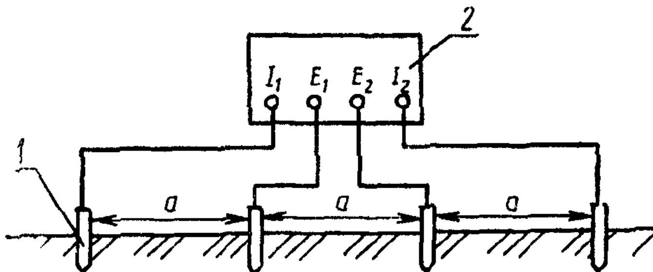
Схема определения удельного сопротивления грунта
