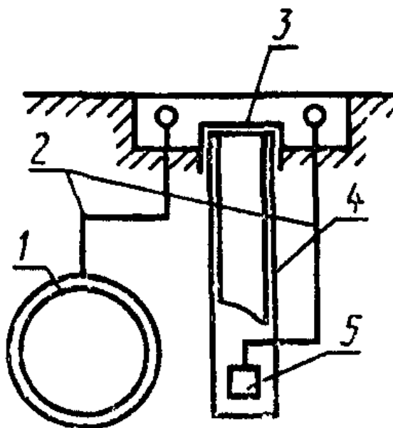
1 - трубопровод; 2 - контрольные проводники; 3 - заглушка; 4 - труба для установки переносного электрода сравнения; 5 - датчик потенциала
