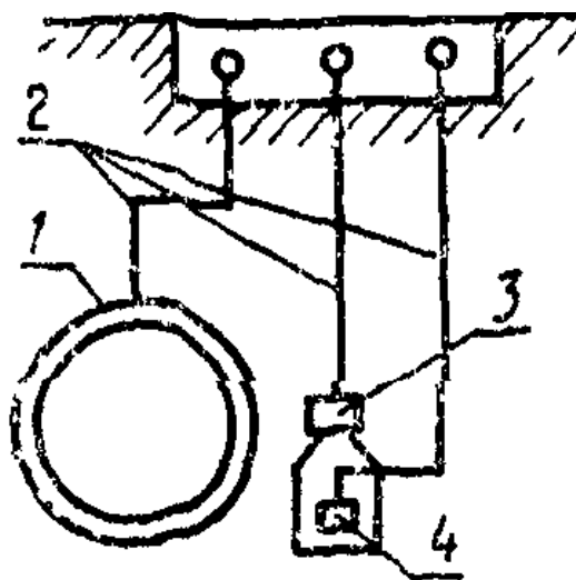
1 - трубопровод; 2 - контрольные проводники; 3 - медносульфатный электрод; 4 - датчик потенциала
