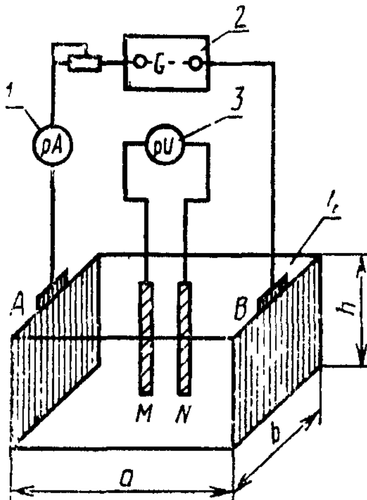
1 - миллиамперметр; 2 - источник тока; 3 - вольтметр; 4 - измерительная ячейка; А, В - внешние электроды; М, N - внутренние электроды (в ред. Изменения N 1, введенного в действие Постановлением Госстандарта РФ от 22.12.1994 N 342)
