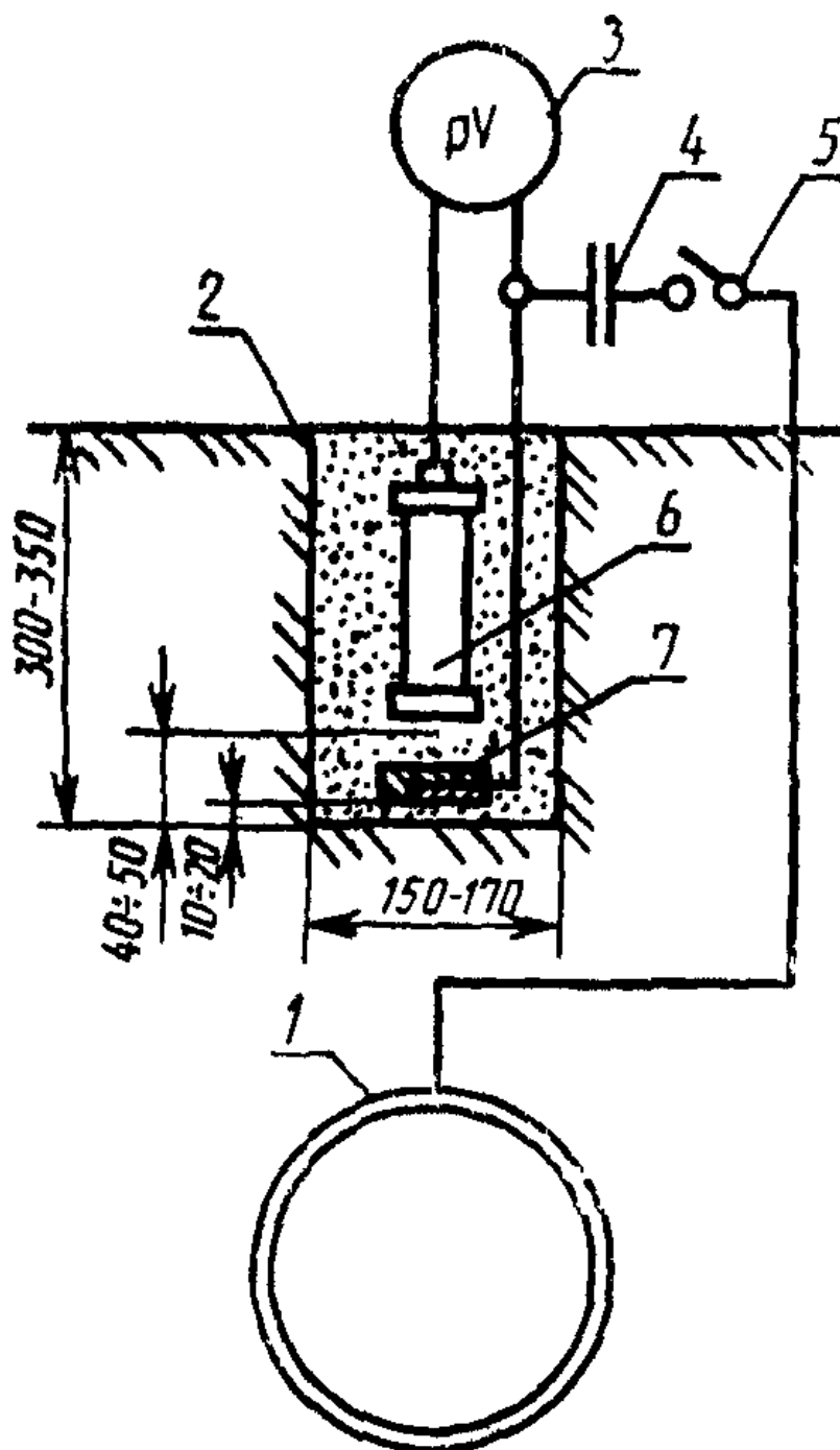
Схема измерений смещения потенциала трубопровода
