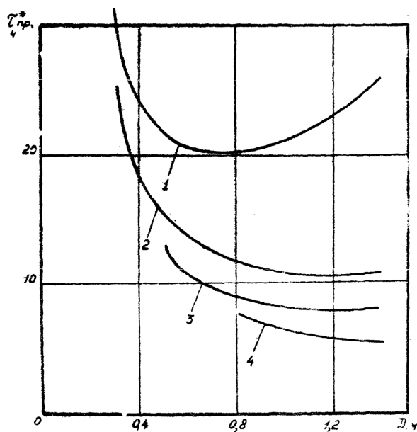
Рис. 1. Зависимость времени прокачки воды с температурой
