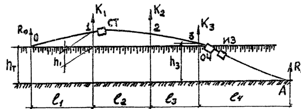
Расчетно-технологическая схема
