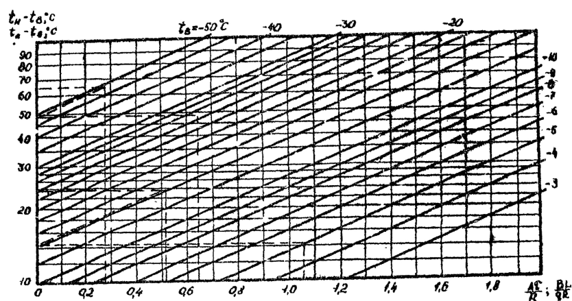
Рис. 1. Номограмма для определения начальной температуры воды в трубопроводе
