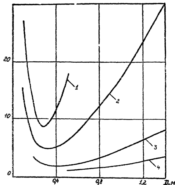
Рис. 2. Зависимость времени прокачки воды с температурой
