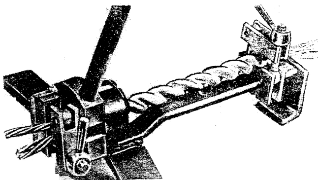
Рис. 4. Приспособление типа МИ-189А для соединения проводов в овальных соединителях методом скрутки
