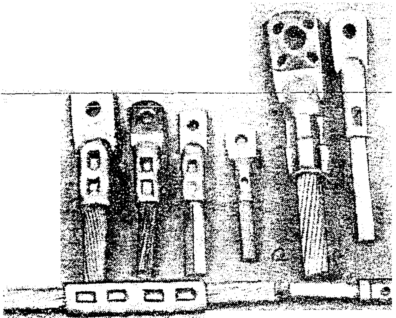
Рис. 27. Образцы оконцевания алюминиевых жил кабелей, выполненные способом опрессовки:
