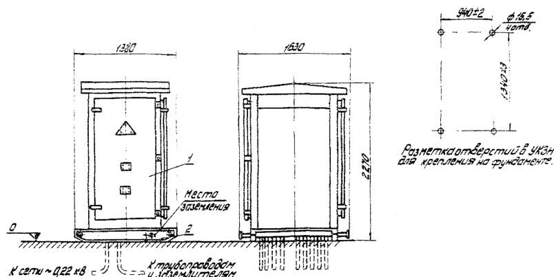
Рис. 1. Общий вид смонтированного устройства катодной защиты низковольтного УКЗН:
