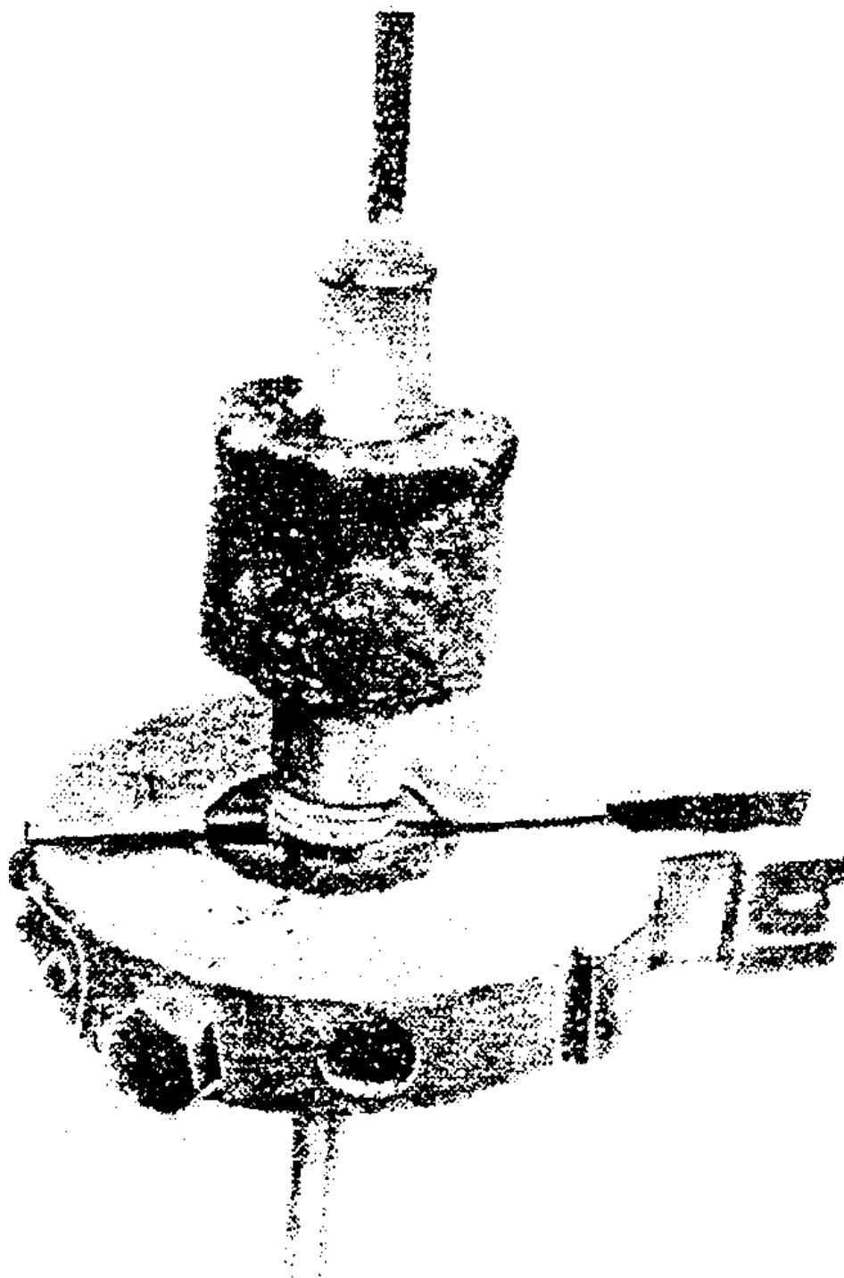
Рис. 18. Введение стального стержня в кокиль термитного патрона с расплавленным алюминием
