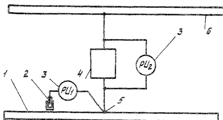
Рис. 33. Схема включения измерительных приборов при пусконаладочных работах на электродренажных установках:
