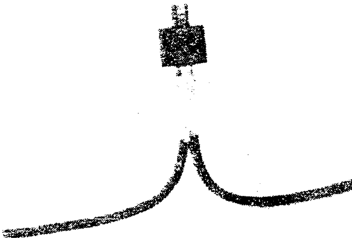
Рис. 11. Подготовленные к сварке жилы кабеля с термитным патроном марки АС
