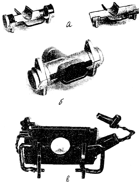
Рис. 22. Сварочные полуформы:
