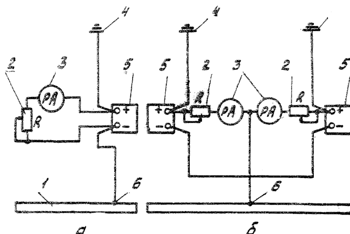
Рис. 32. Схема включения приборов и устройств при испытании преобразователей катодной защиты в режиме максимальной нагрузки:
