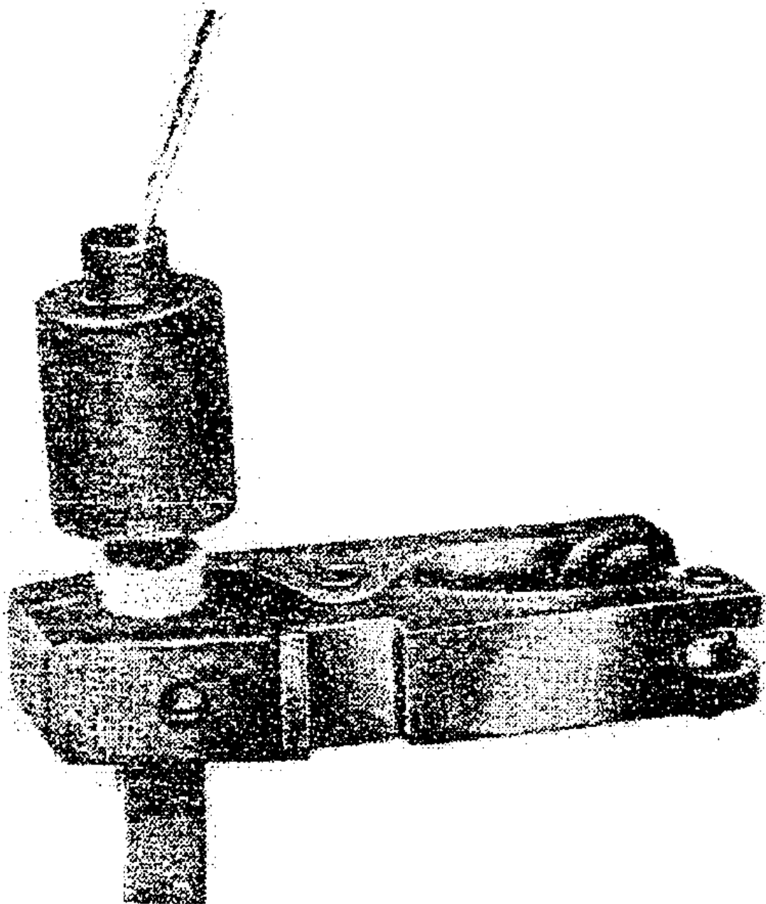
Рис. 17. Введение присадочного прутка из алюминиевой проволоки в кокиль термитного патрона марки АС при сварке алюминиевой жилы кабеля со стальным стержнем
