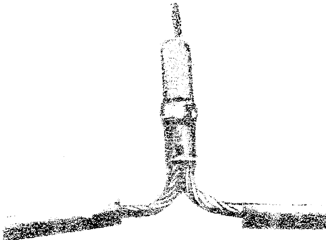
Рис. 14. Образец контактного соединения проводов марки ПСРП с алюминиевыми жилами кабеля
