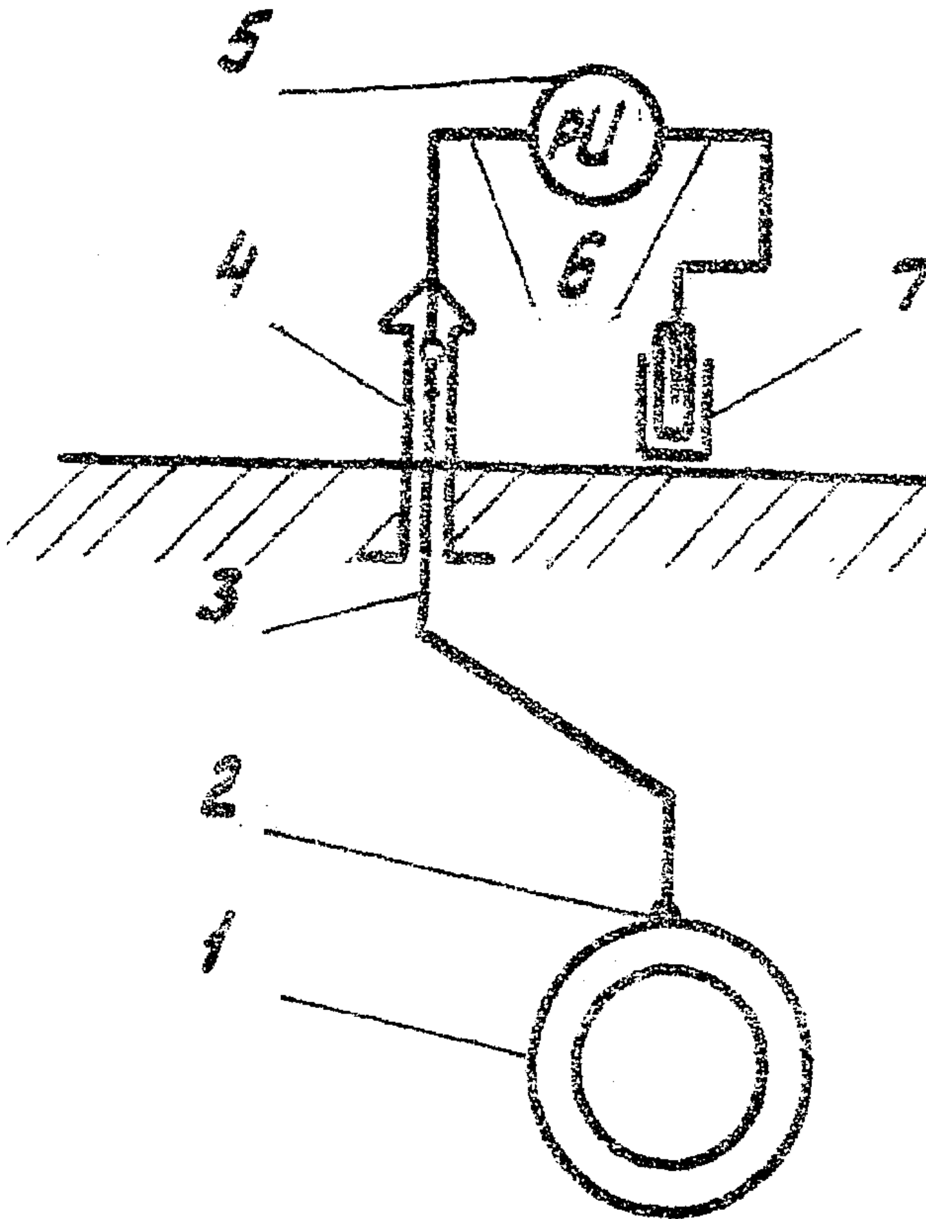
Рис. 31. Схема измерений разности потенциалов "труба - земля":
