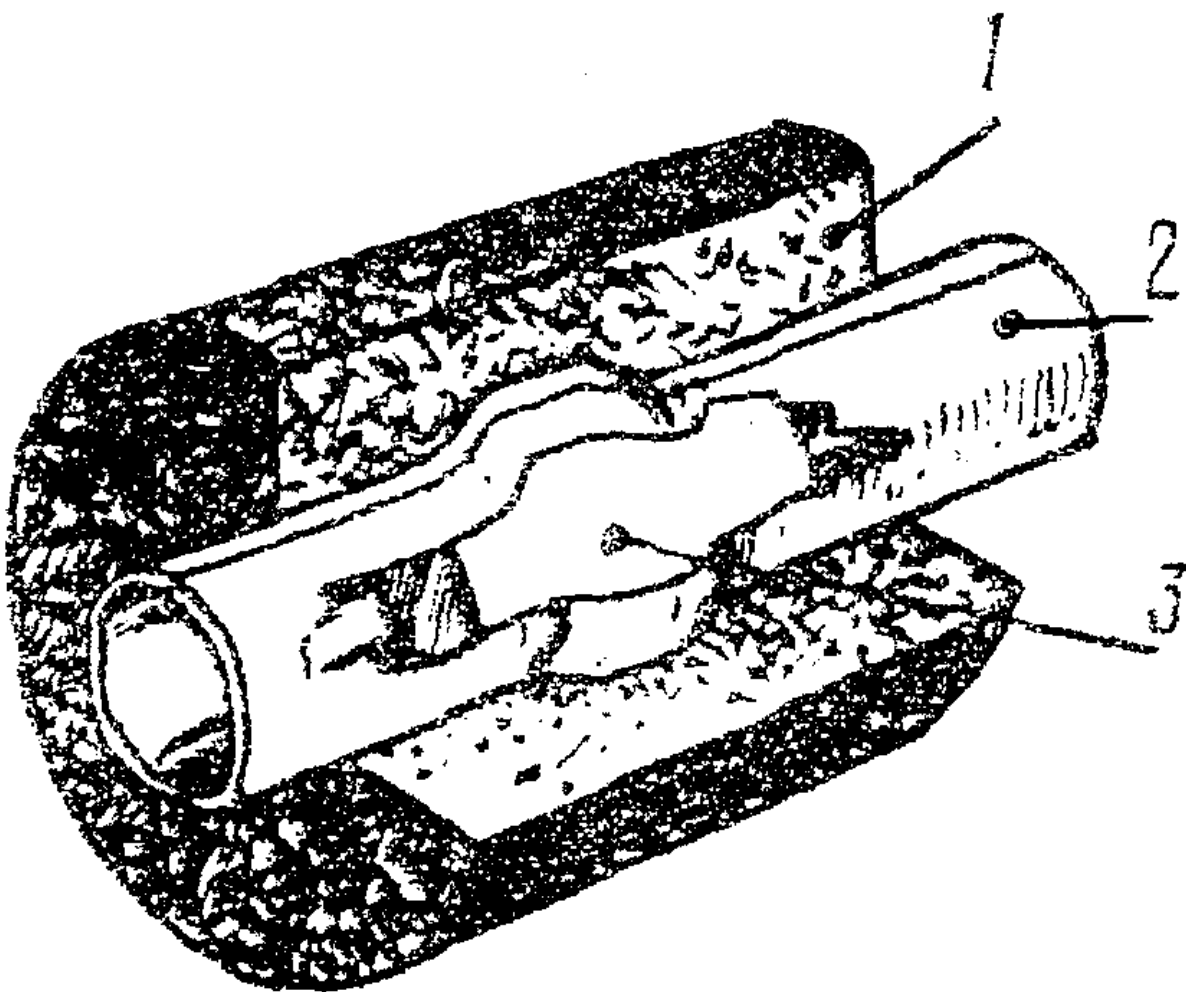
Рис. 9. Термитный патрон марки АС для сварки жил проводов и кабелей:
