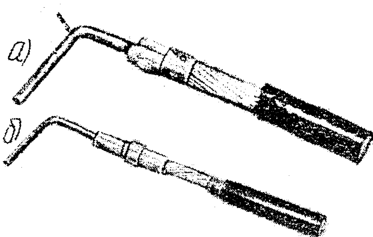
Рис. 19. Образцы контактных соединений стальных стержней с алюминиевыми жилами кабеля:
