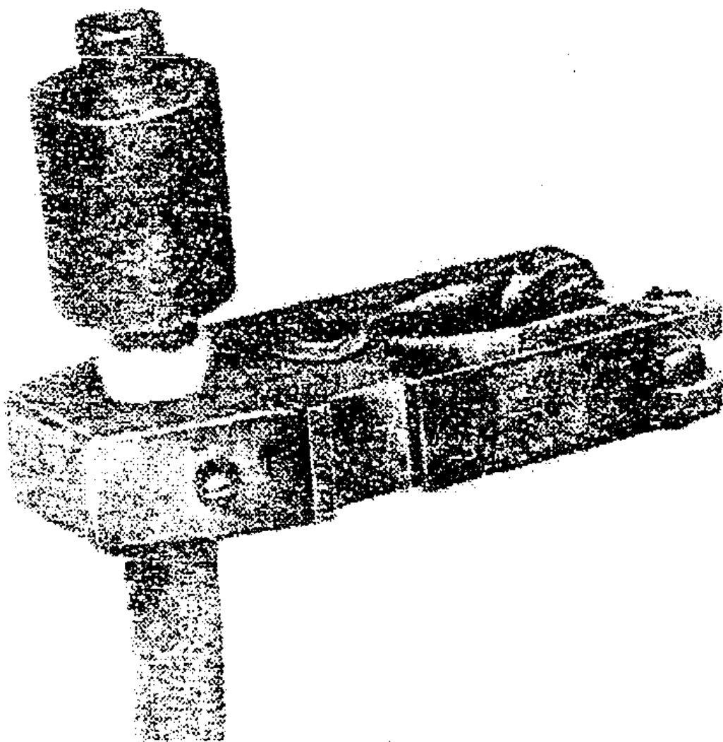
Рис. 16. Патрон марки АС с охладителем, установленный для сварки алюминиевой жилы кабеля со стальным стержнем
