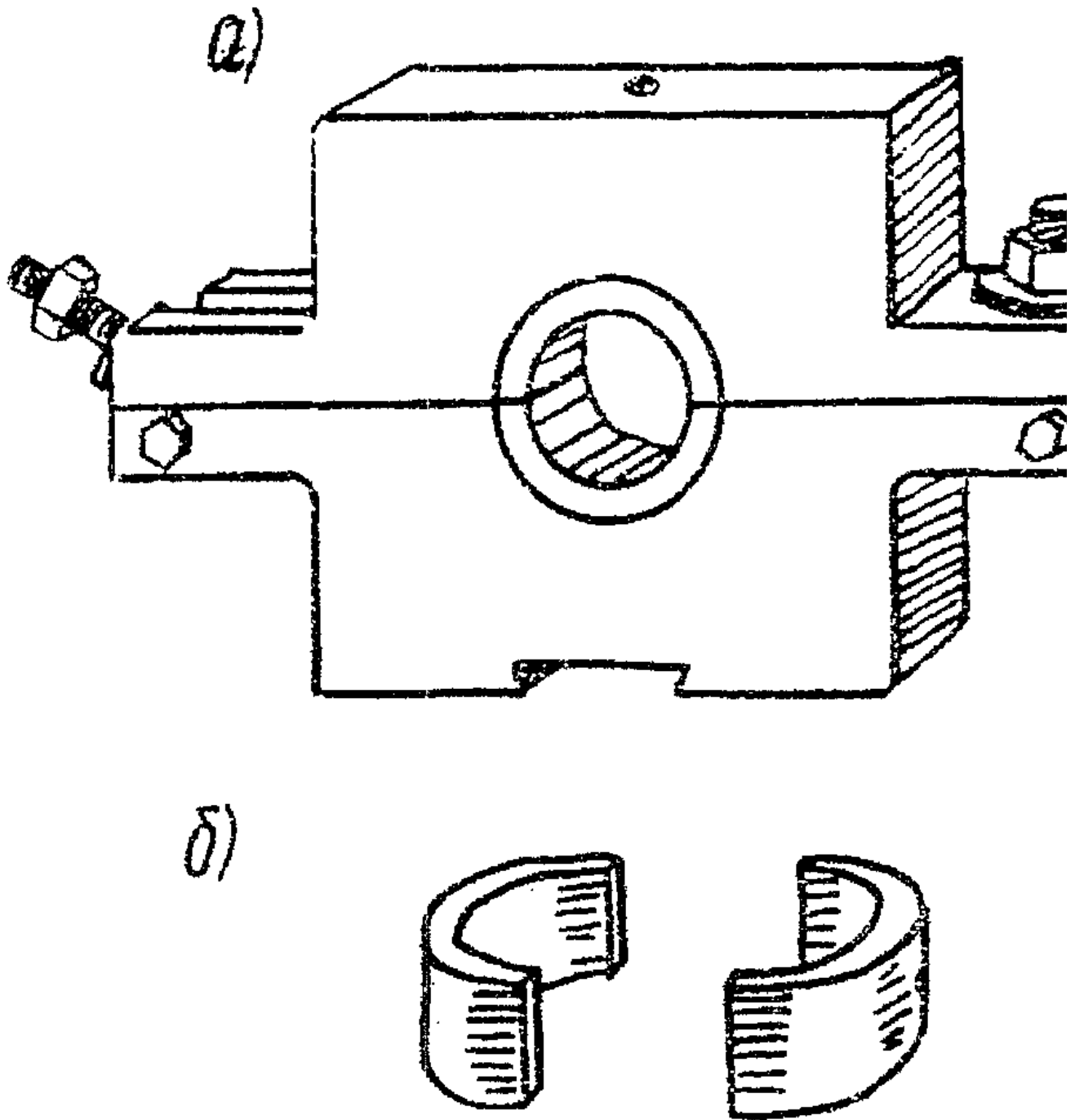
Рис. 23. Охладитель со сменными вкладышами:
