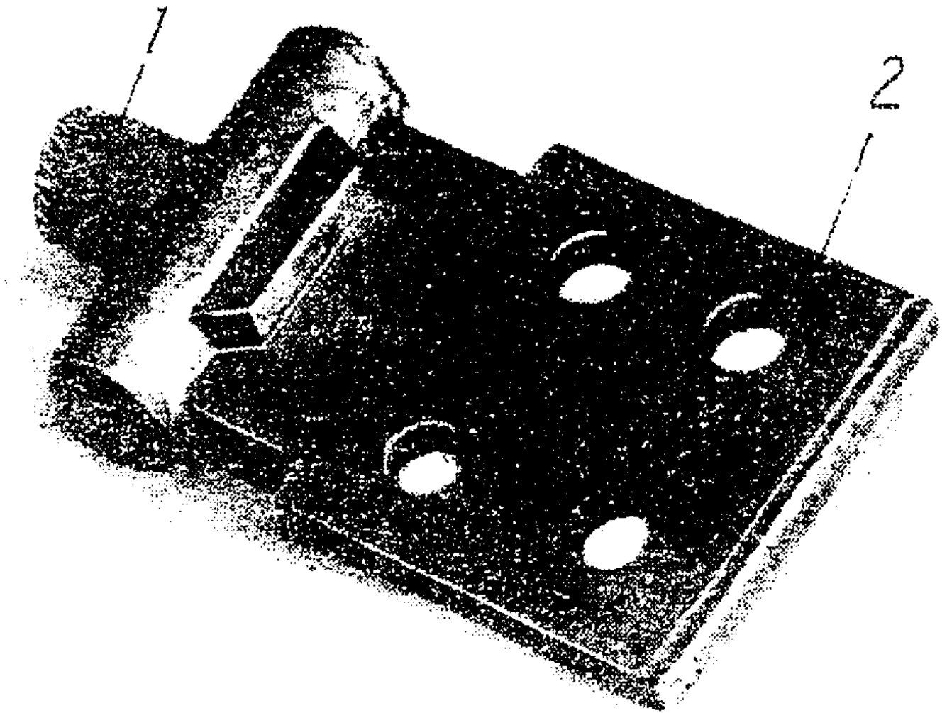
Рис. 25. Оконцованный алюминиевый кабель с применением полуформ, изготовленных на базе набора НГО:
