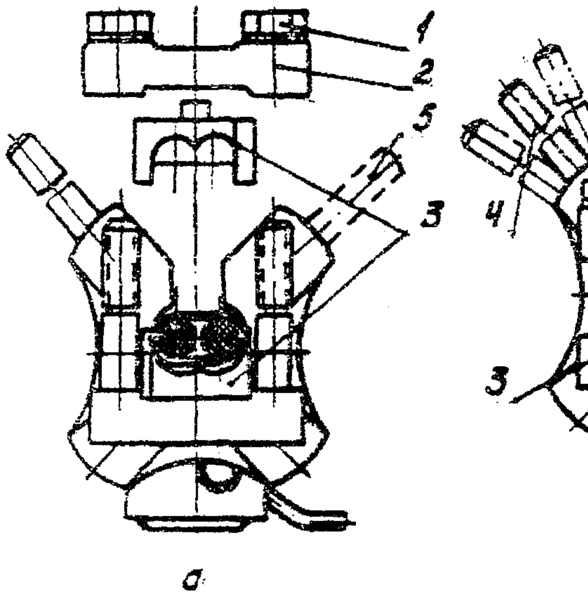
Рис. 7. Зажимные узлы приспособления МИ-230А:
