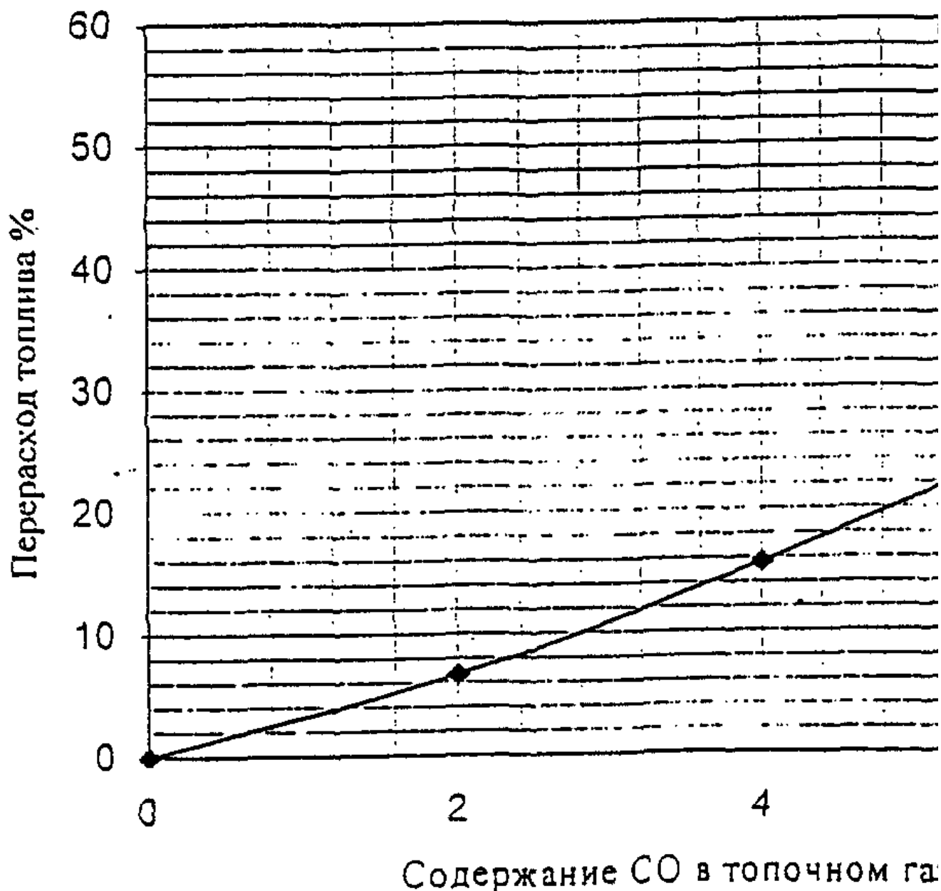
Рис. 15. Влияние содержания СО (химический недожег) в топочном газе на перерасход топлива (газ, нефть)
