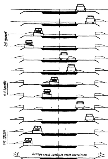
Рисунок 15. Схема проходов снегоочистителей при расчистке дороги, занесенной толстым слоем снега (при отсутствии
