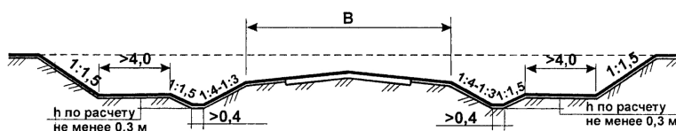
Рисунок 1. Выемки: а - раскрытая; б - разделанная под насыпь; в - с полками
