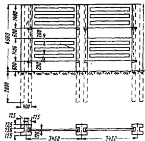
Рисунок 6. Железобетонный снегозадерживающий забор
