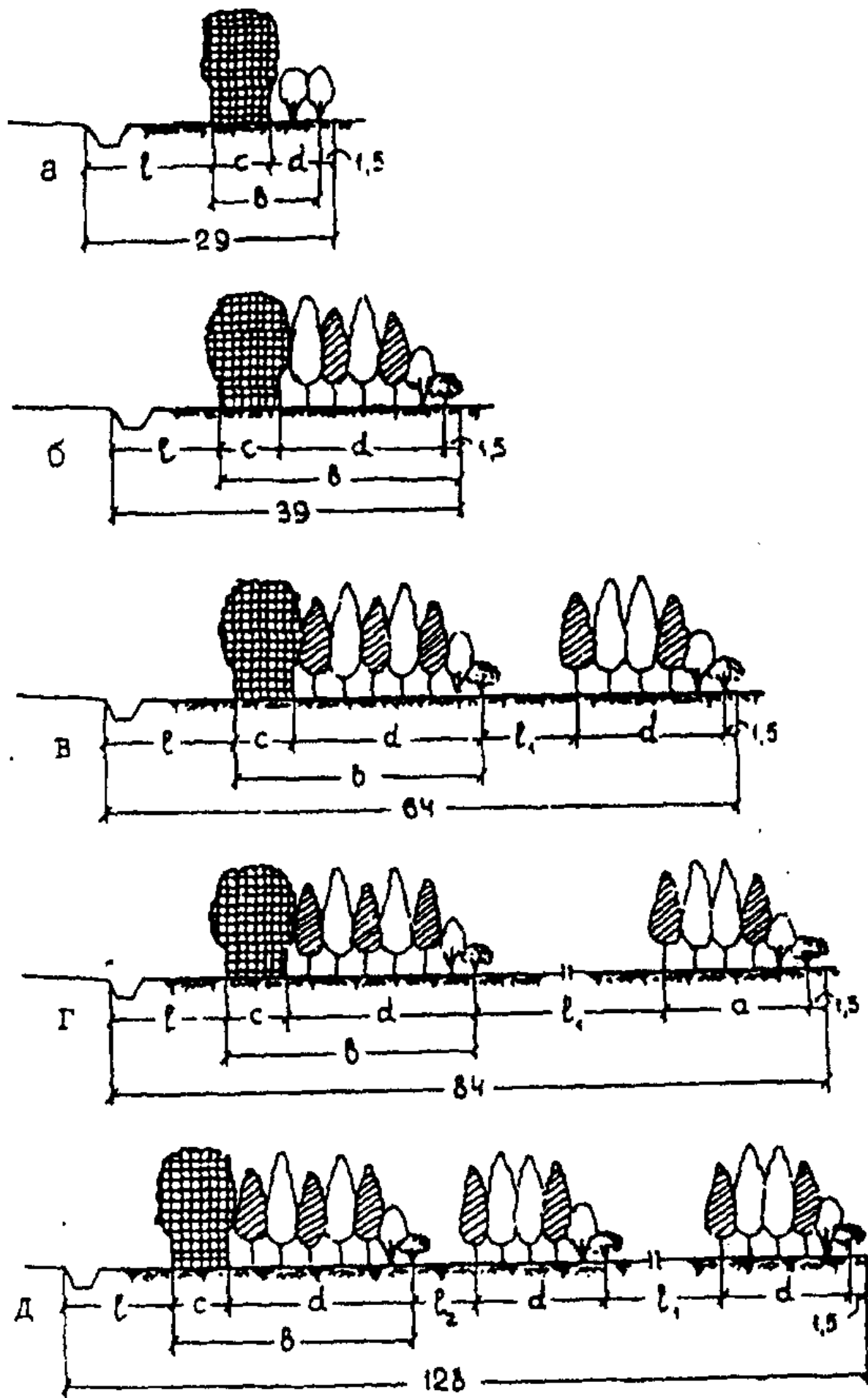
Рисунок 4. Типовые схемы усиления существующих снегозащитных лесных насаждений вдоль автомобильных дорог при объеме снегоприноса (м 3 /м): а - до 25; б - до 50; в - до 100; г - до 150; д - до 250
