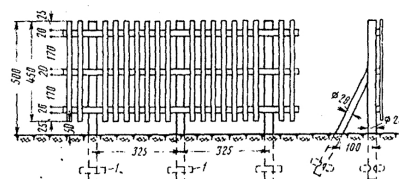
Рисунок 5. Рекомендуемые типы снегозадерживающих заборов: I - противупучинные анкеры (брусек 10 х 14 см или пластины длиной 50 см)
