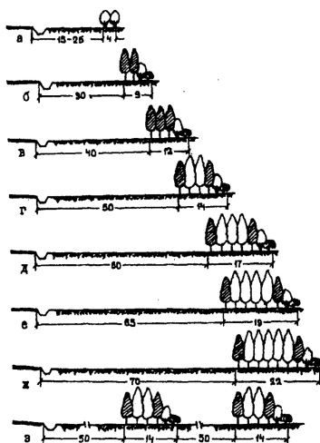
Рисунок 2. Типовые схемы снегозащитных лесных насаждений вдоль автомобильных дорог при объеме снегопереноса (м 3 /м).
