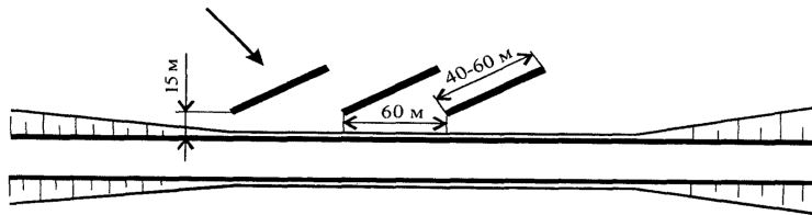
Рисунок 10. Косые звенья щитов
