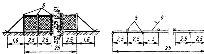
Рисунок 13. Снегозадерживающие полиэтиленовые сетки: а - тип I на стойках металлических труб; б - тип II на деревянных кольях; в - размещение кольев; 1 - стопорная шайба 15 x 150 x 5 с отверстием 33 мм; 2 - упор; 3 - крепление для сетки 5 мм; 4 - стальная труба 33 - 24 мм; 5 - деревянные колья 80 - 100 мм; 6 - сетка
