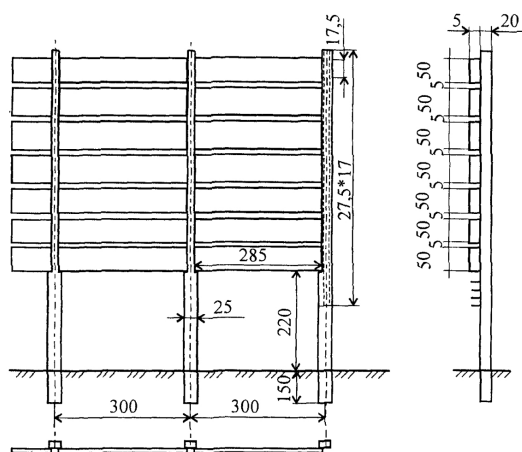
Рисунок 8. Снегопередающий керамзитобетонный забор
