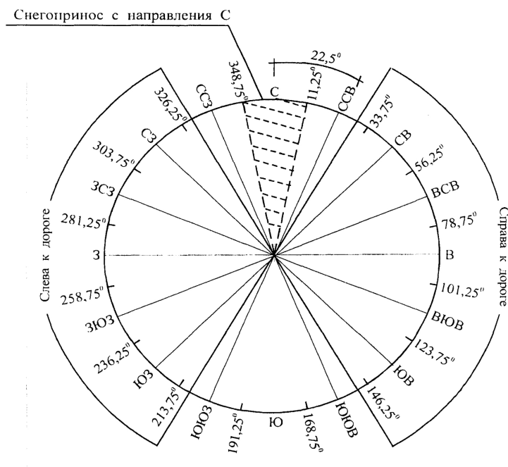
Рисунок Б.1. Схема расчета объемов снегоприноса к дороге, направленной на север.
