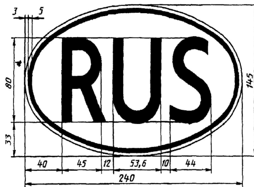
Рисунок 1. Отличительный знак типа 1
