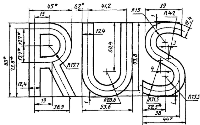
Рисунок 3. Размеры букв отличительного знака типа 1
