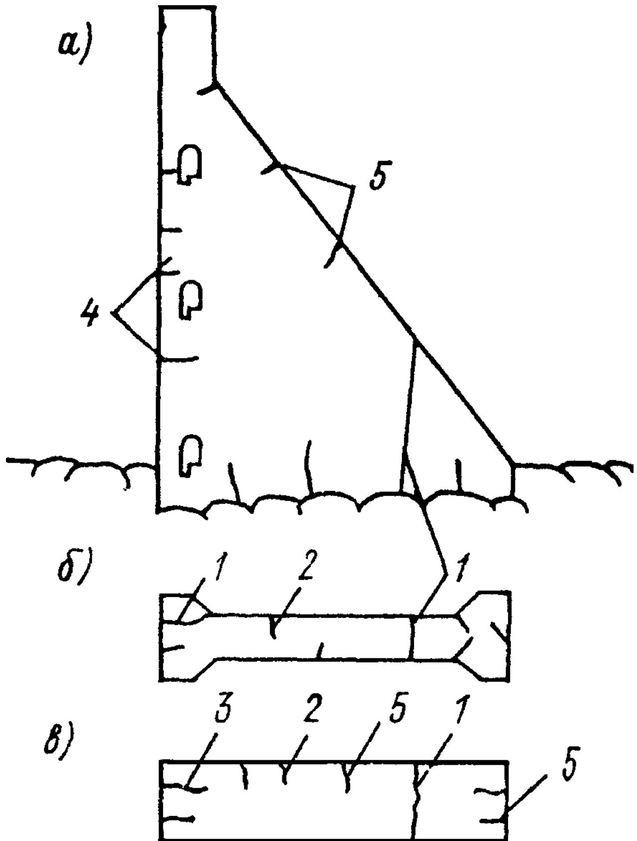
Рис. 1. Схема трещин в бетонной плотине: а - отдельная секция; б - план секции; в - план секции; 1 - трещины вертикальные, продольные, поперечные сквозные; 2 - 3 - трещины глубокие вертикальные и горизонтальные несквозные со стороны напорной грани; 4 - 5 - трещины, выходящие на низовую грань
