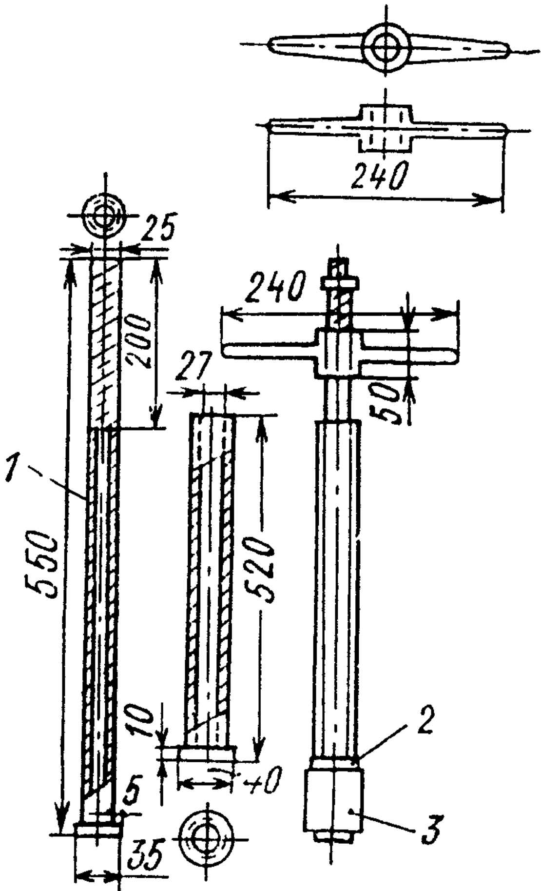
Рис. 3. Тампон-нагнетатель: 1 - иньектор; 2 - запlechник; 3 - резиновый уплотнитель
