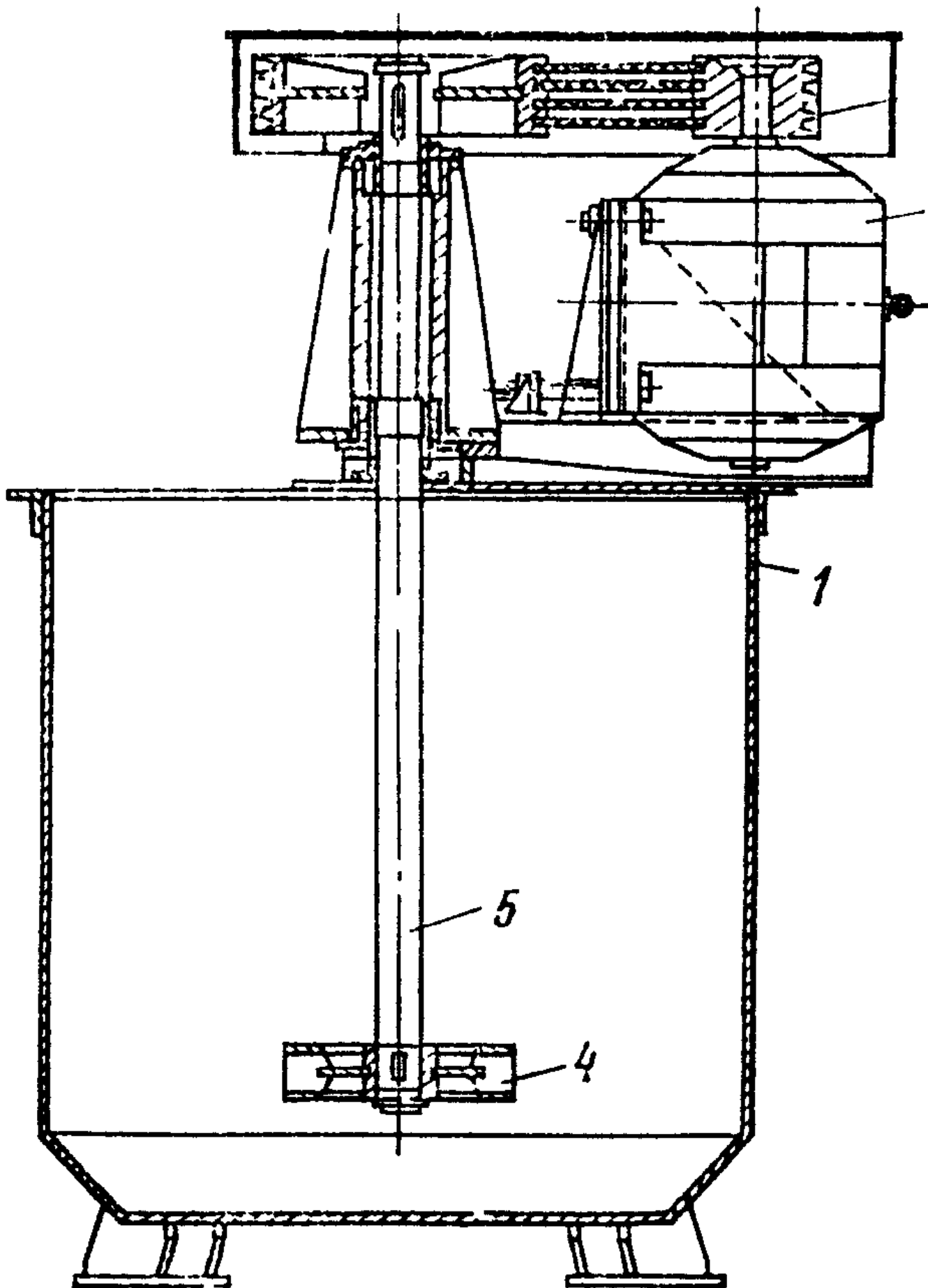
Рис. 2. Растворосмеситель РМ: 1 - корпус смесителя; 2 - электромотор; 3 - шкив; 4 - турбина; 5 - вал
