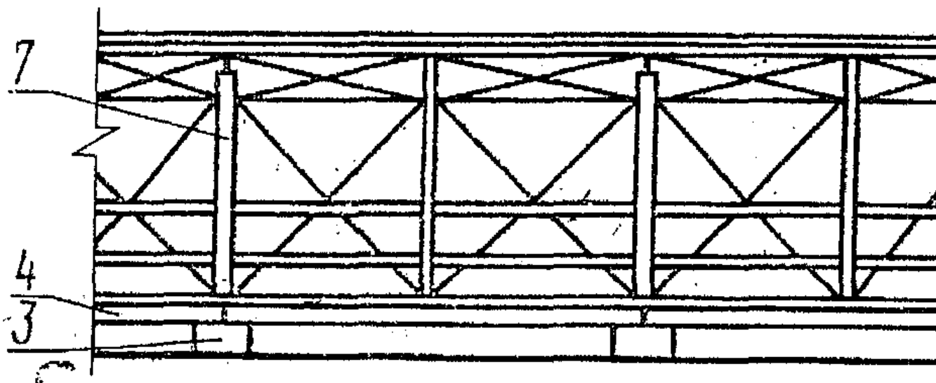
Черт. 2. 1 - панель ограждения; 2 - подкос панели; 3 - опора (лежень); 4 - панель тротуара; 5 - горизонтальный элемент перил; 6 - поручень; 7 - стойка перил; 8 - панель козырька; 9 - подкос козырька; 10 - стойка ограждения; 11 - пеньковый или капроновый канат, проволока
