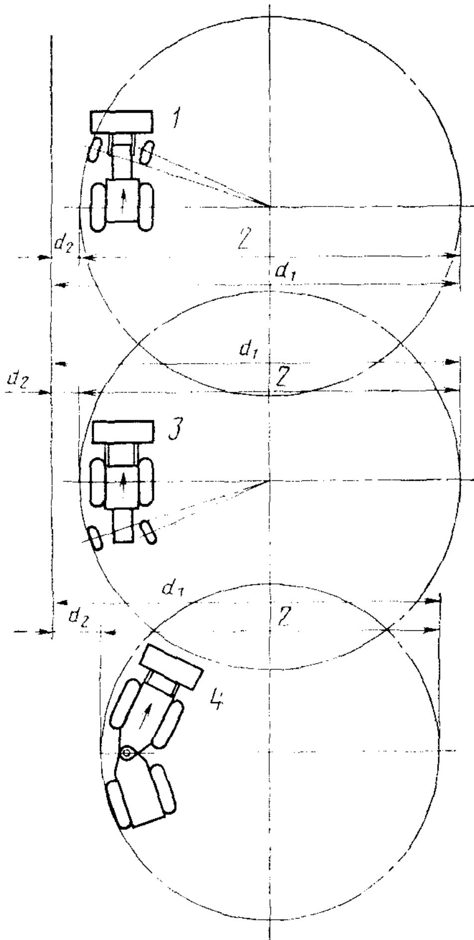
1 - погрузчик с передними управляемыми колесами; 2 - ширина полосы безостановочного разворота (); 3 - погрузчик с задними управляемыми колесами; 4 - шарнирно-сочлененный погрузчик (и погрузчик с четырьмя управляемыми колесами)
