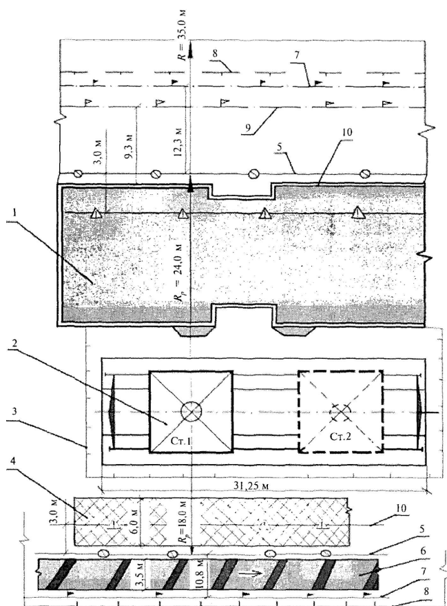
Рисунок 2. Стройгенплан с зонами, образующимися при работе башенного крана (фрагмент)
