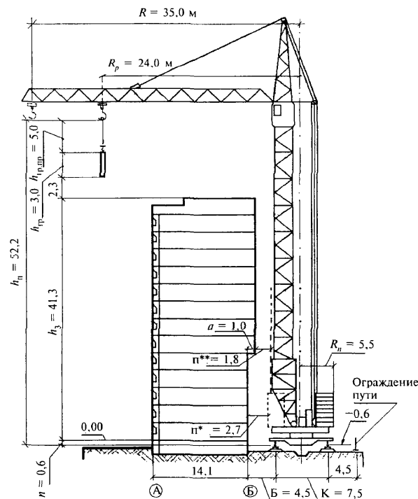
Рисунок 1. Привязка башенного крана к зданию
