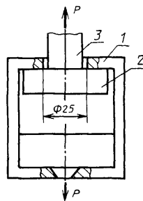
1 - захват образца; 2 - образец; 3 - металлический цилиндр
