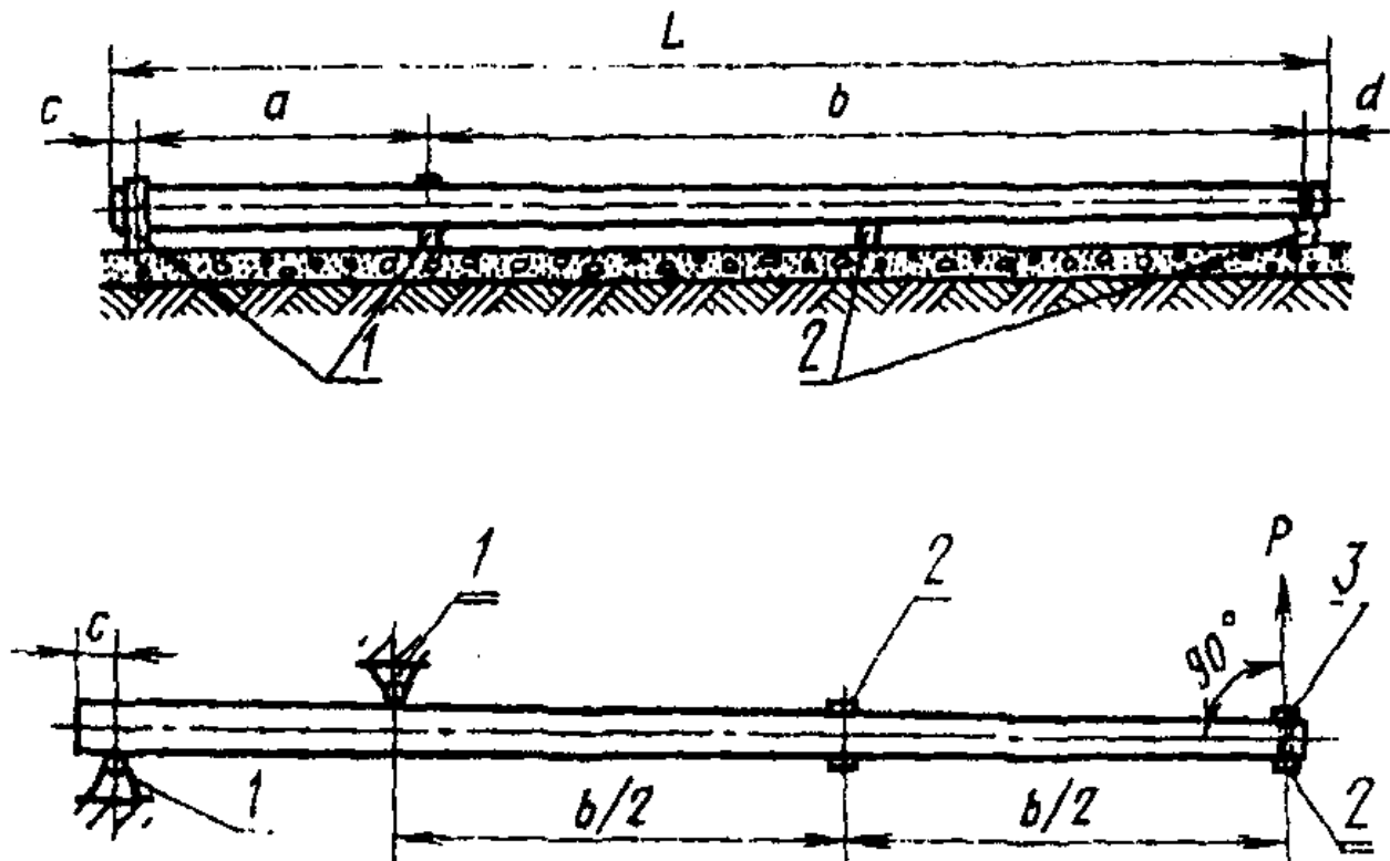
Схема испытания стоек
