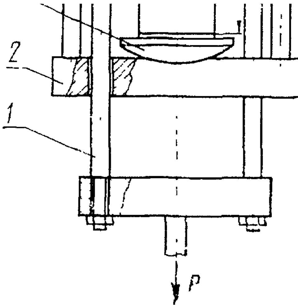
1 - нижняя траверса реверсора; 2 - верхняя траверса реверсора; 3 - шарнирная опора; 4 - образец; 5 - индикатор часового типа; 6 - упорный шток Черт. 1
