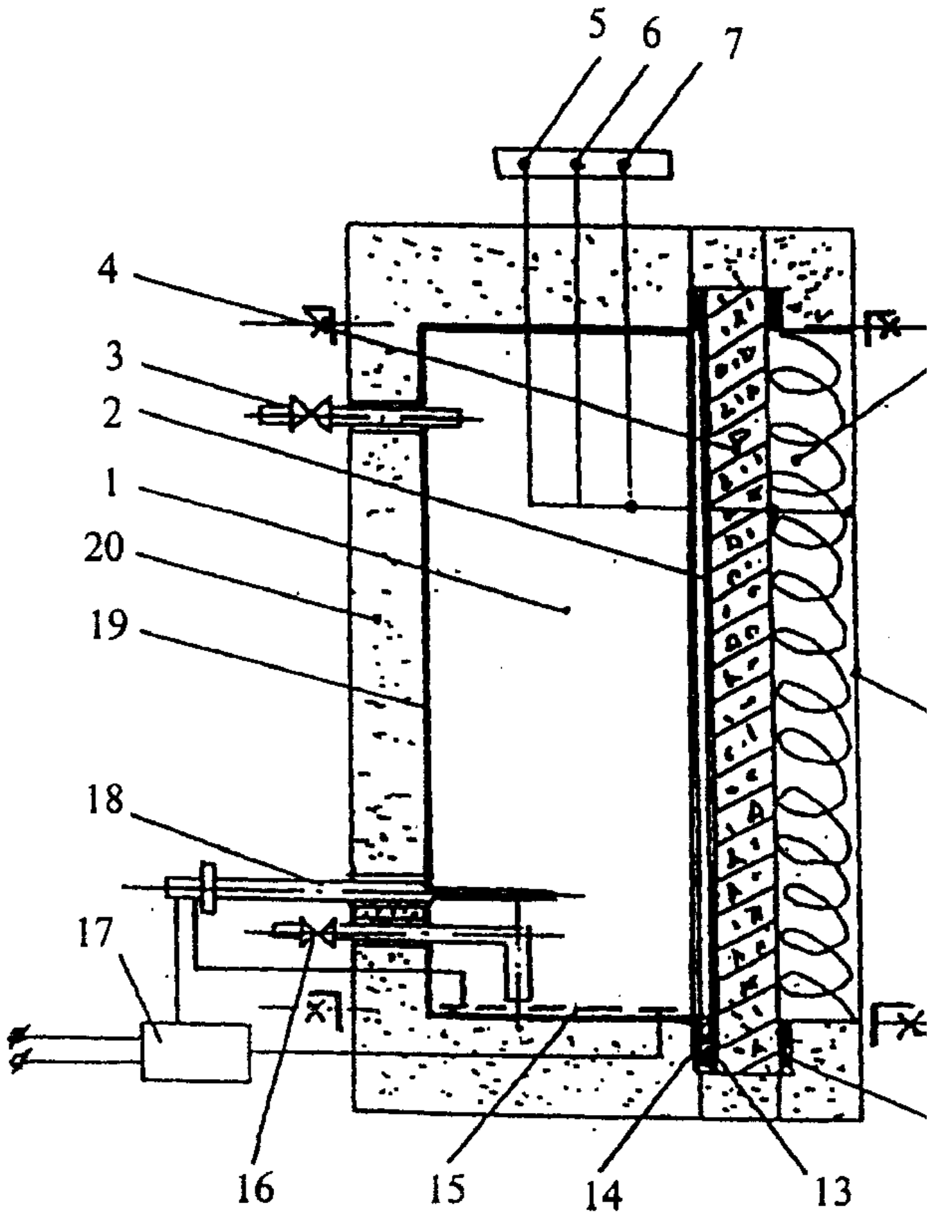
1 - испытательная камера; 2 - диафрагма; 3 - патрубок (штуцер) для отбора проб; 4 - железобетонная плита; 5 - 7, 18 - датчики температуры; 8 - теплоизоляционный слой модели; 9 - источник инфракрасного излучения; 10 - покрывающий короб; 11 - болтовые стяжки; 12 - фланец и резиновая прокладка покрывающего короба; 13 - резиновый уплотнитель камеры; 14 - фланец испытательной камеры; 15 - плоский электронагреватель; 16 - входной патрубок (штуцер); 17 - блок регулирования нагрева испытательной камеры; 19 - корпус испытательной камеры; 20 - тепловая изоляция камеры
