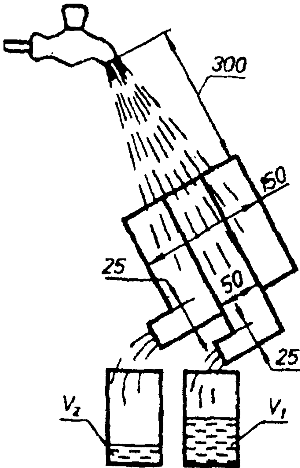
Рисунок 1. Схема определения компактности струи
