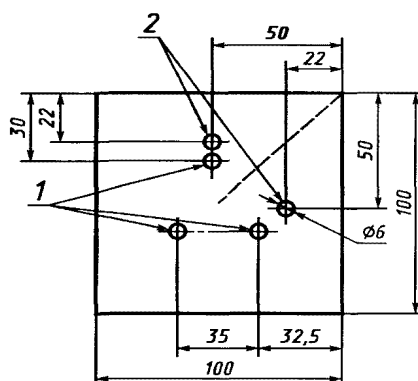
1 - опорные штифты; 2 - установочные штифты Рисунок А.2. Подставка для образцов
