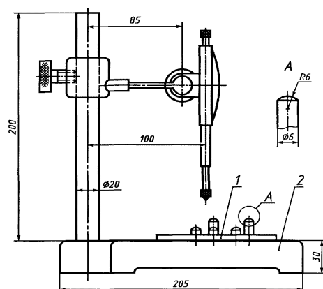
1 - подставка; 2 - опорная плита Рисунок А.1. Устройство для измерения длины
