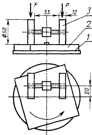
Схема прибора для определения стойкости покрытий к истиранию
