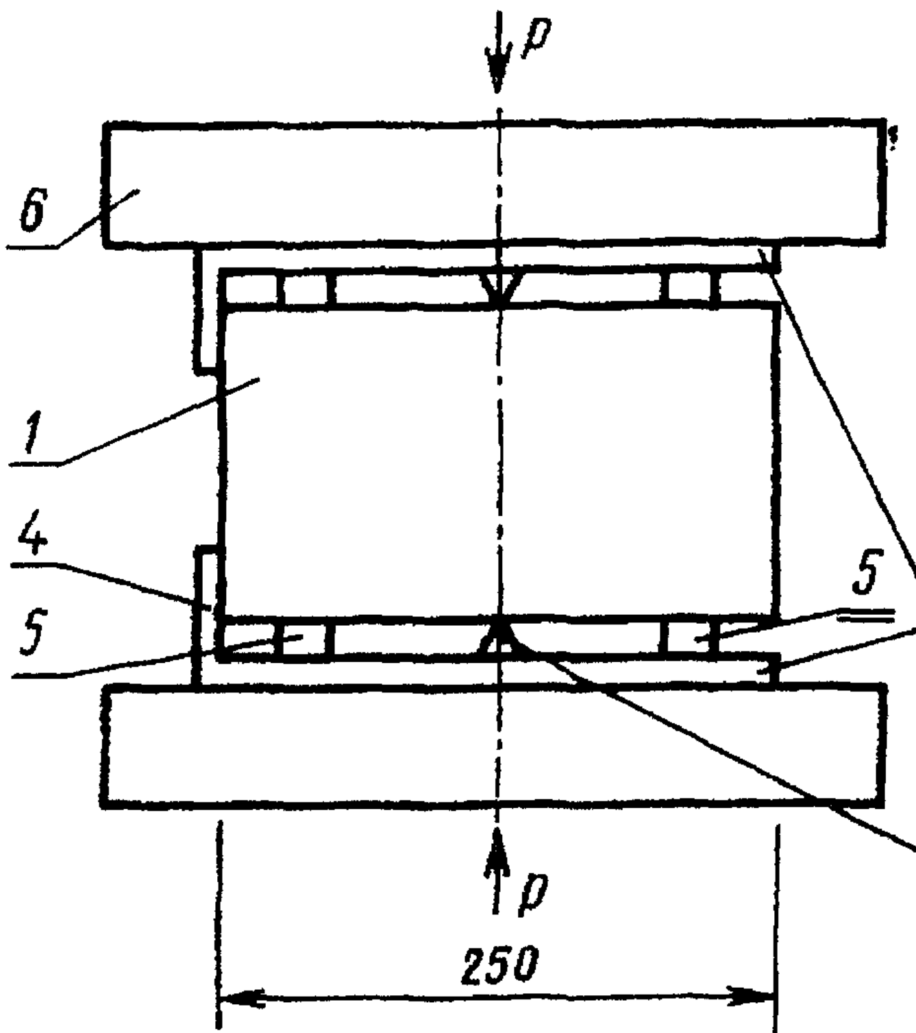
1 - образец; 2 - основание; 3 - металлический нож; 4 - упор; 5 - резиновые прокладки; 6 - плита пресса
