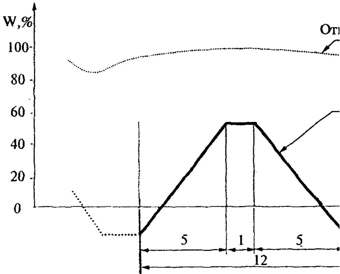
Рис. А.2. График одного цикла испытаний (первая часть испытаний по режиму IV)
