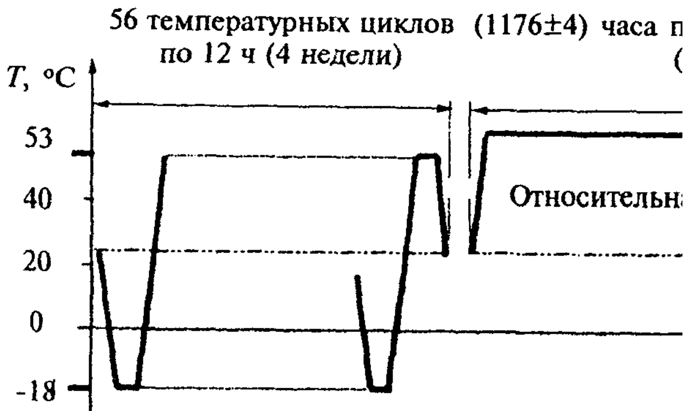
Рис. А.1. График испытаний стеклопакетов по режиму IV
