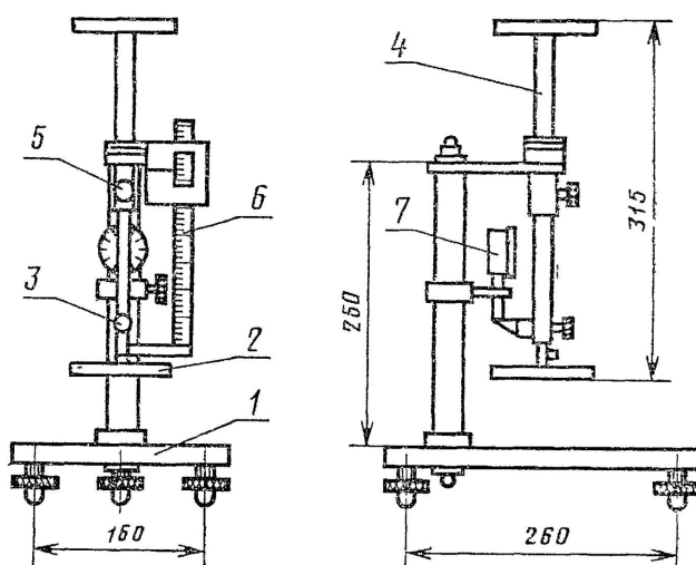
Прибор для измерения сжимаемости
