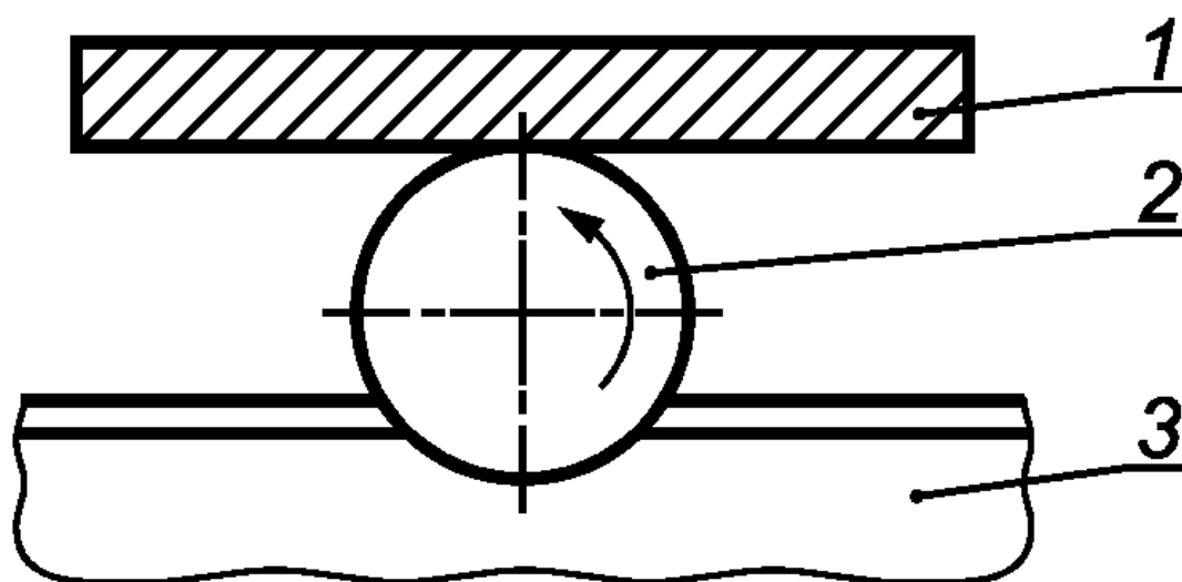
1 - образец; 2 - валик; 3 - битум
